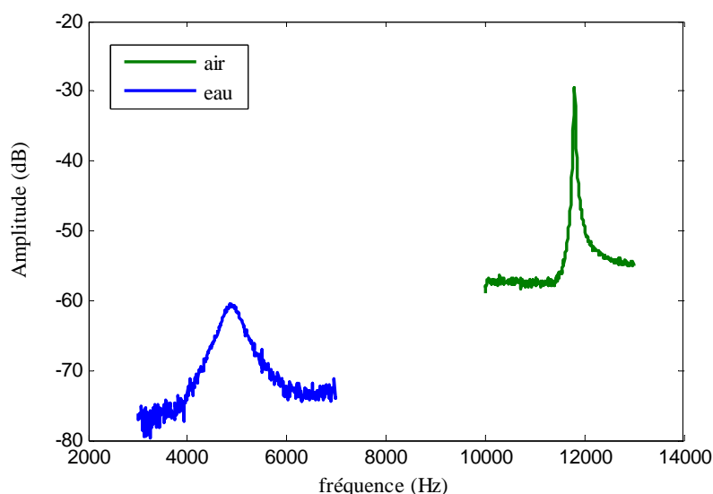
Figure 5 – Mesures électriques en dB 6 d'une micropoutre de géométrie LH dans l'air et dans l'eau déionisée à l'aide d'une détection synchrone.
