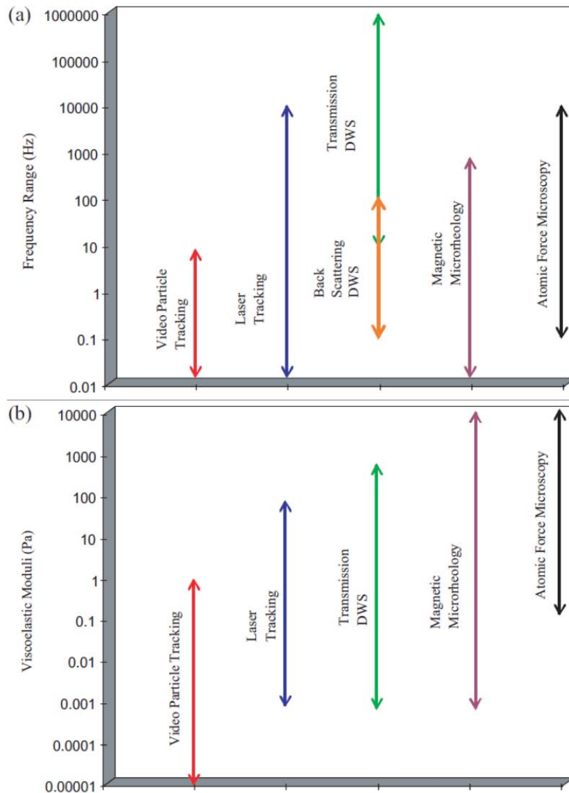
Figure 11 - Gammes typiques de fréquence (a) et de module de cisaillement (b) ; obtenues avec les différentes techniques de microrhéologie lors de la viscoélasticité linéaire de fluides complexes [WAI-05].
