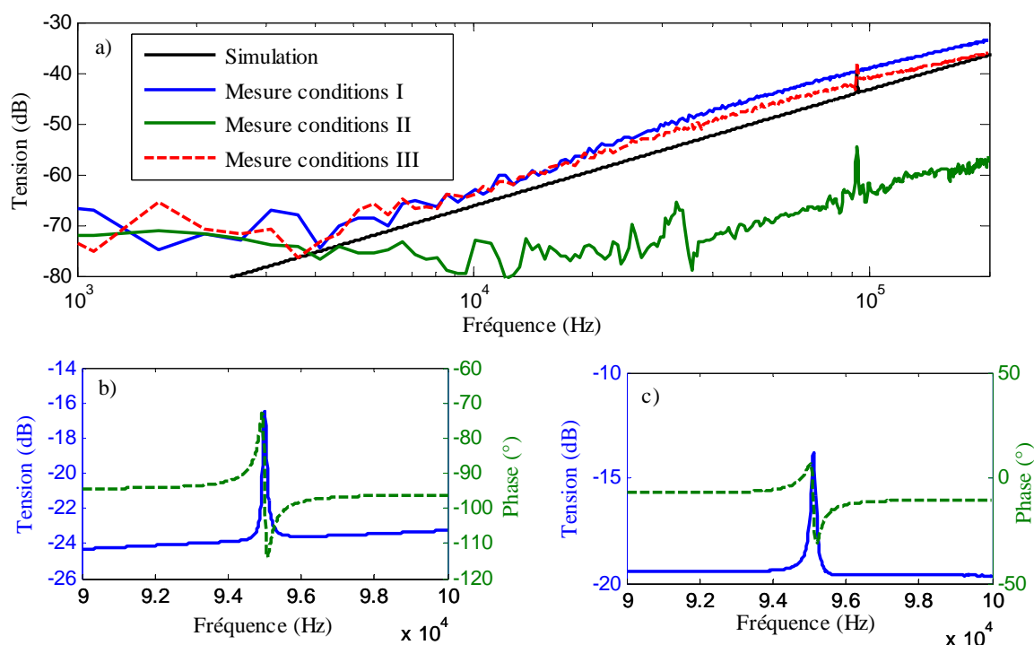
Figure 3– a) Spectres simulés et mesurés d’une poutre de type A dans l’air, illustration du couplage ; b) Simulation du pic de résonance d’une poutre A ( f_0 = 95 kHz et Q = 1000 ); c) Mesure du pic de résonance d’une poutre A altérée par le couplage.
