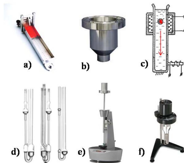
Figure 2 – a) Consistomètre de Bostwick [WEB-3], b) Coupe d'écoulement [WEB-4], c) Viscosimètre à chute de bille [WEB-5], d) Viscosimètres capillaires [WEB-6], e) Viscosimètre de Laray (à tige tombante) [WEB-7], f) Viscosimètre rotatif (Brookfield) [WEB-8].
