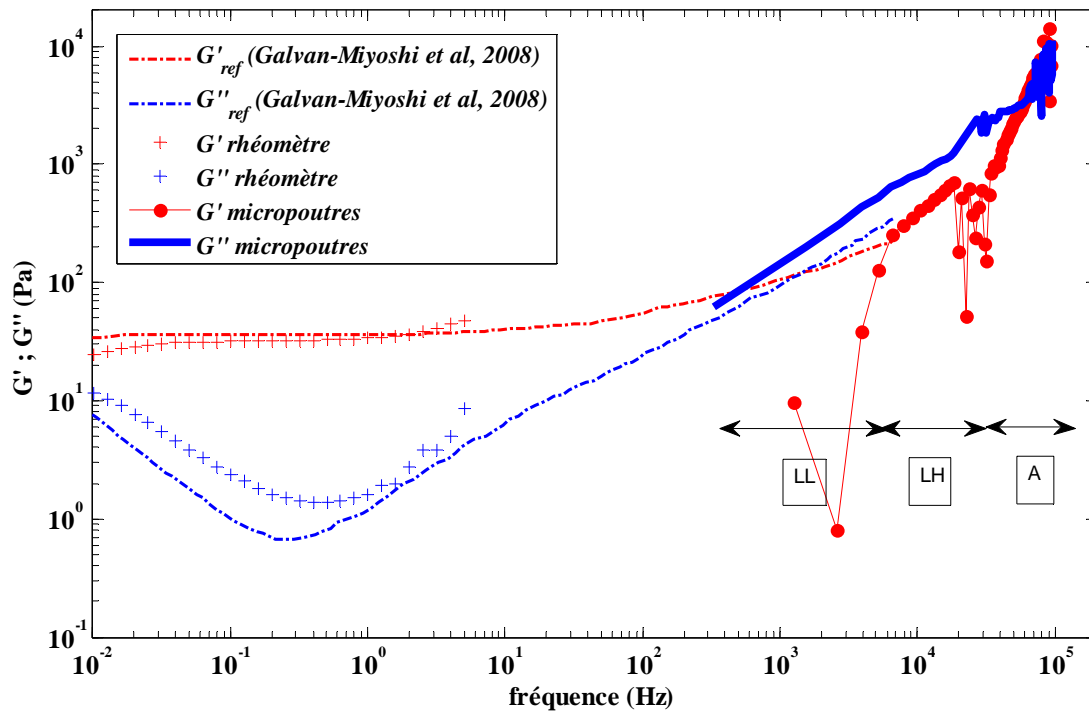
Figure 19 - G' et G'' mesurés au rhéomètre (+) puis calculés après calibration dans les trois plages de fréquence des micropoutres de type LL, LH et A (- et o), comparés avec les résultats obtenus par Galvan-Miyoshi et al. (•-) pour une mixture de CTAB identique.
