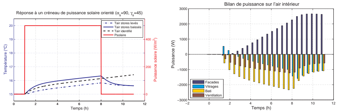
FIGURE III.17 – Réaction de l'air intérieur suite à un créneau de puissance radiative solaire
