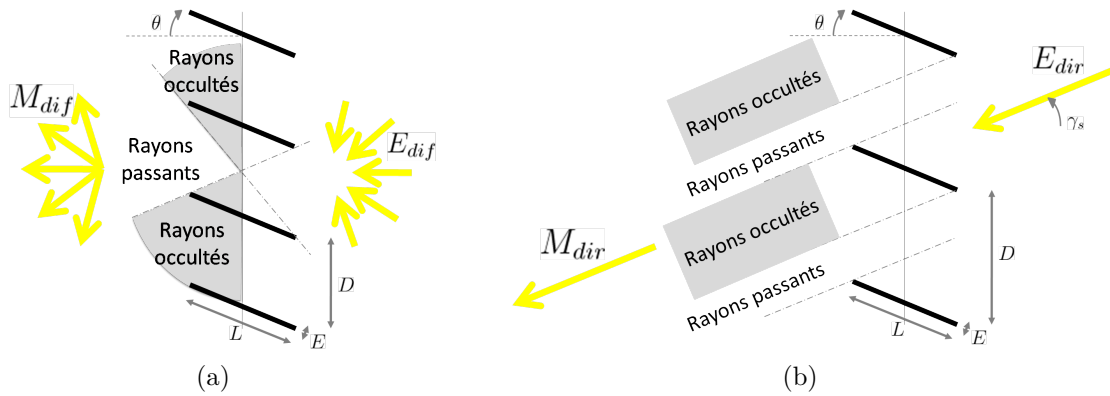
FIGURE II.7 – Indicatrices d'occultation optique du store vénitien en diffus (a) et en direct (b)
