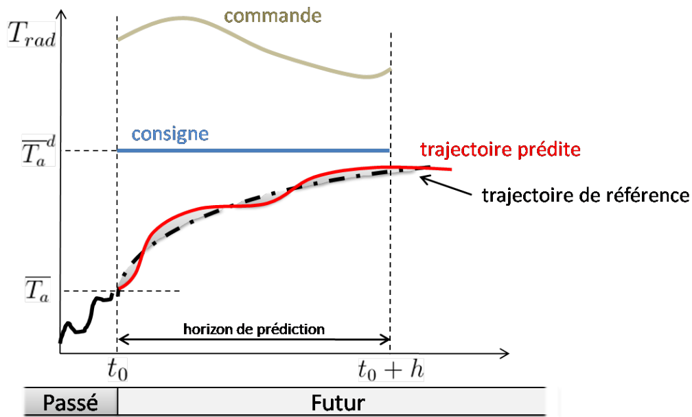
FIGURE III.22 – Modélisation du procédé et trajectoire de référence
