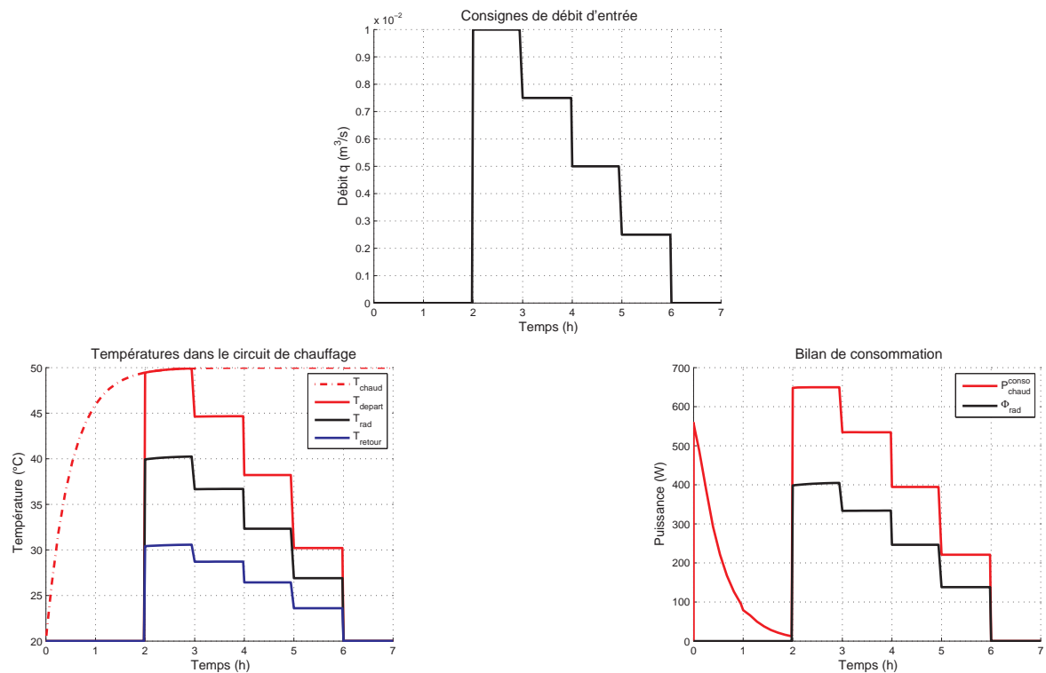
FIGURE II.6 – Températures et puissances du chauffage central
