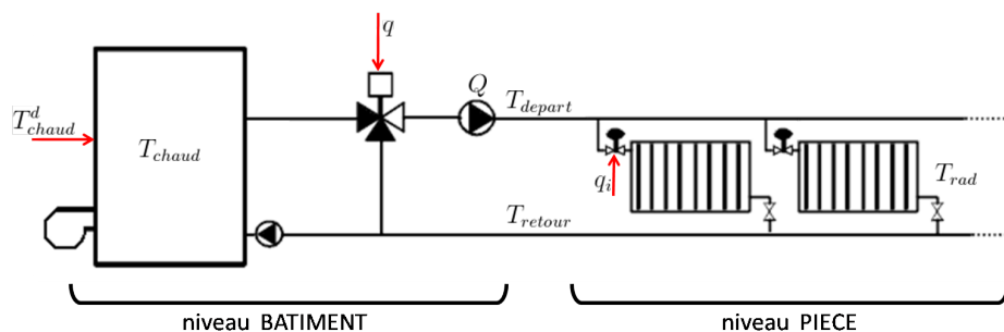
FIGURE II.5 – Principe de fonctionnement du chauffage central
