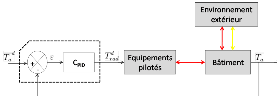
FIGURE III.11 – Schéma bloc de commande par PID du chauffage central
