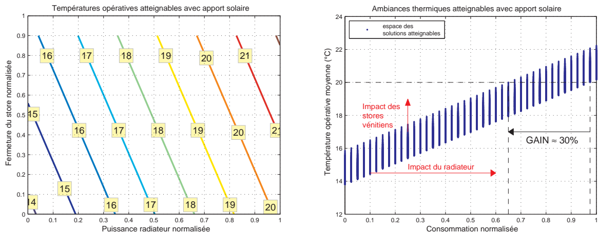
FIGURE III.27 – Espace des ambiances thermiques accessibles dans la pièce insolée
