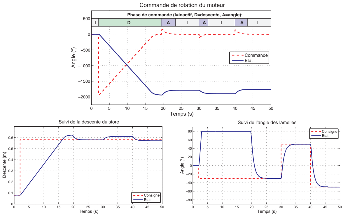
FIGURE III.6 – Suivi de position du store vénitien
