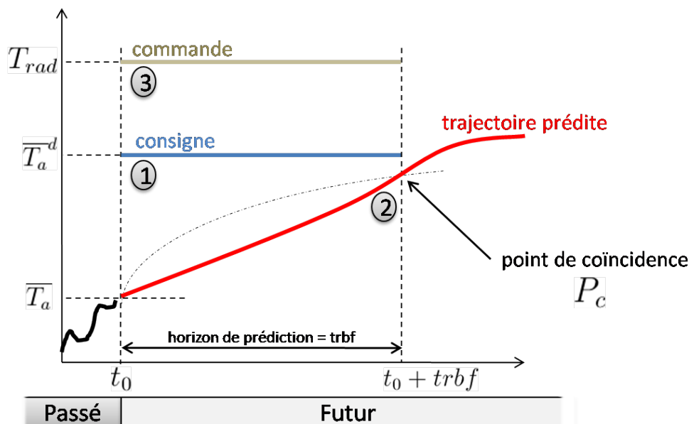
FIGURE III.19 – Modélisation du procédé et point de coïncidence
