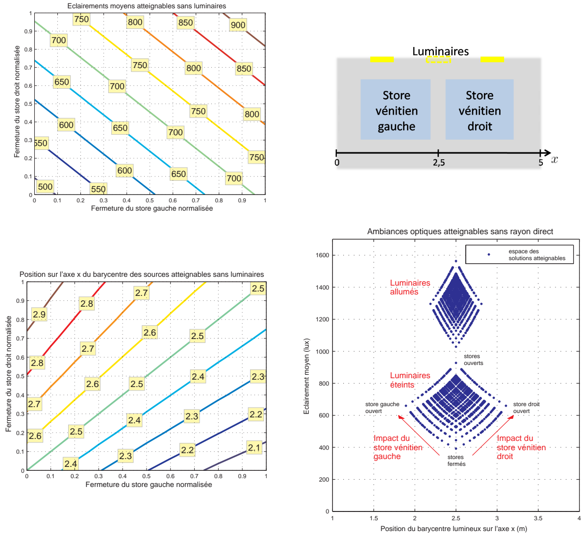
FIGURE III.28 – Représentation de l'espace des ambiances optiques accessibles
