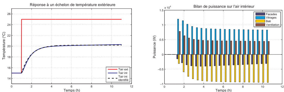
FIGURE III.14 – Réaction de l'air intérieur suite à une augmentation brutale de la température extérieure
