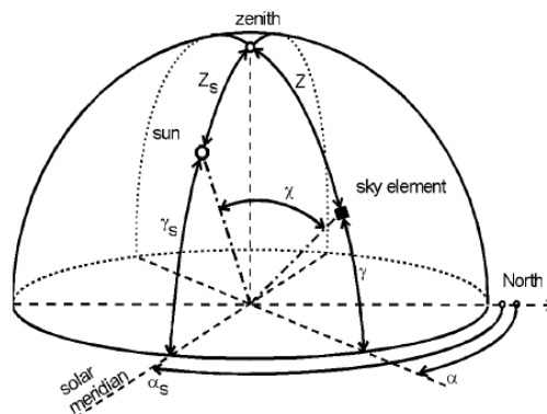
FIGURE II.3 – Référentiel angulaire de la voûte céleste
