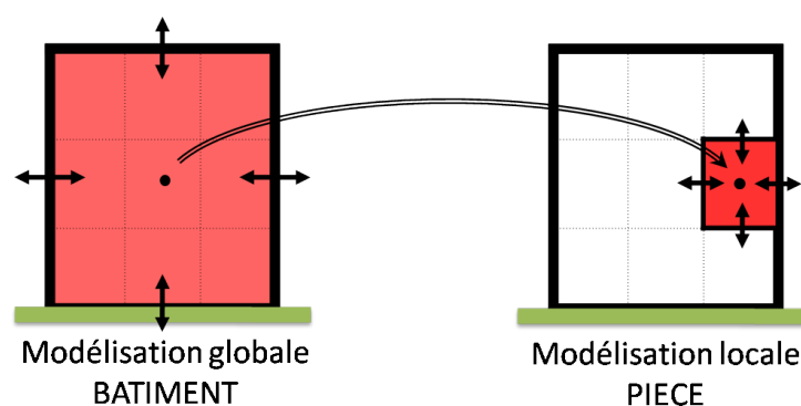
FIGURE II.12 – Principe de modélisation thermique utilisé
