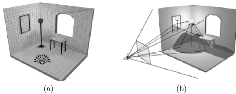
FIGURE II.1 – Principe des calculs par radiosité (a) et par lancer de rayons (b)
