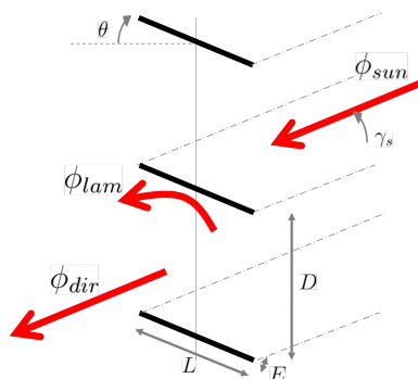
FIGURE II.10 – Modélisation thermique du store vénitien
