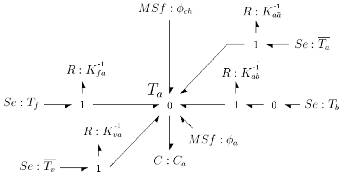
FIGURE II.22 – Représentation Bond Graph de l'air intérieur
