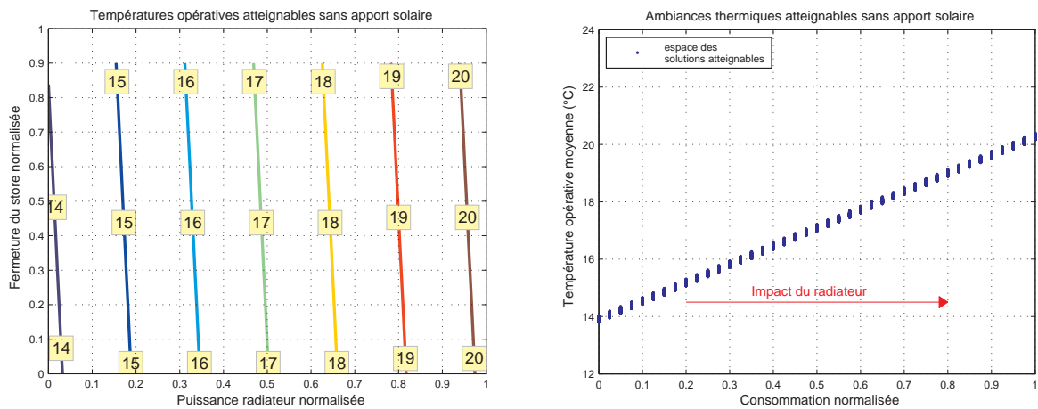
FIGURE III.26 – Espace des ambiances thermiques accessibles dans la pièce non insulée
