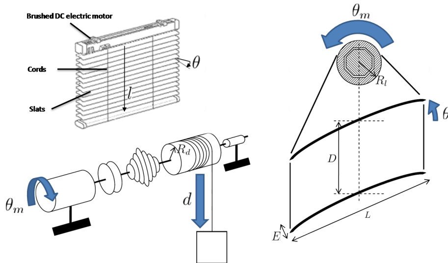
FIGURE III.4 – Schéma mécanique d'un store vénitien
