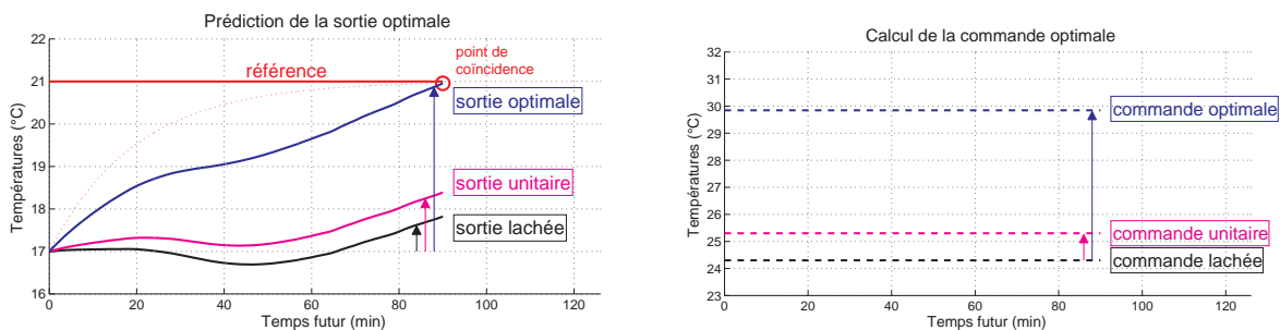
FIGURE III.21 – Exemple de calcul de la commande prédictive du chauffage central
