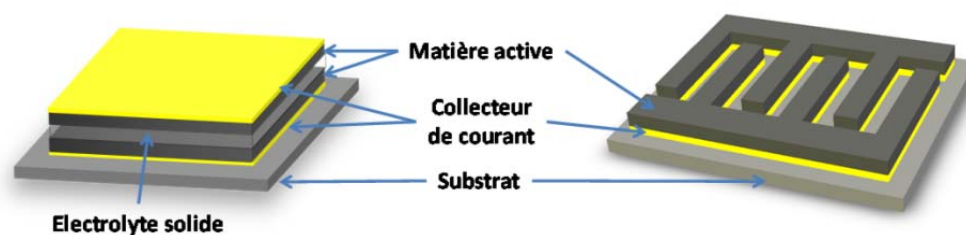
Figure III. 2. Schémas des configurations possibles pour les micro-supercondensateurs: a) empilé; b) interdigité
