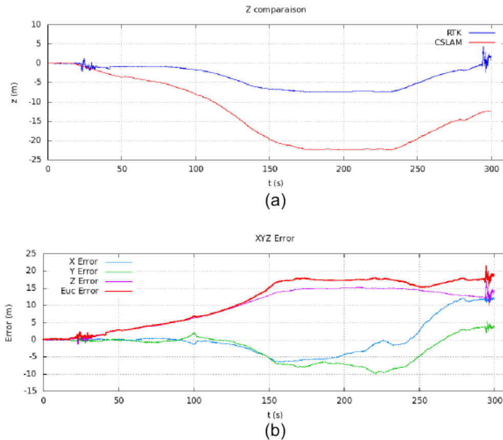
FIGURE 4.16 – Résultats du SLAM EKF monoculaire avec couplage serré d’une centrale inertielle. (a) Trajectoire en Z obtenue (rouge) et comparaison avec la vérité terrain (bleu). (b) Erreurs commises.
