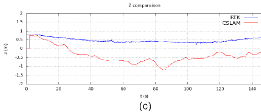
FIGURE 4.19 – Résultats du SLAM EKF monocular infrarouge avec couplage serré d'une centrale inertielle, et utilisation d'un GPS pour la correction. (a) Images de la séquence. (b) Trajectoire en XY obtenue (rouge) et comparaison avec la vérité terrain (bleu). (c) Trajectoire en Z obtenue (rouge) et comparaison avec la vérité terrain (bleu).
