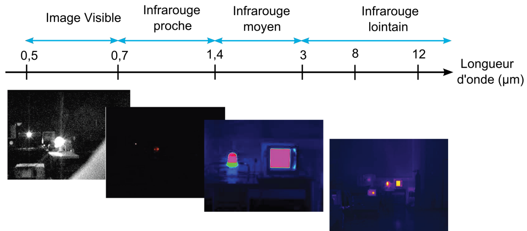
FIGURE 2.3 – Balise lumineuse marquant les bords de pistes d'un aéroport vu par différentes caméras captant le spectre visible à l'infrarouge lointain. Notons que les caméras étaient équipés d'optiques différentes.
