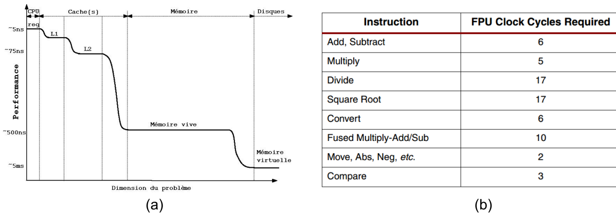
FIGURE 6.1 – A gauche, le temps d’accès aux différentes mémoires du système, comprenant un registre, deux niveaux de cache (L1 et L2), une Mémoire vive et une Mémoire virtuelle (disque dur. . .). A droite, le nombre de cycles d’horloge nécessaires à un FPU pour l’opération mathématique concernée sur des nombres simple précision.
