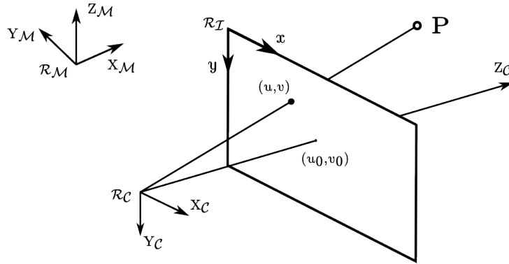
FIGURE 2.7 – Dans la représentation sténopée, un point \mathbf{P} dans le repère monde \mathcal{R}_M se projette en un point p dans le repère image \mathcal{R}_I
