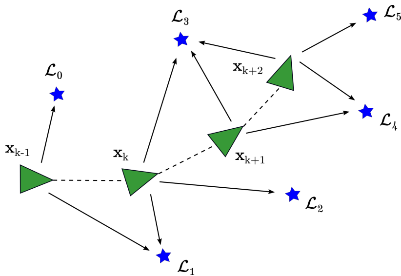
FIGURE 3.1 – Illustration du principe du SLAM. L’objectif est d’améliorer la connaissance sur la position de notre système. Pour cela, à chaque instant, il perçoit des percepts remarquables, ou amers , grâce à ses capteurs. Si ce sont des amers qu’il a déjà observés auparavant et donc qui font partie de sa carte, il effectue une réobservation de ceux-ci. Ainsi, il affine simultanément sa connaissance sur sa position et sur celle de ces amers. Si ce sont des amers qu’il observe pour la première fois, il les intègre dans sa carte dans le but de les réobserver durant les itérations suivantes.
