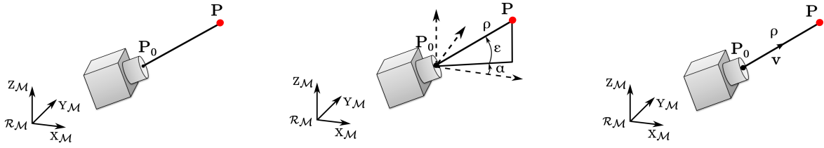
FIGURE 4.1 – Les 3 paramétrisations de points les plus courantes en SLAM visuel. A gauche, la paramétrisation euclidienne où uniquement 3 composantes sont nécessaires pour caractériser un point. Au milieu, la paramétrisation IDP , utilisant 6 composantes. A droite, la paramétrisation AHP qui fait appel à 7 composantes.
