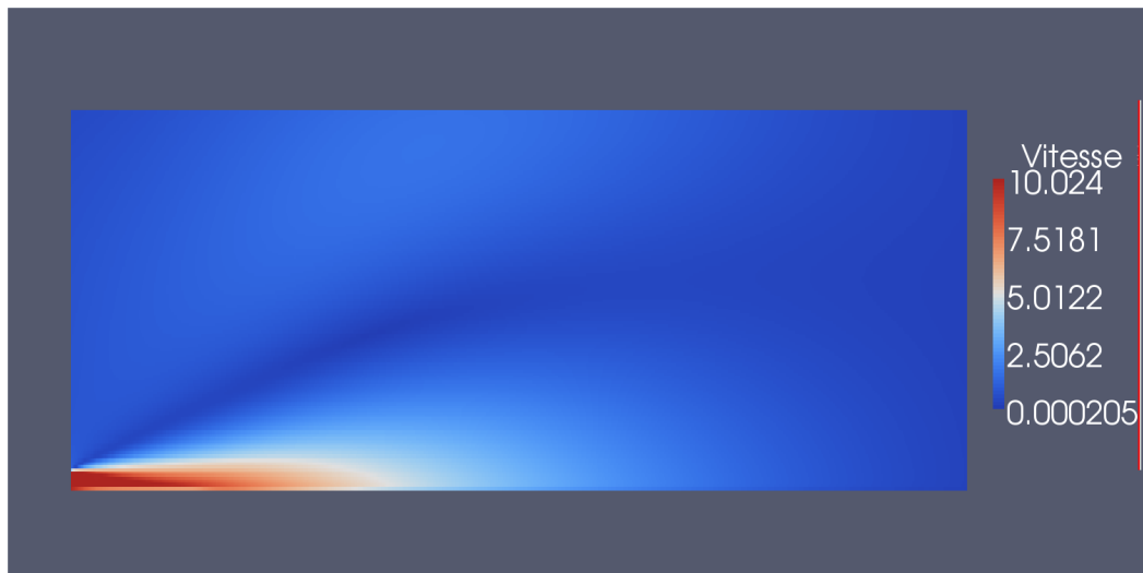
Figure 87 : Distribution de la vitesse dans la zone d'injection
