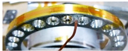
12- Ajout d'un ruban de Kapton pour maintenir l'échantillon en place et améliorer la répartition de la charge
