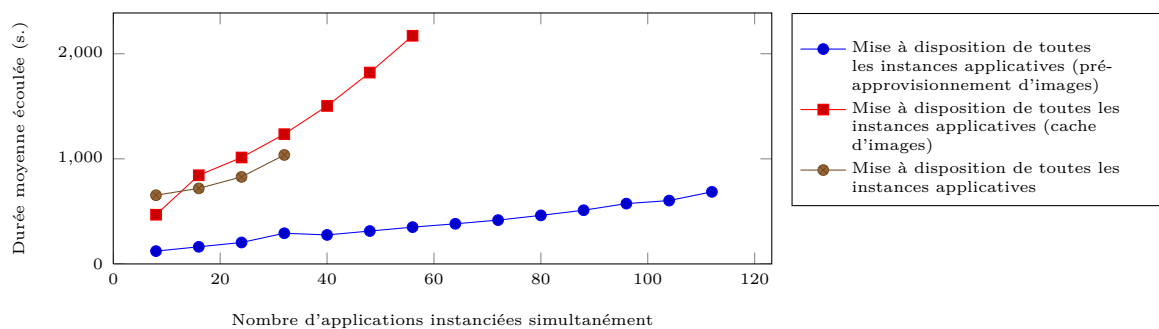
FIGURE 7.9 – Apports des mécanismes de cache d'images et de pré-appvisionnement de machines virtuelles
