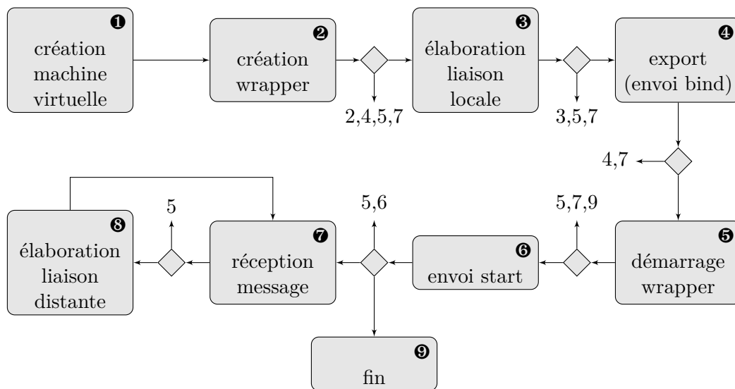
FIGURE 5.2 – Vue abstraite du flux d'exécution interne d'un configurateur
