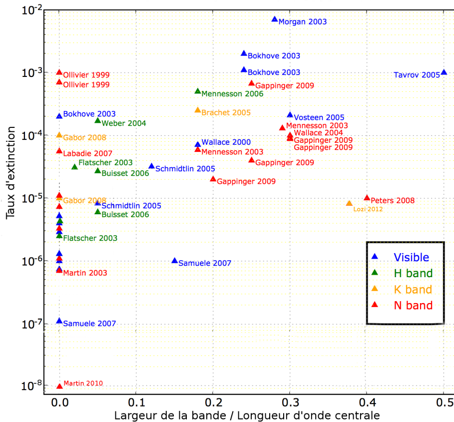
FIGURE 4.8 – État de l'art des résultats de laboratoire en termes de taux d'extinction
