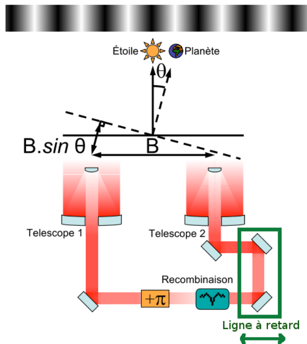
FIGURE 1.9 – Schéma de principe d'un interféromètre de Bracewell. Il est constitué de deux télescopes que l'on va cophaser à l'aide d'une ligne à retard et recombiner afin de faire interférer les deux faisceaux. Jusque-là, il s'agit d'un interféromètre à deux télescopes tout à fait classique, mais dans l'un des bras de l'interféromètre, on ajoute un déphaseur achromatique (APS) de \pi afin d'obtenir des interférences destructives et achromatiques au niveau de la ligne de visée.
