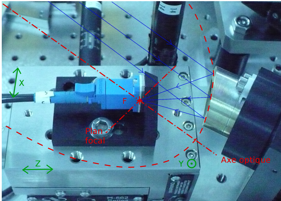
FIGURE C.14 – Mécanique d'injection dans la tête de fibre 29. Les tracés de couleur rouge représentent la parabole, son axe optique et son plan focal. Les tracés verts donnent les axes de déplacement de la platine 3 axes, sur laquelle est fixée la tête de fibre. Enfin, les rayons bleus décrivent le chemin suivi par le faisceau. On s'aperçoit que cet agencement n'est pas optimum puisque l'on aurait souhaité que l'axe X (de déplacement de la platine) soit parallèle au plan focal et que l'axe Z soit parallèle à l'axe optique de la parabole. Cette situation a pour conséquence directe de compliquer l'équilibrage des flux.
