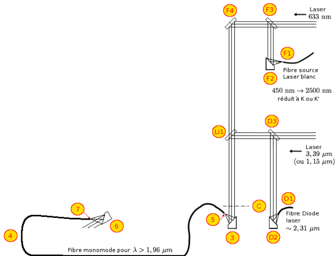
FIGURE 3.3 – Schéma optique du bloc source. Le bloc source comporte 4 sources différentes (laser 633 nm, laser blanc, laser 3,39 \mu\text{m} , diode laser dont les caractéristiques sont données tableau 3.1 ) qui empruntent, comme on peut le voir, 4 chemins différents. Cependant, toutes les sources finissent par traverser le chopper C et atteindre la parabole 3 pour être injectées dans la fibre 4 qui va uniformiser les caractéristiques des faisceaux. Sur ce schéma, les ronds jaunes cerclés de rouge donne les références des différentes optiques. Les traits gras noir indiquent des fibres optiques, les rectangles indiquent des miroirs plans, les trapèzes indiquent des miroirs paraboliques et enfin les 3 traits fins parallèles indique la propagation des faisceaux.
