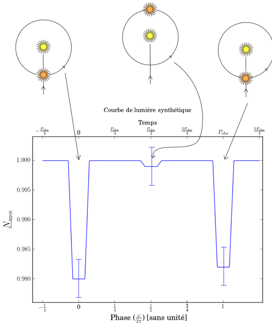
FIGURE 7.6 – Courbe de lumière simplifiée dans le cas d’un modèle basé sur un système éclipseur {étoile+ étoile} pour lequel P = P_{\text{obs}} : Dans ce cas, la période orbitale correspond bien à la période mesurée, car la profondeur du transit secondaire est plus faible que celle du transit primaire. Les profondeurs \frac{\Delta F}{F}|_0 , \frac{\Delta F}{F}|_1 et \frac{\Delta F}{F}|_{1/2} sont bien des mesures du transit primaire, du transit primaire impair, et du transit secondaire respectivement.
