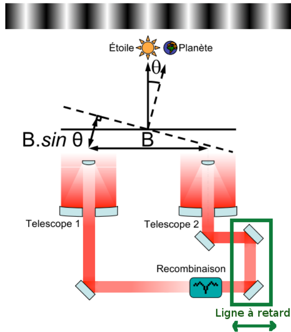
FIGURE 1.6 – Schéma simplifié d'un interféromètre classique à deux télescopes : On retrouve les éléments principaux d'un interféromètre : les télescopes, bien sûr, mais aussi la ligne à retard (LAR) et la recombinaison. En sortie de recombinaison, on vient mesurer l'évolution de l'intensité lumineuse résultant de l'interférence entre les deux faisceaux de l'interféromètre en fonction de la position de la LAR et l'évolution. C'est ce que l'on appelle le paquet de franges. Chaque source ponctuelle observée produit un paquet de franges sinusoïdal (si la source est monochromatique). Si l'on observe plusieurs sources ponctuelles en même temps, et sous l'hypothèse qu'elles soient incohérentes entre elles, le paquet de franges observé est donné par la somme des paquets de franges produits par chacune des sources ponctuelles. C'est l'étude de ce paquet de franges qui va nous permettre de retrouver l'information sur la distribution spatiale des sources observées.
