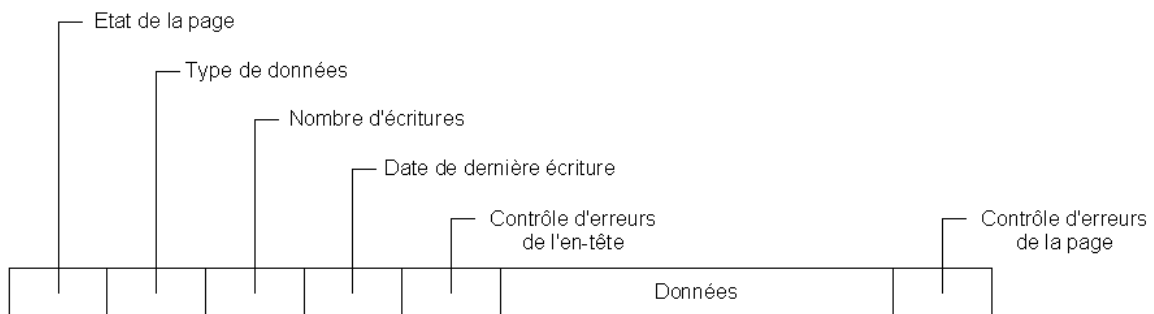
Figure 3.7 – Exemple d'attributs de l'en-tête d'une page
