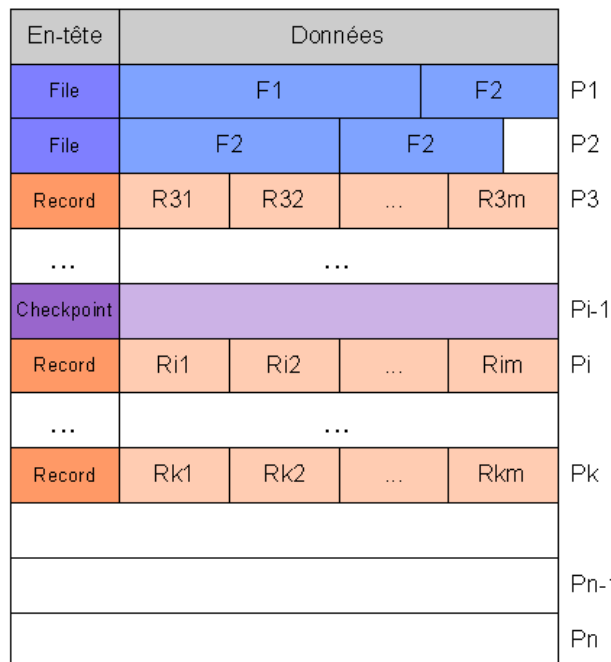
Figure 3.9 – Organisation générale de la mémoire Flash gérée par le système LiveFile
