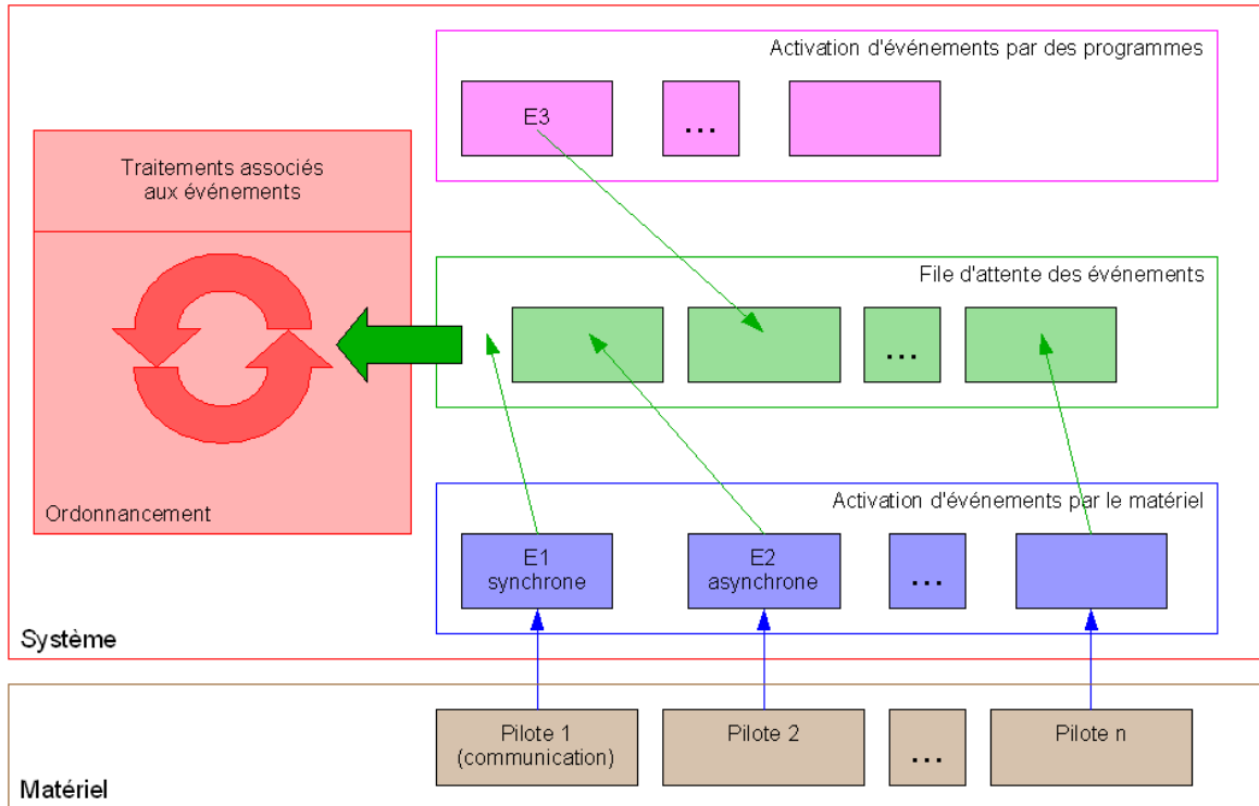
Figure 2.18 – Gestion des événements dans le système Contiki
