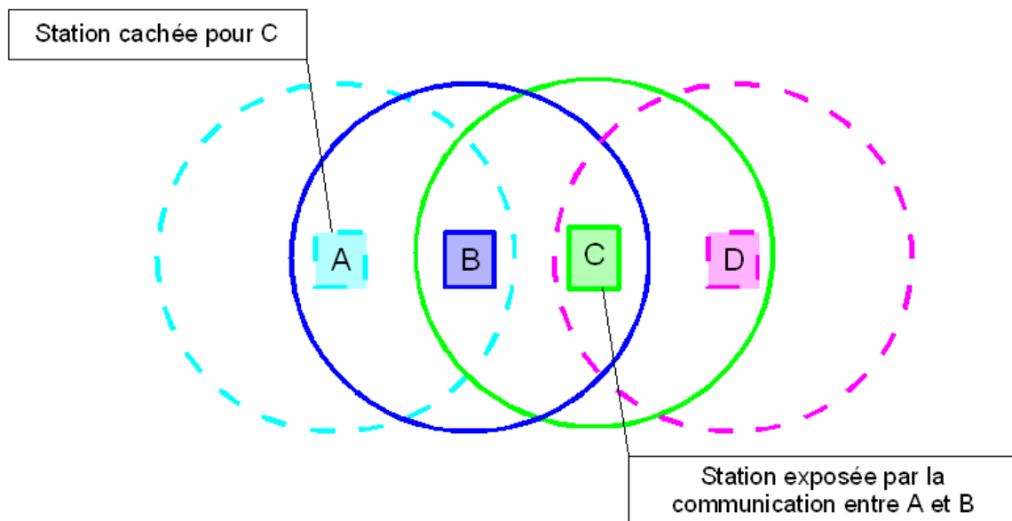
Figure 1.13 – Illustration des problèmes de station cachée ou exposée
