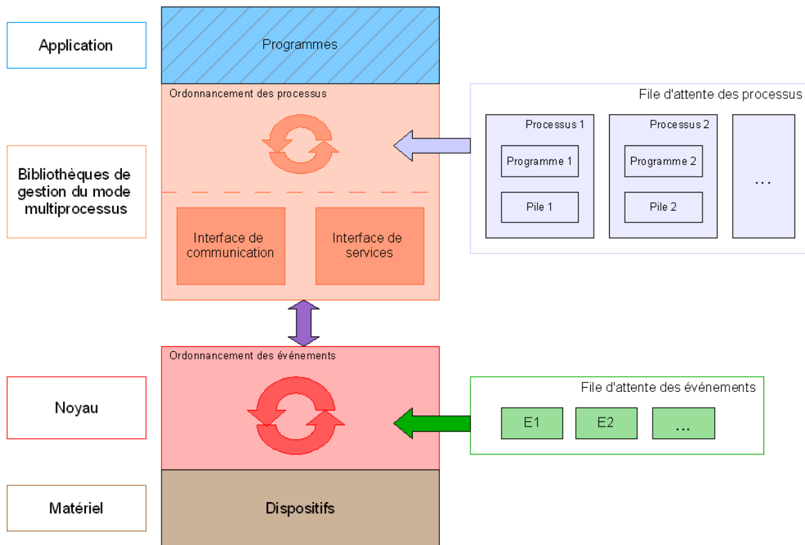
Figure 2.19 – Principe de fonctionnement du système Contiki en mode multitâche
