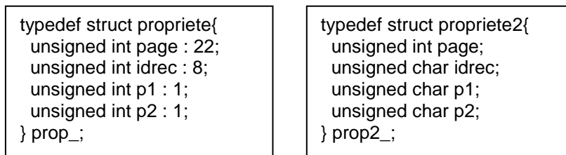
Figure 4.18 – Différentes solutions pour le stockage des propriétés
