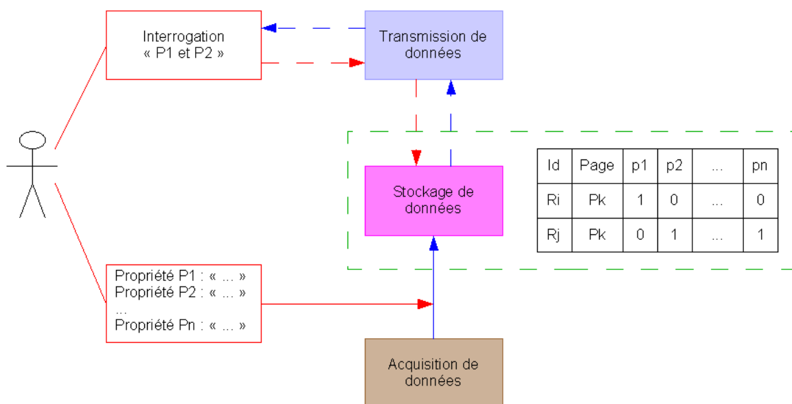
Figure 3.33 – Gestion des propriétés des données collectées
