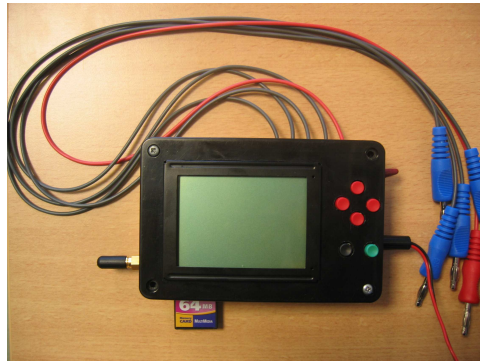
Figure 4.1 – Capteur biomédical du projet STAR
