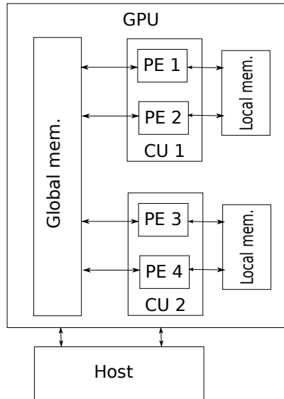
FIGURE 7.1 – Illustration d'un GPU. – l'accès à la mémoire locale est nettement plus rapide que l'accès à la mémoire globale.
