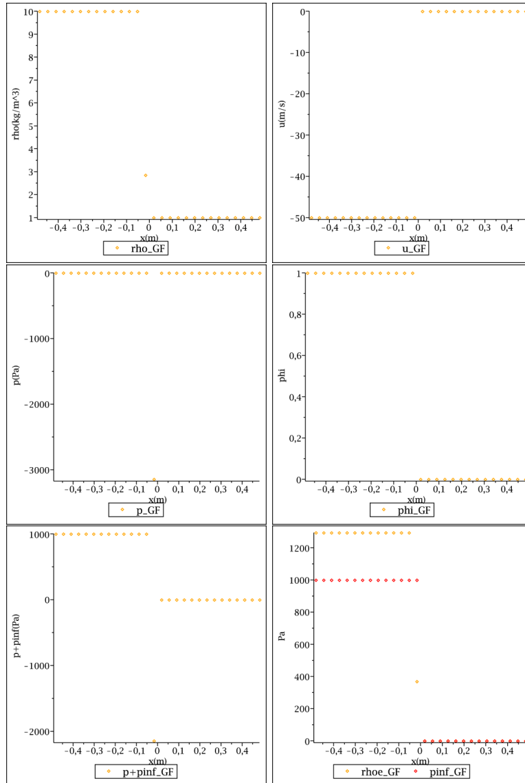
FIGURE 2.8 – Tracés de la masse volumique \rho , de la vitesse u , de la pression p , de la fraction de gaz \varphi , de la variable p + p_\infty et de la variable \rho\varphi que nous comparons à p_\infty après une itération dans le cas du problème de Riemann référencé dans le Tableau 2.2. Nous illustrons les problèmes de robustesse du schéma « Single Fluid », en effet après une itération le schéma « Single Fluid » nous fournit un état en dehors du domaine d’hyperbolicité \Omega car p + p_\infty < 0 ou de manière équivalente \rho\varphi < p_\infty .
