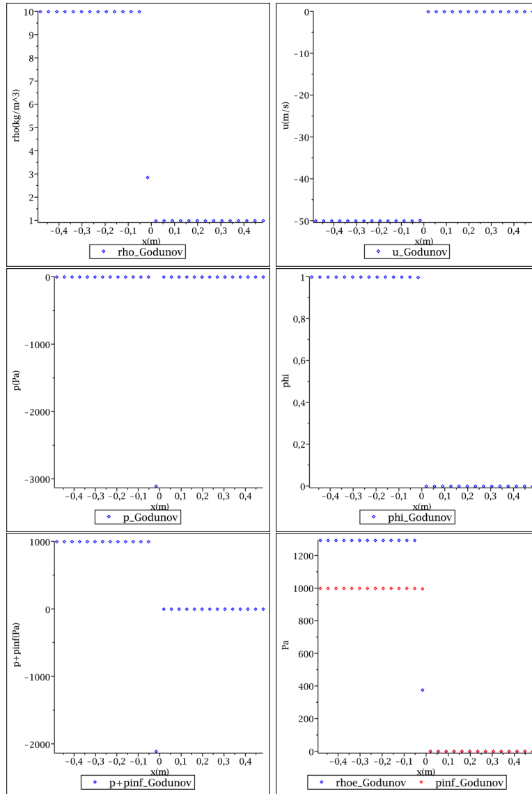
FIGURE 2.6 – Tracés de la masse volumique \rho , de la vitesse u , de la pression p , de la fraction de gaz \varphi , de la variable p + p_\infty et de la variable \rho e que nous comparons à p_\infty après une itération dans le cas du problème de Riemann référencé dans le Tableau 2.2. Nous illustrons les problèmes de robustesse du schéma de Godunov, en effet après une itération le schéma de Godunov nous fournit un état en dehors du domaine d’hyperbolicité \Omega , car p + p_\infty < 0 ou de manière équivalente \rho e < p_\infty .
