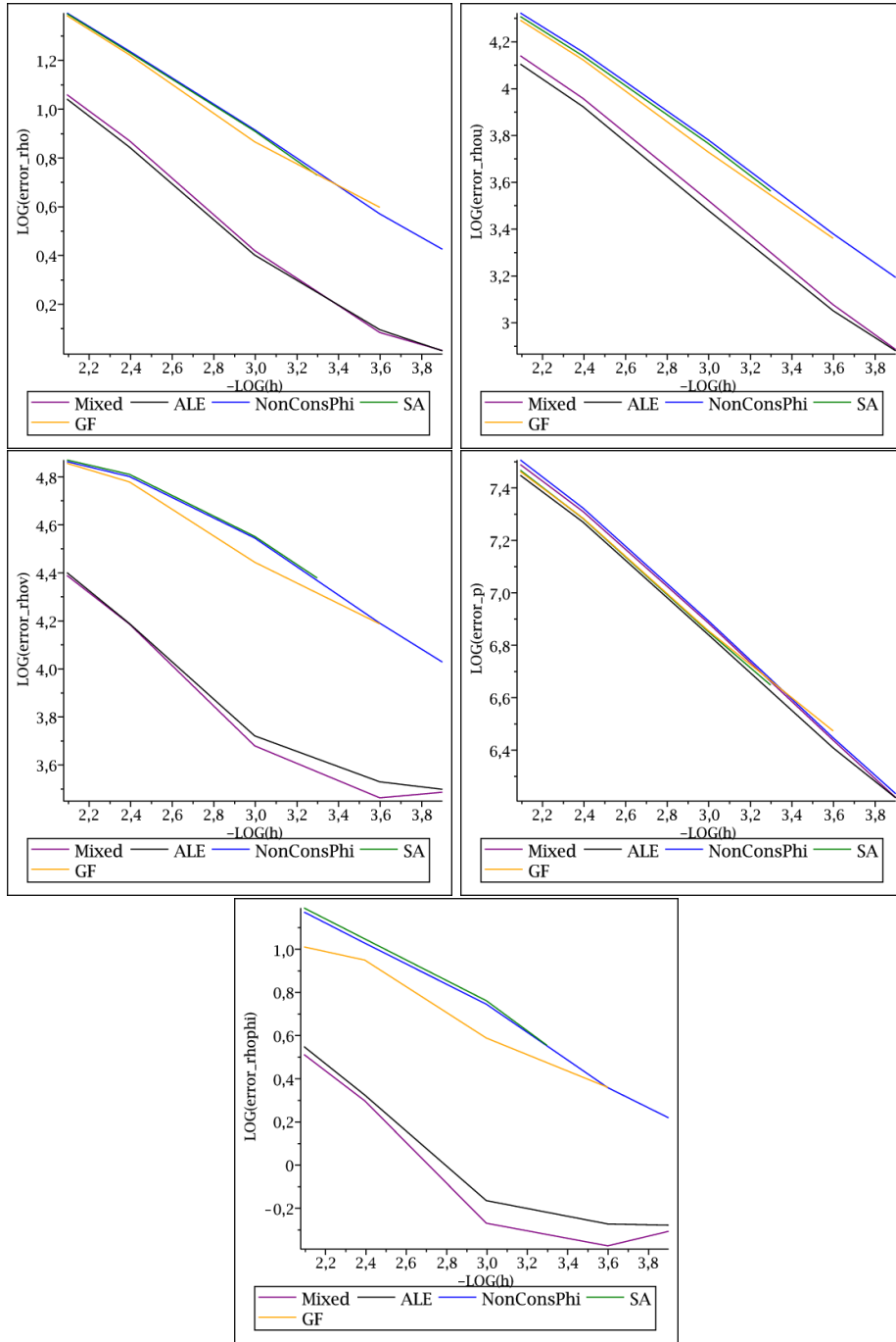
FIGURE 5.10 – Erreurs en norme L^1 sur la masse volumique \rho , les quantités de mouvement \rho u et \rho v , la pression p et la masse volumique de gaz \rho\phi au temps final t_1 = 240 \mu s pour le cas d'un tube à choc avec une forte discontinuité sur la vitesse transversale v (voir Tableau 5.4). Le taux de convergence est approximativement le même pour les différents algorithmes et les différents algorithmes fournissent la même erreur sur la pression p . Nous constatons cependant que les deux algorithmes « Mixed » et « ALE » faisant intervenir la projection mixte \Pi_{\omega}^{\text{mxt}} améliorent la résolution de l'interface \varphi et approchent donc mieux la solution exacte sur la masse volumique \rho et les quantités de mouvement \rho u et \rho v que les algorithmes « SA », « GF » et « NonConsPhi ». Les « cassures » dans les graphes obtenus avec les algorithmes « Mixed » et « ALE » sont liées à la projection aléatoire.
