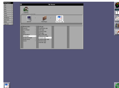
(d) 1985 NeXTSTEP (OpenStep here)
