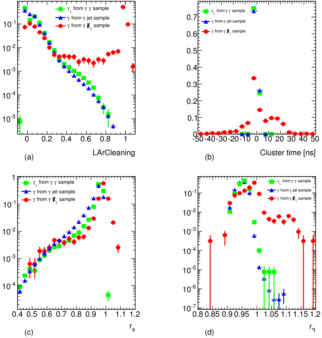
FIGURE 6.10 – Distributions des variables discriminantes pour les photons de l'échantillon \gamma\gamma (carrés verts), de l'échantillon \gamma + \text{jet} (les triangles bleus) et de l'échantillon \gamma + \cancel{E}_T (points rouges).
