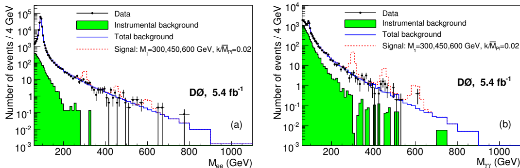
FIGURE 2.18 – Spectres en masse invariante des événements diélectron et diphoton obtenus par la collaboration D\bar{O} dans le contexte de la publication [72].
