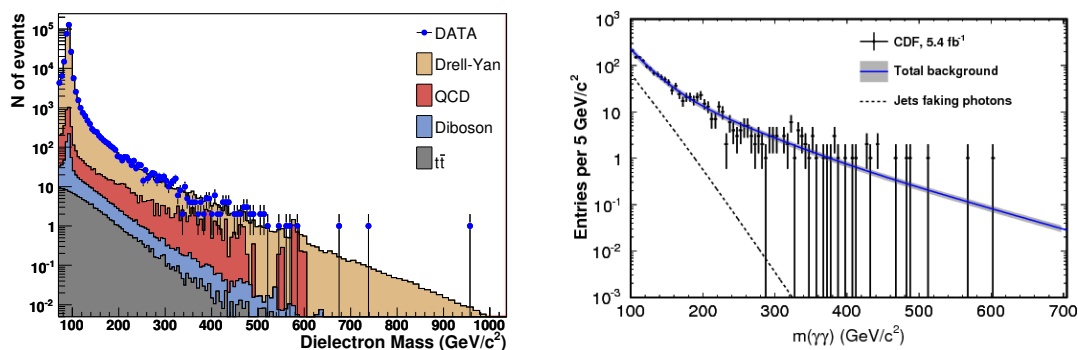
FIGURE 2.17 – Spectres en masse invariante des événements diélectron et diphoton obtenus par la collaboration CDF dans le contexte des publications [70] et [69].
