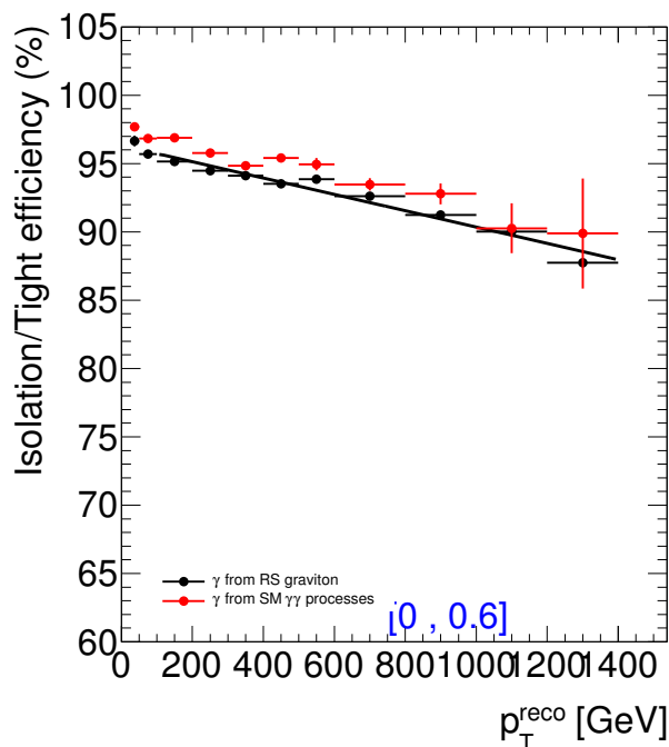
FIGURE 5.20 – Efficacité de la coupure d'isolation en fonction de l'impulsion transverse ( p_T^{\text{reco}} sur la figure) du photon pour des photons avec |\eta| \in [0, 0.6] . Les points rouges représentent la simulation de photons de processus diphoton du Modèle Standard alors que les points noirs représentent des photons de processus gravitons de RS. Un ajustement linéaire est superposé à la prédiction du modèle RS.
