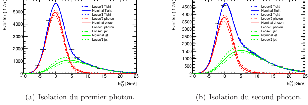
FIGURE 7.12 – Impact de la variation de la définition de loose' sur les distributions des faux candidats et des vrais photons.
