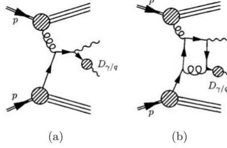
FIGURE 3.4 – Exemples de diagrammes de Feynman illustrant la production de deux photons dont un photon de fragmentation.
