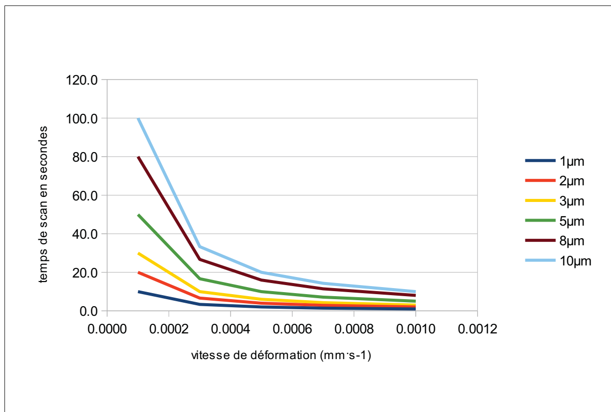
Figure 1.7 : Temps de scan en fonction de la vitesse de déformation pour plusieurs valeurs de la résolution
