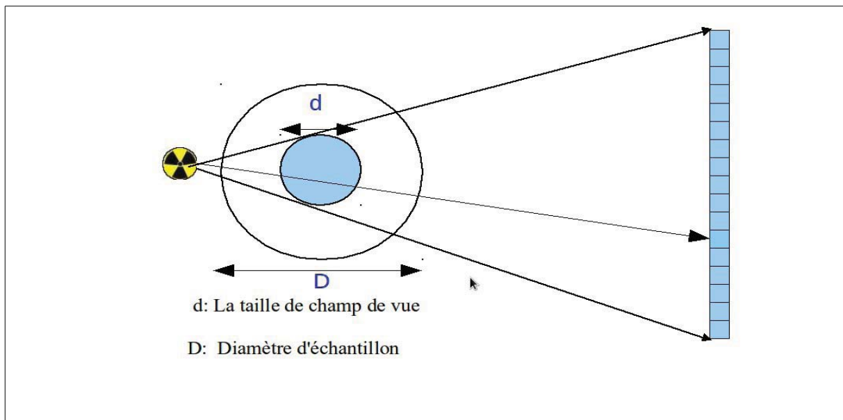
Figure 3.11 : Relation entre la taille du champ de vue et le diamètre de l'échantillon
