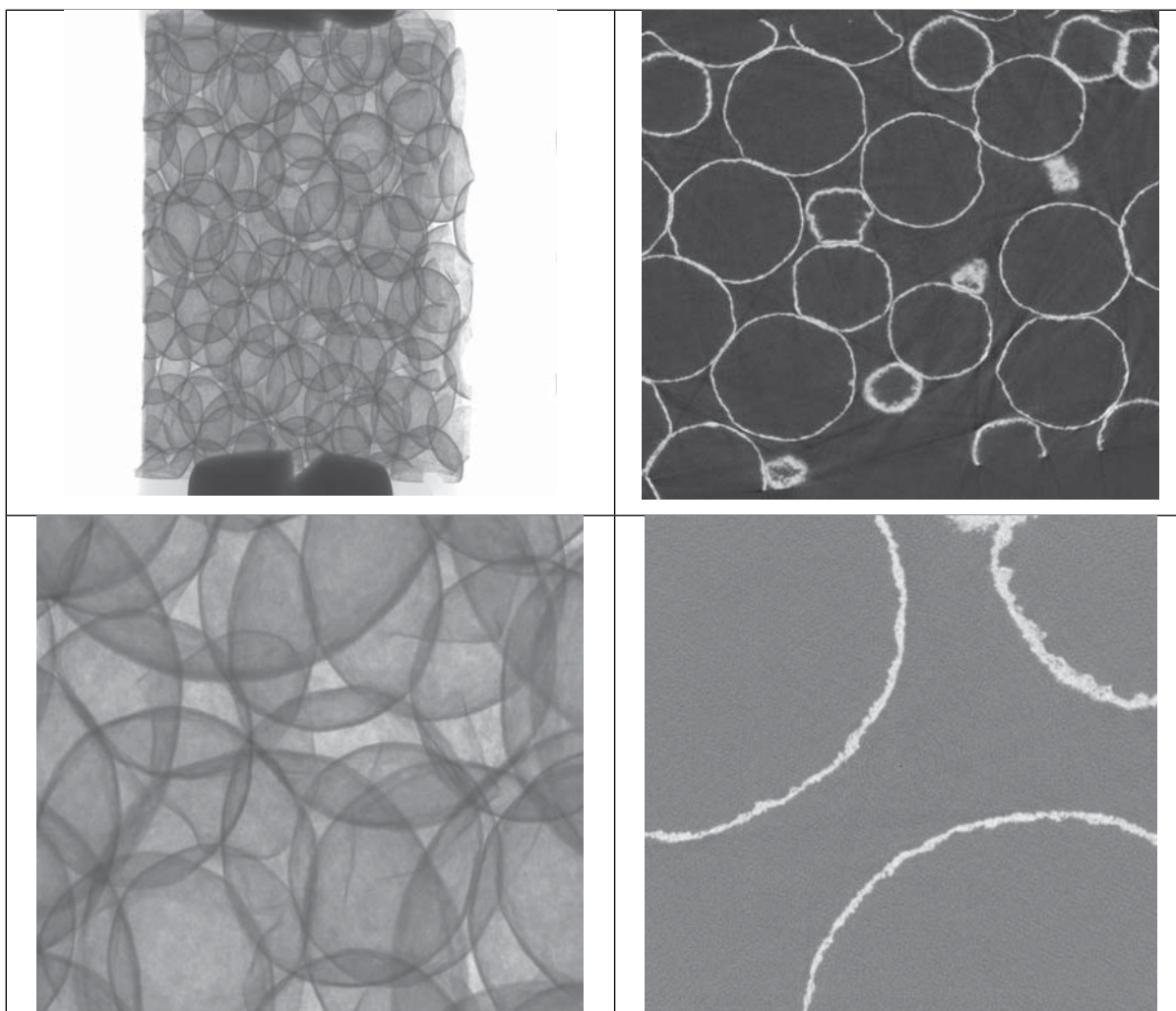
Figure 2.7a : Projection basse et haute résolution de l'empilement de sphères creuses
