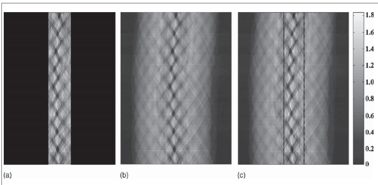
Figure 1.26 : Sinogramme de fantôme 'sea-urchin'. (a) Sinogramme en haute résolution(la tomographie locale). (b) Sinogramme en basse résolution. (C) Sinogramme combiné par (a) et (b) [xiao 2007]
