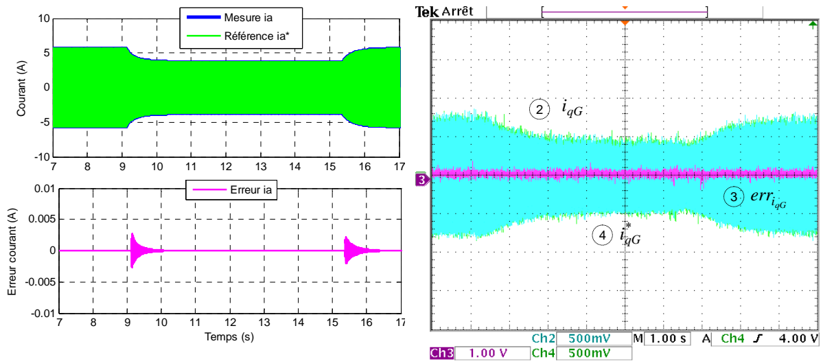
Figure 5.18. Réponse temporelle face à une variation de la vitesse d'eau en simulation à gauche et en expérimental à droite : courant i_{qG} et i_{qG}^* 2.5A/div (le même zéro), err_{i_{qG}} 2.5A/div
