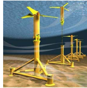
Figure 1.23. Le système d'émergence des turbines ©[TGL-09]
