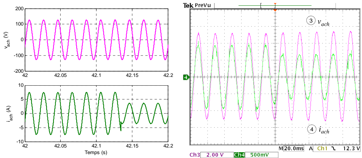
Figure 5.75. Zoom sur l'instant de la diminution de la charge, en simulation à gauche et en expérimental à droite : i_{ach} : 2.5A/div , v_{ach} 50V/div
