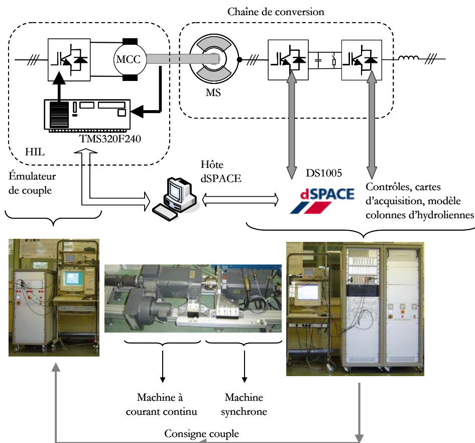
Figure 4.3. Correspondance avec les éléments physiques pour le générateur hydrolien interfacé en aval de la connexion
