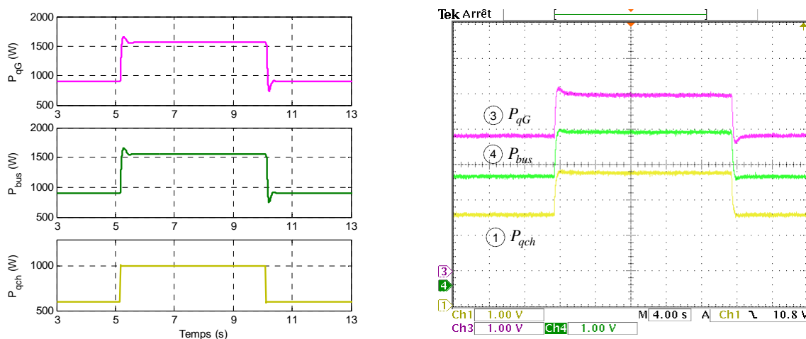
Figure A5.18. Bilan équilibre production – consommation P_{qG} , P_{bus} , P_{qch} : 500W/div
