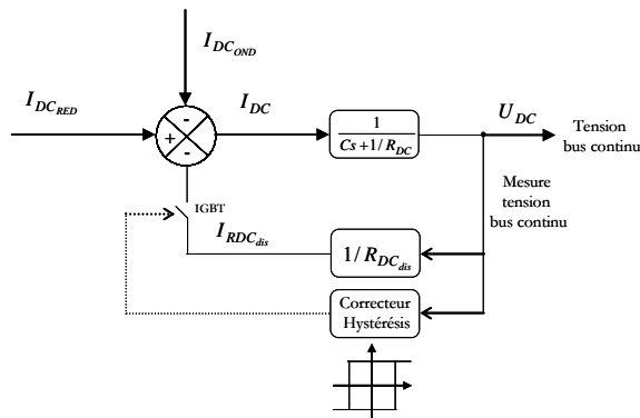
Figure 5.54. La structure de commande avec le correcteur analogique à hystérésis
