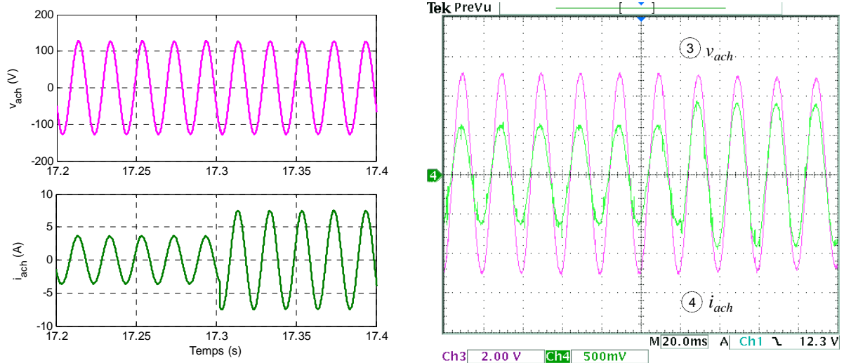
Figure 5.74. Zoom sur l'instant de l'augmentation de la charge, en simulation à gauche et en expérimental à droite : i_{ach} : 2.5A/div , v_{ach} 50V/div
