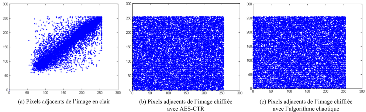
Figure IV.4 : La corrélation entre les pixels adjacents de l'image de Lenna en clair et chiffrée avec AES-CTR et l'algorithme du chaos.
