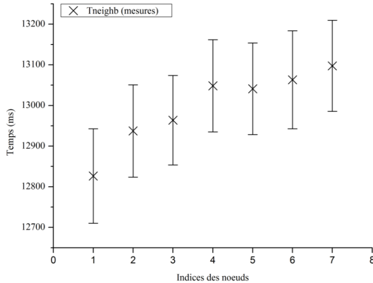
Figure IV.15 : Temps d'établissement d'un lien sécurisé d'un nœud N_i avec son nouveau voisin N_{i+1} .
