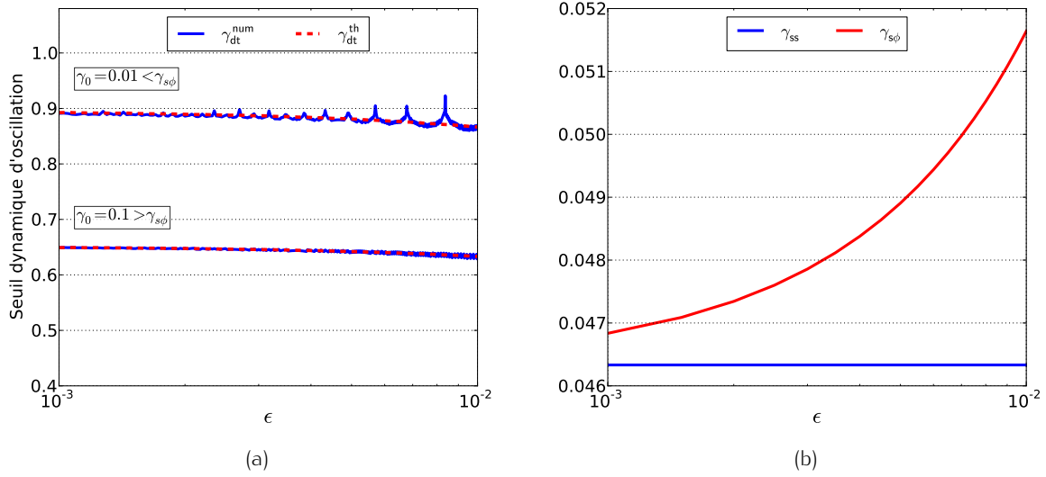
FIGURE C.2 – (a) Seuil dynamique \gamma_{dt}^{num} calculé sur la simulation du système (2.23) comparé à la prédiction théorique \gamma_{dt}^{num} obtenu par la résolution de l'équation (2.36) pour \gamma_0 = 0.01 < \gamma_{s\phi} (courbes du haut) et \gamma_0 = 0.1 > \gamma_{s\phi} (courbe du bas). (b) Point \gamma_{s\phi} et point superstable \gamma_{ss} en fonction de \epsilon . \zeta = 0.5 et la précision utilisée est de 200 chiffres significatifs.
