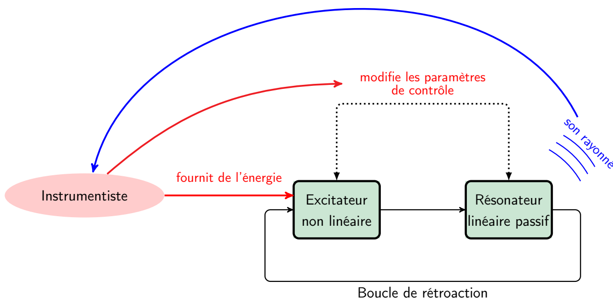
FIGURE 1.1 – Schéma général d'instrument de musique auto-oscillant, modélisé par un élément non linéaire actif couplé avec un élément linéaire passif. L'instrumentiste fournit l'énergie au système puis modifie les paramètres de contrôle (pression dans la bouche et embouchure) en fonction de son jugement sur le son rayonné.
