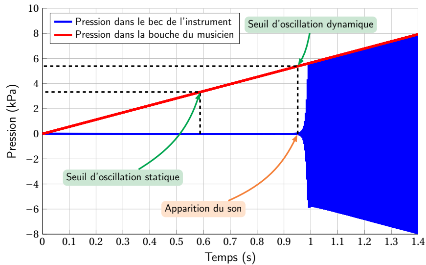
Figure 1.2 – Simulation du modèle de clarinette dit "de Raman" (cf. section 1.2.4) où la pression dans la bouche du musicien augmente linéairement dans le temps. L'apparition du son apparaît à une valeur de pression dans la bouche, seuil d'oscillation dynamique , supérieur au seuil d'oscillation statique théorique [59].
