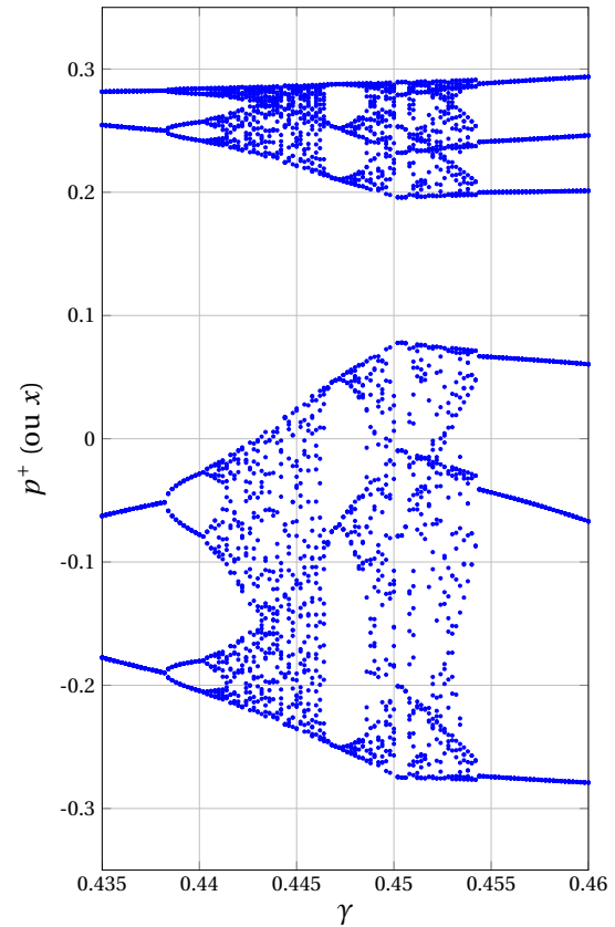
Figure 1.7 – Diagramme de bifurcation statique de modèle du clarinette de Raman (équation (1.33)) pour \lambda = 0.95 et \zeta = 0.8 . Digramme correspondant à la variable p^+ (ou x ) tracé entre \gamma = 0.435 et \gamma = 0.46 . Le diagramme est obtenu en simulant 1000 itérations de l'équation (1.33) puis en prenant les 40 dernières valeurs des orbites obtenues.
