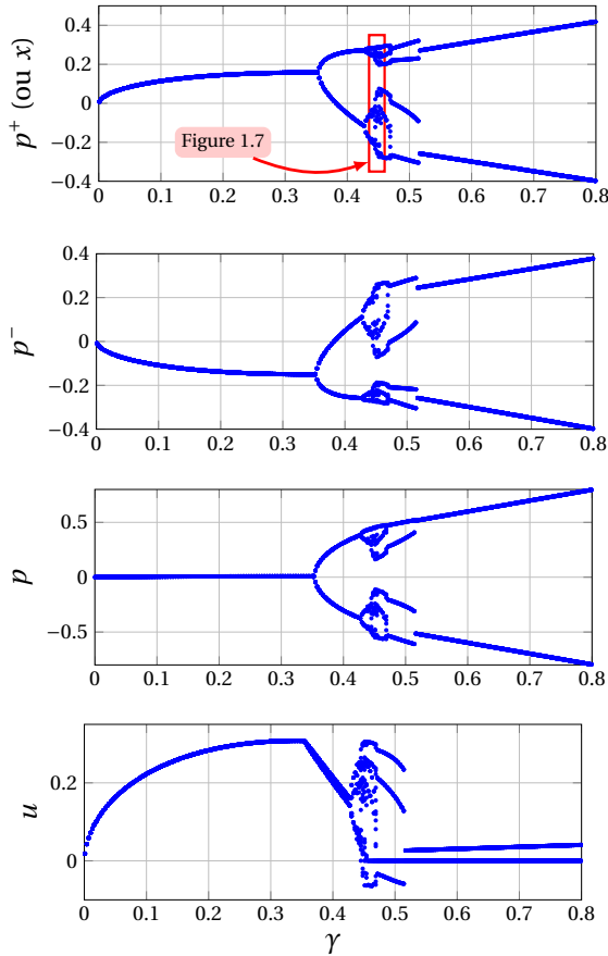
Figure 1.6 – Diagrammes de bifurcation statiques du modèle du clarinette de Raman (équation (1.33)) pour \lambda = 0.95 et \zeta = 0.8 . De haut en bas : digramme en p^+ (ou x ), p^- , p et u . Ces digrammes sont obtenus en simulant 400 itérations de l'équation (1.33) puis en prenant les 20 dernières valeurs des orbites obtenues. Cette méthode est tirée de [84] où elle est aussi vérifiée.
