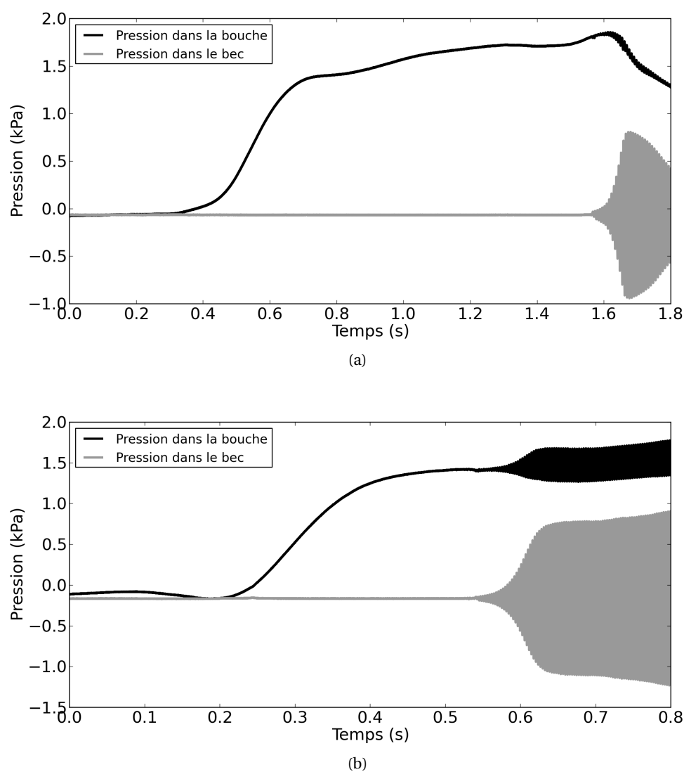
Figure 5.2 – Mesure in vivo de l'attaque d'une note de clarinette. Pression dans la bouche de l'instrumentiste (en noir) et pression dans le bec de l'instrument (en gris). (a) Première attaque d'une gamme détachée effectuée en pianissimo . (b) Attaque lors d'un exercice d'échauffement spontané, sans consigne précise.
