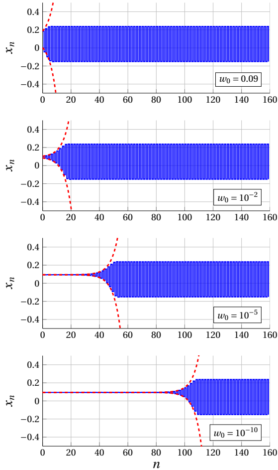
Figure 1.10 – (—) Évolution temporelle de la variable x , solution de (1.33), pour différentes valeurs de w_0 . De haut en bas : w_0 \approx 0.09 , w_0 = 10^{-2} , w_0 = 10^{-5} and w_0 = 10^{-10} . (---) Enveloppe théorique déduite de la fonction (1.53). \gamma = 0.42 , \zeta = 0.5 et \lambda = 1 .
