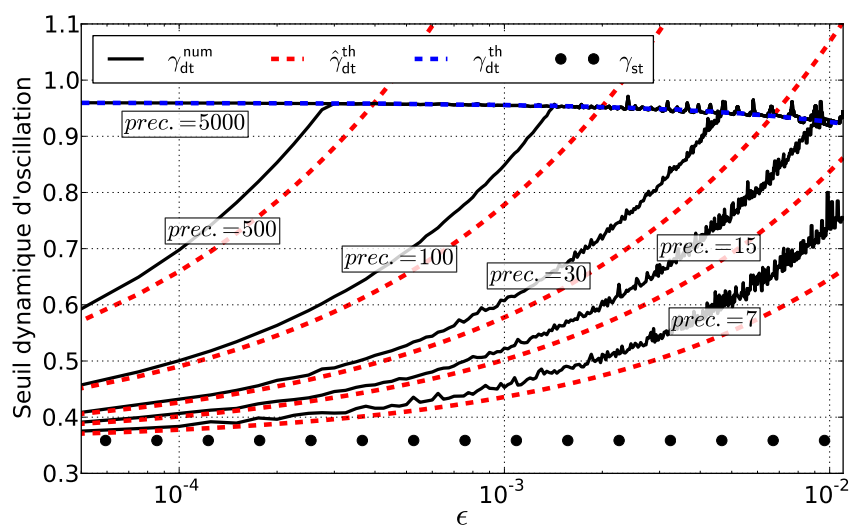
Figure 3.11 – Représentation de \gamma_{dt}^{num} (ligne noire) en fonction de \epsilon pour différentes précisions ( prec. = 7, 15, 30, 100, 500 and 5000 ). Comparaison avec les seuils théoriques statique \gamma_{st} (points noirs) et dynamiques \gamma_{dt}^{th} (pointillés bleus) et \hat{\gamma}_{dt}^{th} (pointillé rouge). \gamma_0 = 0 , \zeta = 0.5 et \lambda = 0.95 .
