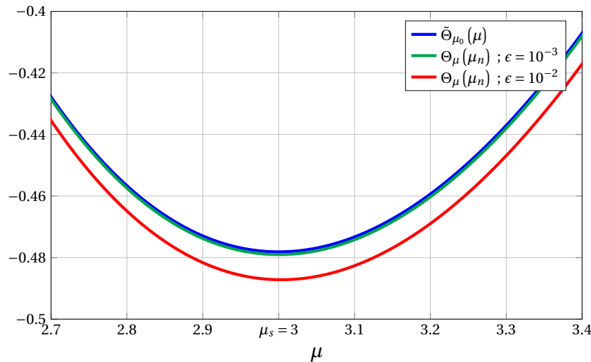
Figure 1.17 – Comparaison entre la fonction \Theta_{\mu_0}(\mu) (ligne verte : \epsilon = 10^{-3} et ligne rouge : \epsilon = 10^{-2} ) et la fonction \tilde{\Theta}_{\mu_0}(\mu) . \mu_0 = 2.2 .
