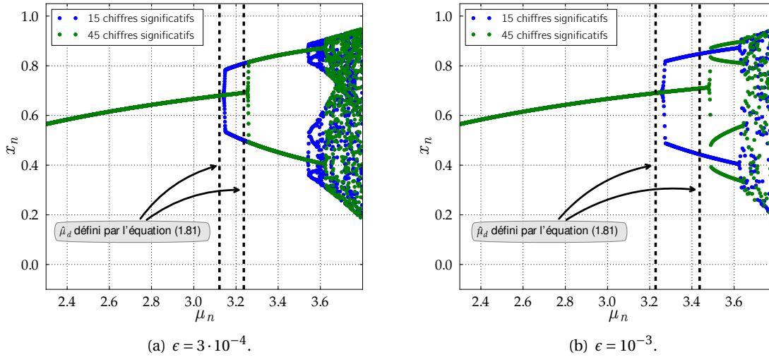
Figure 1.19 – x_n obtenu par simulation du système (1.57) pour différentes précisions de calculs : 15 (•••) et 45 (•••••). x_0 = 0.6 et \hat{\mu}_d est le point de bifurcation dynamique déterminé par l'équation (1.81). (a) \epsilon = 3 \cdot 10^{-4} et (b) \epsilon = 10^{-3} .
