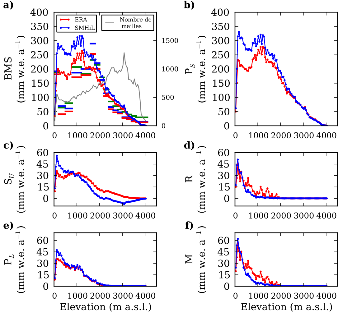
FIGURE 3.8 – BMS et ses composantes intégrés sur la calotte posée par classes d'élévations de 50 m, pour SMHiL (lignes bleues continues) et ERA-Interim interpolé linéairement sur la grille de SMHiL (lignes rouges continues). Les figures présentent les résultats pour a) le BMS b) les précipitations solides c) la sublimation d) le ruissellement e) les précipitations liquides et f) la fonte de la neige. Le nombre de mailles par classes d'élévations est présenté en gris à la figure a) (axe de droite). Les traits épais horizontaux de la figure a) représentent la moyenne du BMS pour les mailles contenant des observations, par classes d'élévations correspondant à la longueur des traits (traits verts pour les valeurs moyennes observées).
