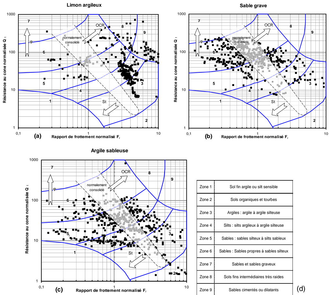
Figure IV-22. Evolution de la résistance au cône normalisée Q_c en fonction du rapport de frottement normalisé F_c dans le limon argileux (a), les sables graves (b), l'argile sableuse (c) et classification des sols (d) (modifié d'après Robertson, 1990)
