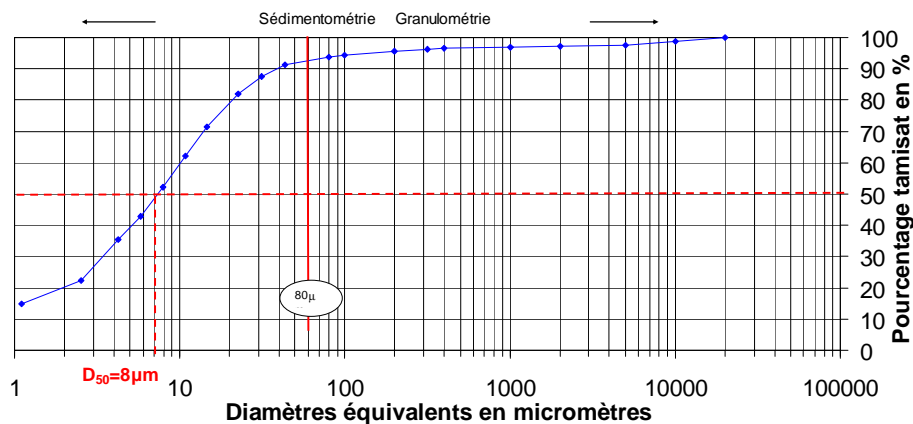
Figure III-10. Courbe granulométrique
