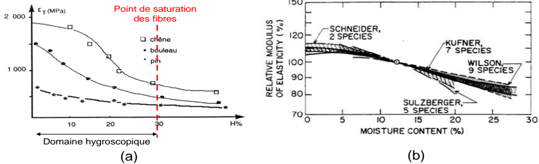
Figure I-16. Variation du module d'élasticité E_{Tangentiel} (a) et du module d'élasticité longitudinal relatif (b) en fonction du taux d'humidité du bois (modifié d'après Pluvinage, 1992 , cité par Dinh, 2011 ; Forest Products Laboratory, 2010 )
