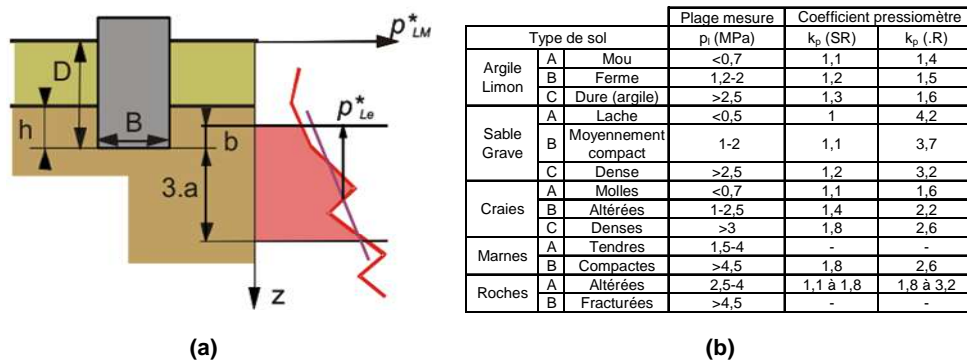
Figure V-29. Pression limite nette équivalente (a) et valeurs du coefficient de portance k_p (b) (modifié d'après le Fascicule 62-V (MELT, 1993))
