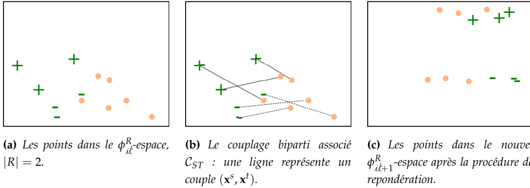
FIGURE 6.2 – Une itération i^{\text{t}} de DASF. Les points sources sont en vert (foncé) (pos. +, neg. -), les points cibles (non étiquetés) sont les ronds orange (clair)
