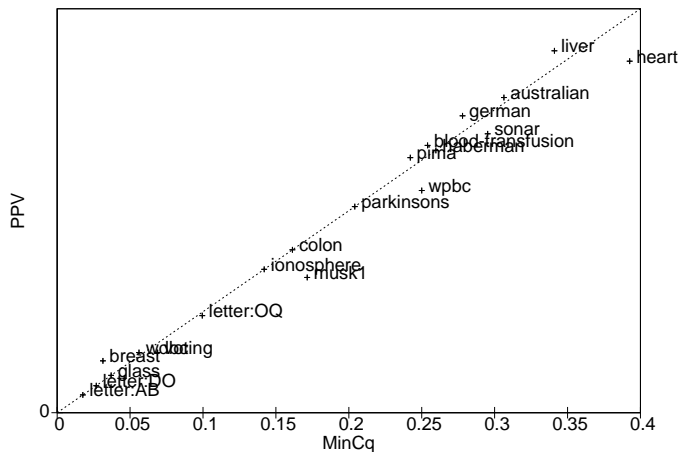
FIGURE 4.1 – Comparaison de \text{MinCq} versus \text{PPV} . Un point correspond au taux d'erreur test des deux algorithmes sur un jeu de données. Un jeu de donnée au-dessus de la bissectrice est en faveur de \text{MinCq} .
