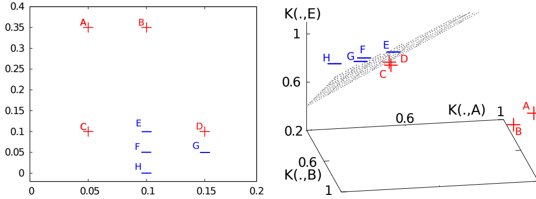
FIGURE 1.4 – Exemple d'un ensemble de points positifs et négatifs. A gauche dans l'espace d'origine, à droite dans le \phi^R -espace avec R = \{A, B, E\} , en gris l'hyperplan séparateur.
