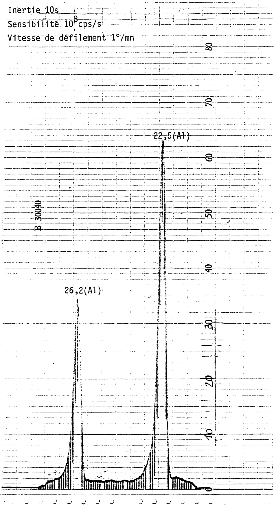
I - FIGURE 5a - Spectre aux RX Alliage d'aluminium X7091 atomisé sous hélium.
