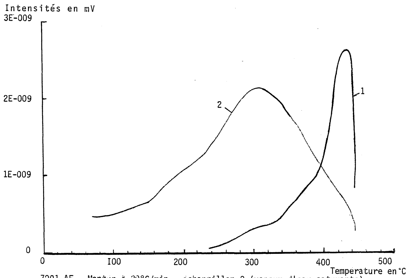
7091 AF - Montee à 20°C/min - échantillon 2 (vapeur d'eau saturante) 1:H 2 , 2:H 2 O
