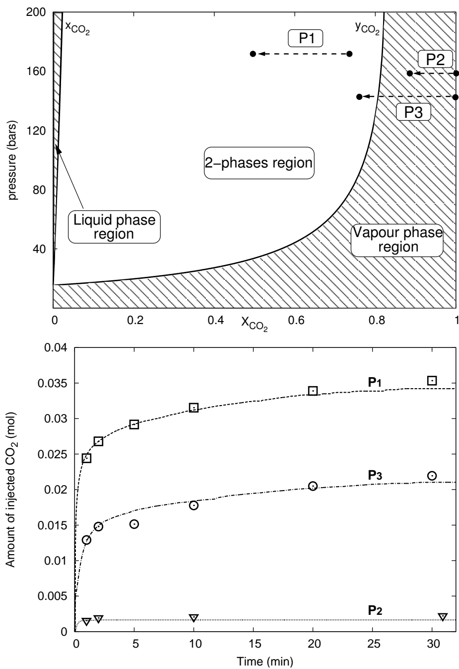
FIGURE 4.4 – Réactivité de la portlandite dans différents environnements : présence initiale d'eau liquide (P1), milieu anhydre (P2), milieu initialement anhydre puis apparition d'eau liquide (P3).
