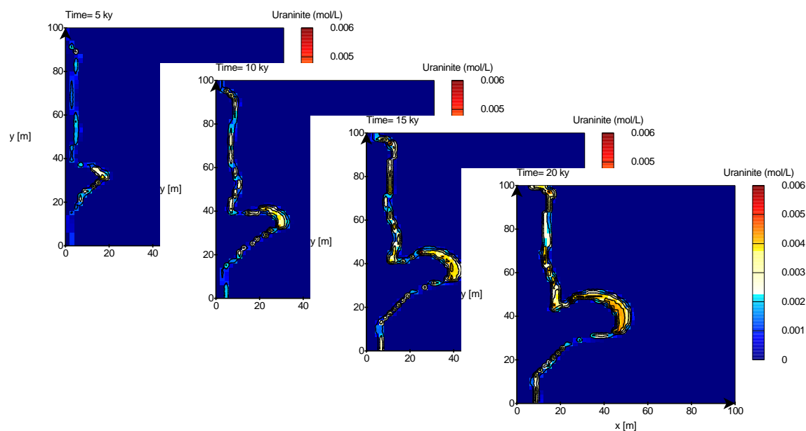
FIGURE 5.5 – Modélisation de la dynamique d'un roll-front d'uranium dans un aquifère hétérogène.
