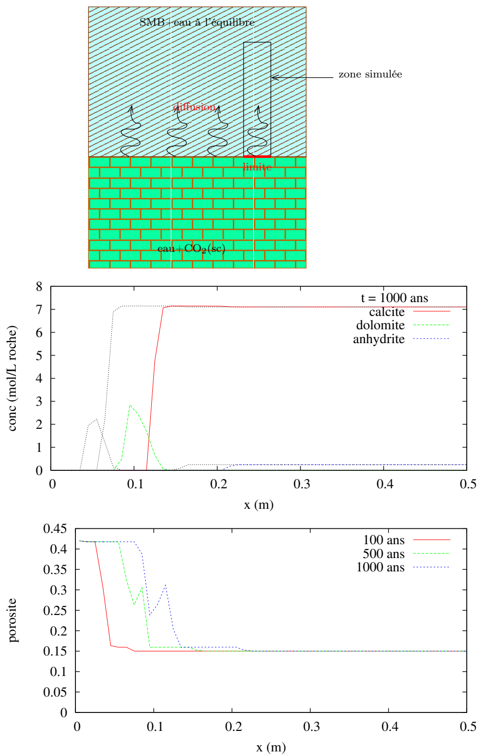
FIGURE 4.5 – Résultat de simulation interaction saumure et CO 2 à l'interface réservoir-couverture : schéma de la zone simulée (en haut), résultats jusqu'à 1 000 ans (au milieu et en bas).
