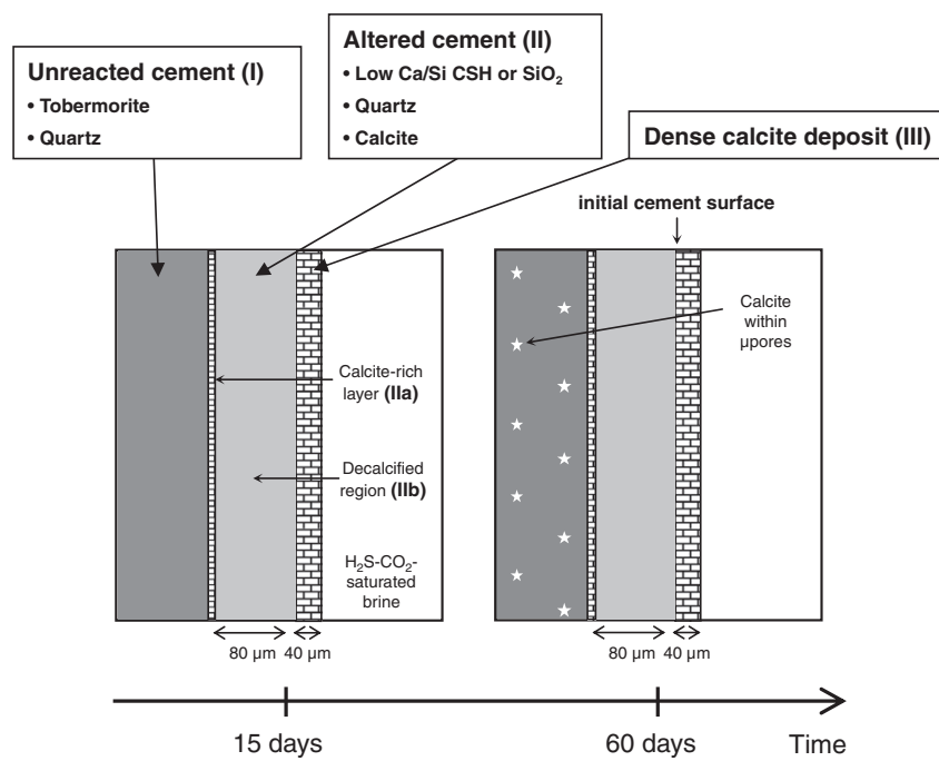
FIGURE 4.1 – Représentation schématique des résultats de l'expérience Jacquemet (2006) d'attaque de ciment par une saumure et une gaz CO 2 /H 2 : position des fronts minéralogiques dans l'expérience avec saumure et gaz (de Jacquemet et al., 2012).
