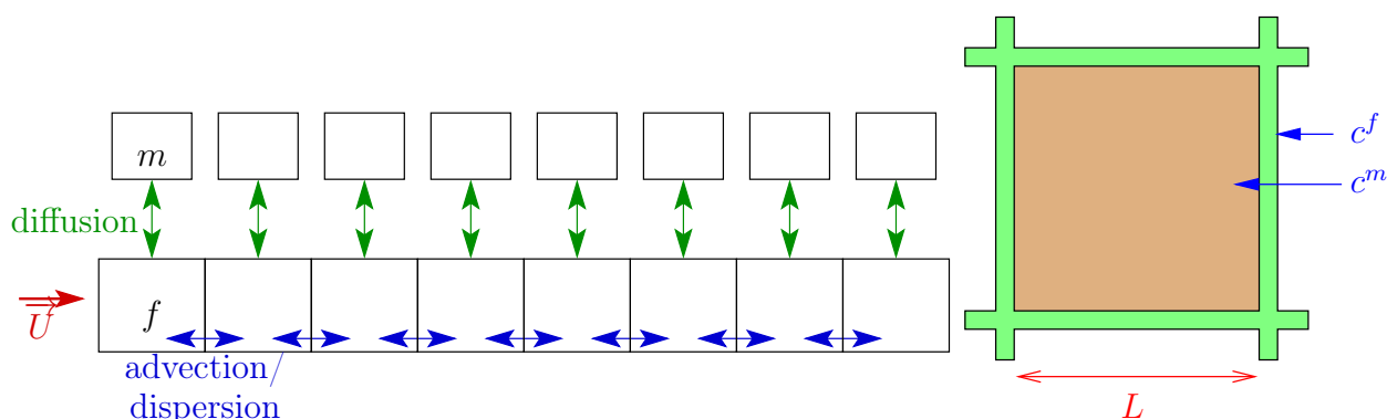
FIGURE 2.4 – Schéma de discrétisation et traitement du transport pour l'option double porosité. Représentation schématisée des transferts entre fracture et matrice.
