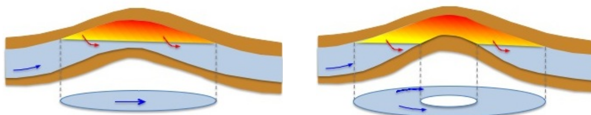
FIGURE 2.6 – Deux types de contact réservoir aquifère : à droite, le contact est intercepté par le mur de la formation aquifère – en 3D, le contact est une couronne et l'aquifère contourne la partie sommitale du réservoir.
