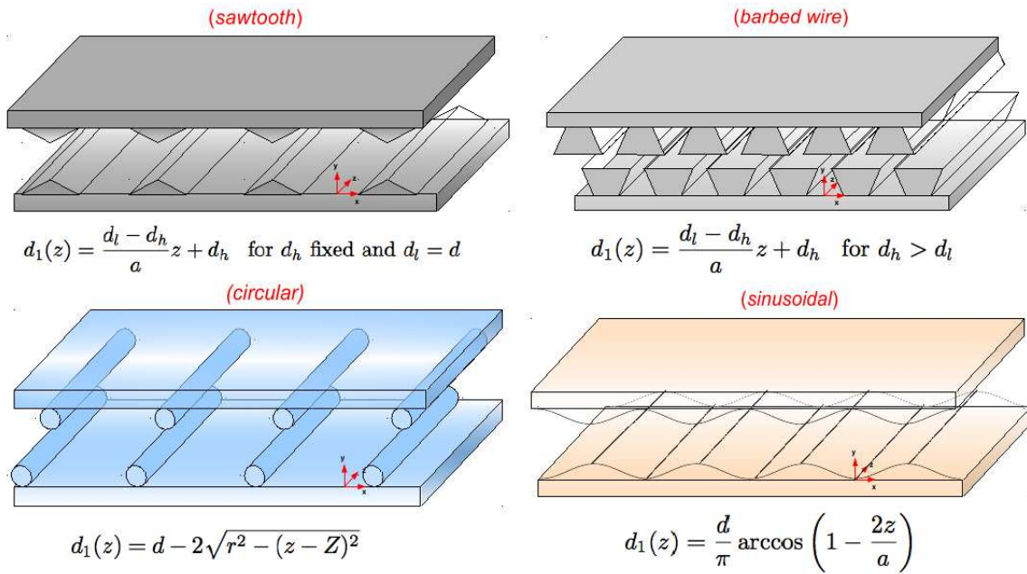
FIG. 7: Différentes géométries de réseaux arbitraires avec spécification associée de la fonction d'espace entre les corrugations d_1(z) .
