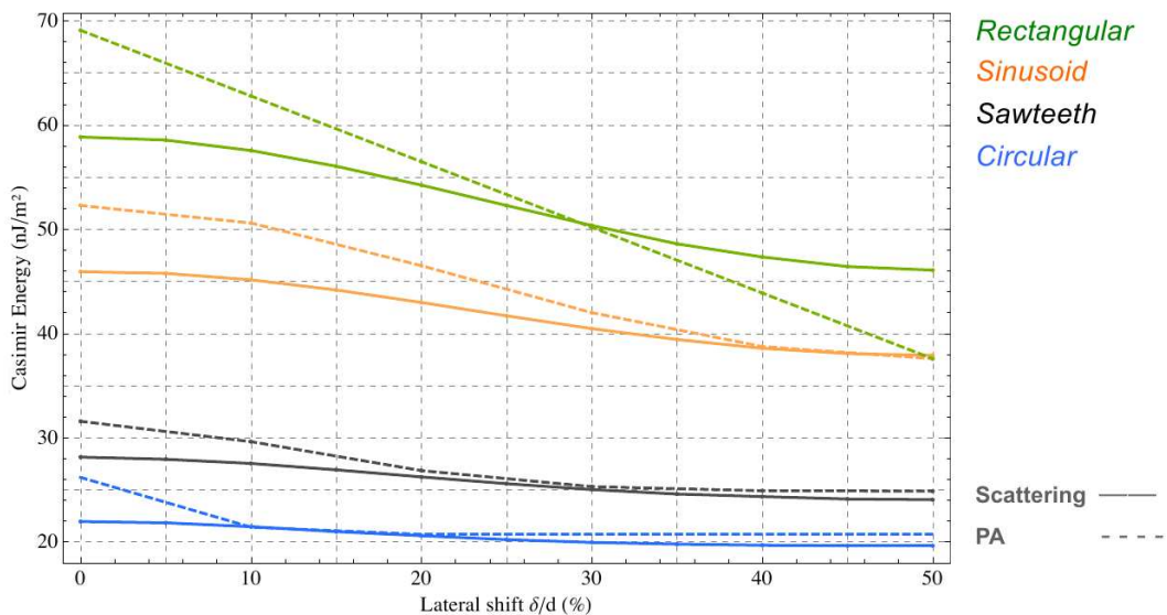
FIG. 8: Dépendance de l'énergie de Casimir en fonction du déplacement latéral \delta pour quatre types de réseaux arbitraires de silicium intrinsèque, pour une distance de séparation L = 100 nm, une période d = 400 nm, et une profondeur de corrugation a = 50 nm. Les profils rectangulaires sont paramétrés par d_1 = 200 (courbe verte), les profils sinusoïdaux par d_1(z) = (400/\pi) \arccos[1 - (z/25)] (courbe orange), les profils en dents de scie par d_1 = 4z + 200 (courbe noire), et les profils circulaires par d_1 = 400 - 2\sqrt{50z - z^2} (courbe bleue). Ces quatre ensembles de résultats exacts provenant de la théorie de diffusion (courbes continues) sont comparés avec les résultats obtenus par l'Approximation de Proximité (courbes en pointillés de couleur respectives).
