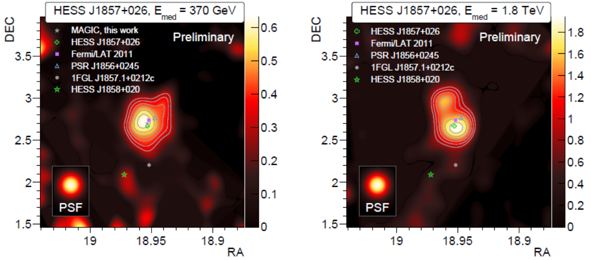
Figure VII.1 - Cartes de flux relatif extraites de la référence Klepser (2011). Le flux relatif est défini comme le rapport du nombre d'évènements en excès sur le nombre d'évènements du fond (Lombardi 2011). La carte de gauche correspond aux énergies entre 0.2 et 1 TeV, tandis que la carte de droite montre les énergies supérieures au TeV. La croix verte montre le centre de l'émission observée par H.E.S.S. , le carré magenta représente celui obtenu par le LAT (Neronov & Semikoz 2010). On voit que la morphologie de l'émission change avec l'énergie.
