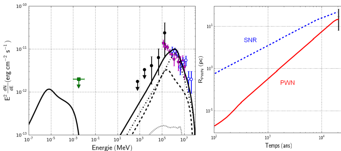
Figure VII.5 - Modèle de nébuleuse supposant un spectre d'injection en loi de puissance brisée pour HESS J1857 + 026. Gauche : Spectre multi-longueur d'onde de la source HESS J1857 + 026 suivant les mêmes conventions que la figure VII.4. Droite : Evolution du rayon en fonction du temps suivant les mêmes conventions que la figure VII.4.
