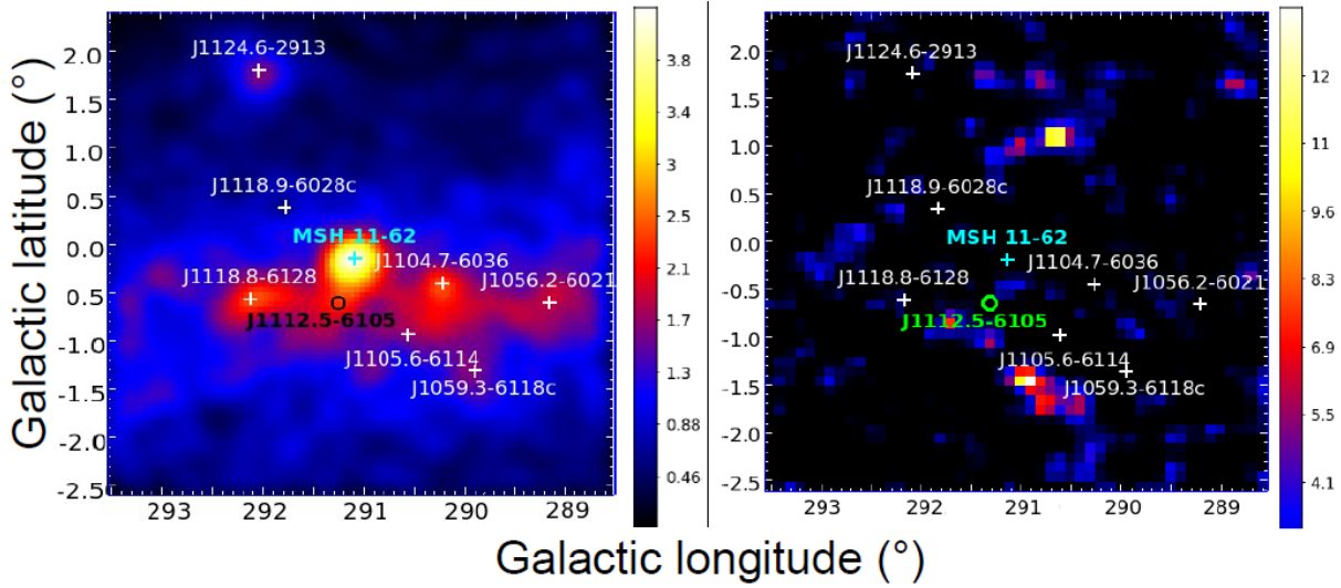
Figure VI.2 - (Gauche) Carte de photons observés par le LAT dans une région de 5^\circ centrée sur MSH 11–62 (unité arbitraire). Pour réduire l’émission venant du diffus Galactique, seuls les photons d’énergie supérieure à 1 GeV ont été sélectionnés. Cette carte est lissée par une Gaussienne de 0.25^\circ . (Droite) Carte de TS obtenue après soustraction de toutes les sources incluses dans le modèle. Cette carte est obtenue en ajustant la normalisation d’une source ponctuelle dont le spectre est décrit par une loi de puissance d’indice \Gamma = 2 dont on fait varier la position selon les axes de la carte. On peut voir qu’il n’existe aucun résidu dont le TS dépasse 13 (ce qui correspond à une significativité < 4\sigma ) ce qui signifie que le modèle reproduit bien la région sans source supplémentaire. Sur les deux cartes, les points blancs représentent les sources 2FGL qui font partie du modèle. Le cercle (noir/magenta) représente la position de la source associée au pulsar PSR J1112–6103 et la position de MSH 11–62 est symbolisée par une croix bleue.
