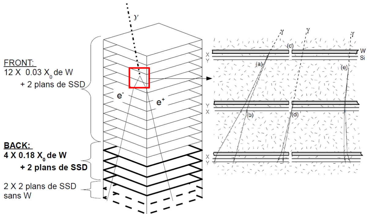
Figure IV.3 - Schéma d'une tour du trajectographe du LAT. Les différentes parties présentées dans le texte y sont résumées. Un zoom sur la zone de conversion du photon en une paire électron positron \gamma a été ajouté. Ces figures sont respectivement adaptées de Ackermann et al. (2012a) et Atwood et al. (2009). Sur le zoom à droite, on peut voir différentes configurations de conversions dans le trajectographe. Tandis que (a) représente une conversion idéale dans le tungstène proche des pistes de silicium, (d) montre le cas où la trace de l'un des deux composants de la paire e^\pm est manquée ce qui dégrade la résolution angulaire. Afin de diminuer le nombre de conversions loin de toute mesure, les feuilles de tungstène ne recouvrent que la surface des détecteurs à pistes de silicium (c).
