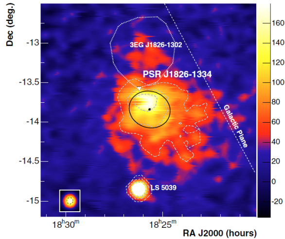
Figure III.3 - Carte d'excès de la nébuleuse HESS J1825–137 extraite de Aharonian et al. (2006c). Les contours de la source avec une significativité de 5, 10 et 15 \sigma sont représentés par les pointillés blancs. La position de PSR J1826–1334 est symbolisée par la flèche blanche. On voit que l'extension de la nébuleuse est asymétrique par rapport à la position du pulsar. Le maximum d'émission est aussi décalé par rapport au pulsar.
