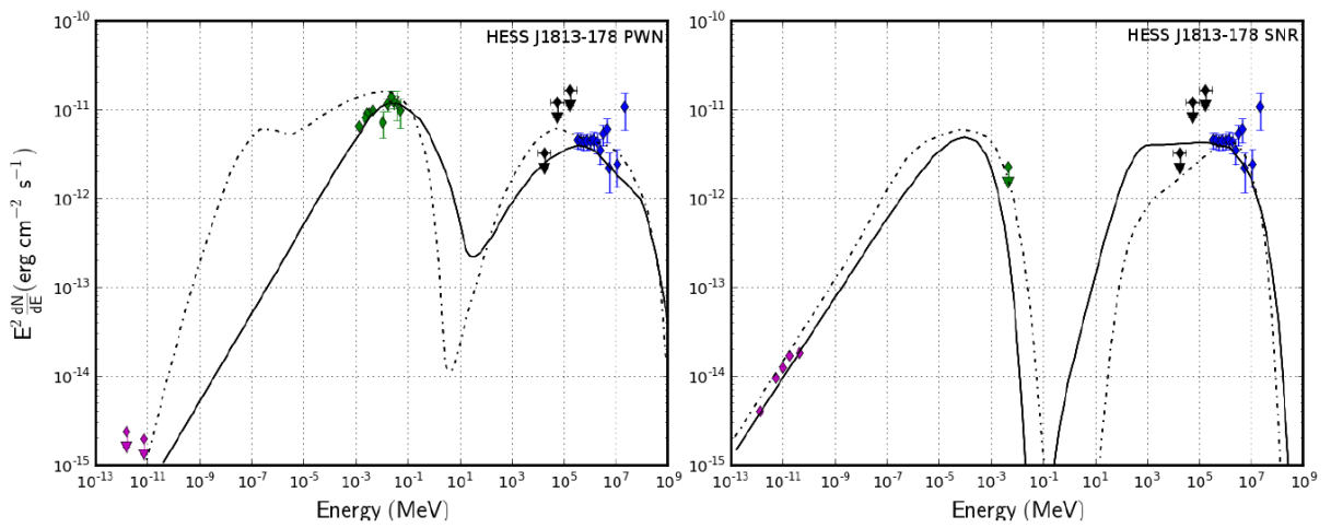
Figure VIII.10 - Distribution spectrale en énergie pour la source HESS J1813 – 178. (Gauche) Modèle dans lequel l'émission observée par le LAT est émise par la PWN. (Droite) Modèle dans lequel l'émission observée par le LAT est émise par le SNR. Les lignes pleines et tiretées correspondent respectivement aux modèles proposés par Funk et al. (2007a) et par Fang & Zhang (2010b). De gauche à droite, les points magentas, verts, noirs et bleus correspondent aux données radios, X, LAT et TeV.
