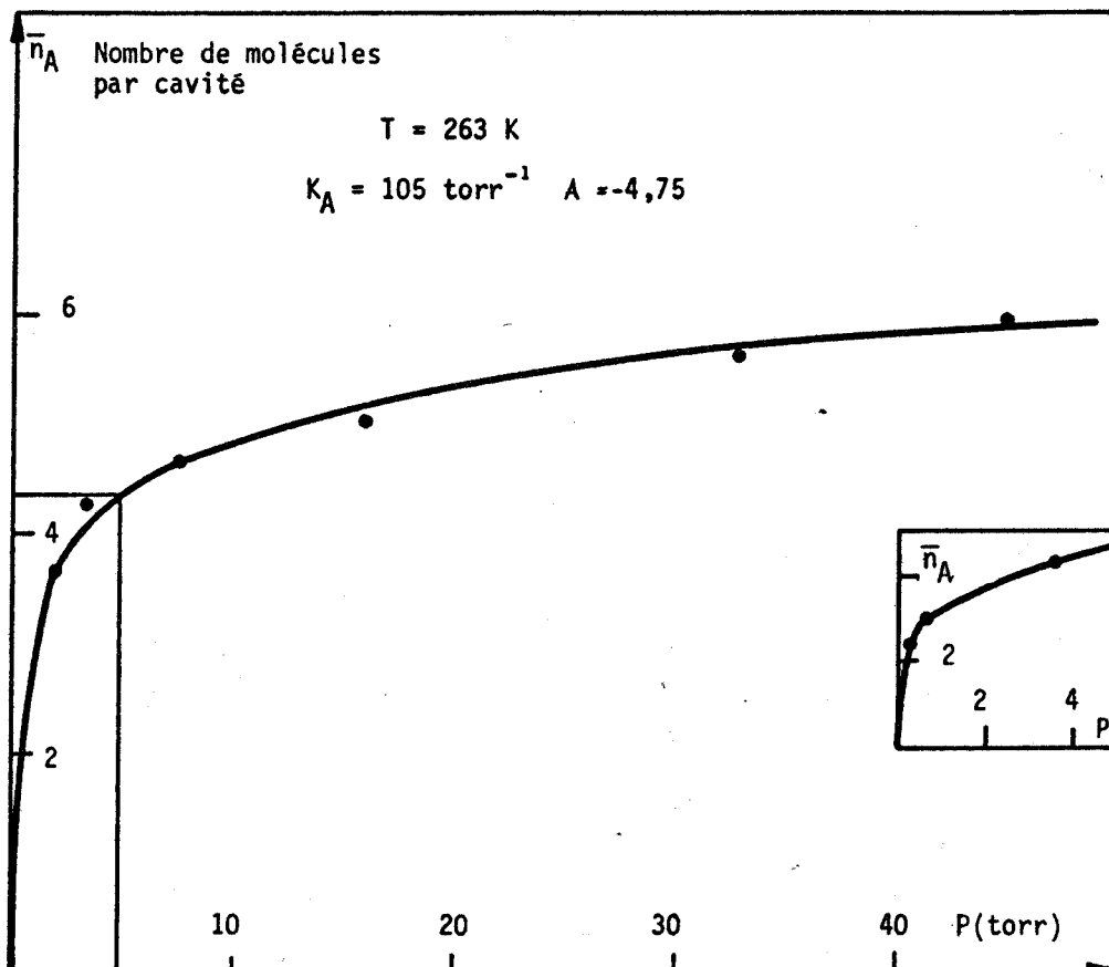
Figure II-5 : Adsorption de \text{CO}_2 sur la zéolithe 4A
