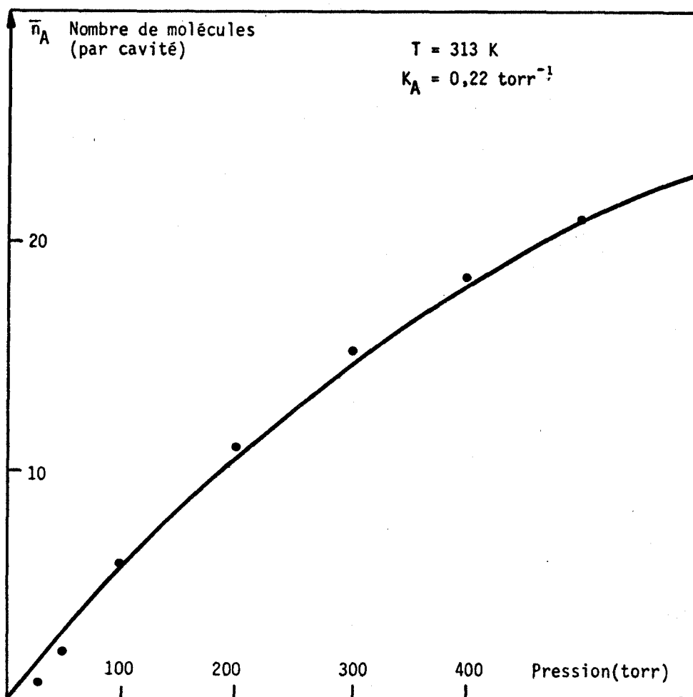
Figure II-20 : Adsorption de C_2H_6 sur 13 X
