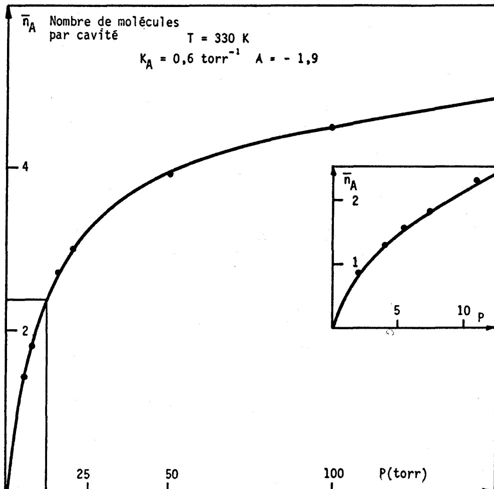
Figure II-7 : Adsorption de CO 2 sur la zéolithe 4A
