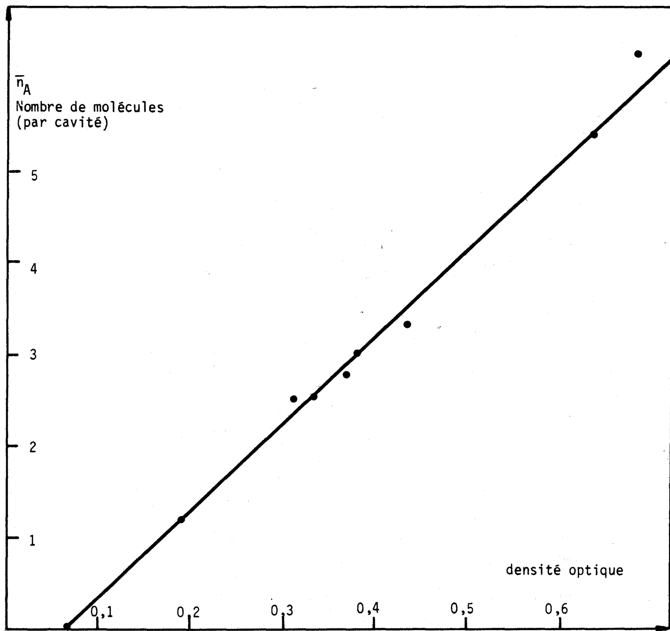
Figure II-13 : Etalonnage par la méthode d'adsorption infra-rouge de \text{CO}_2 adsorbé sur la zéolithe 4A.
