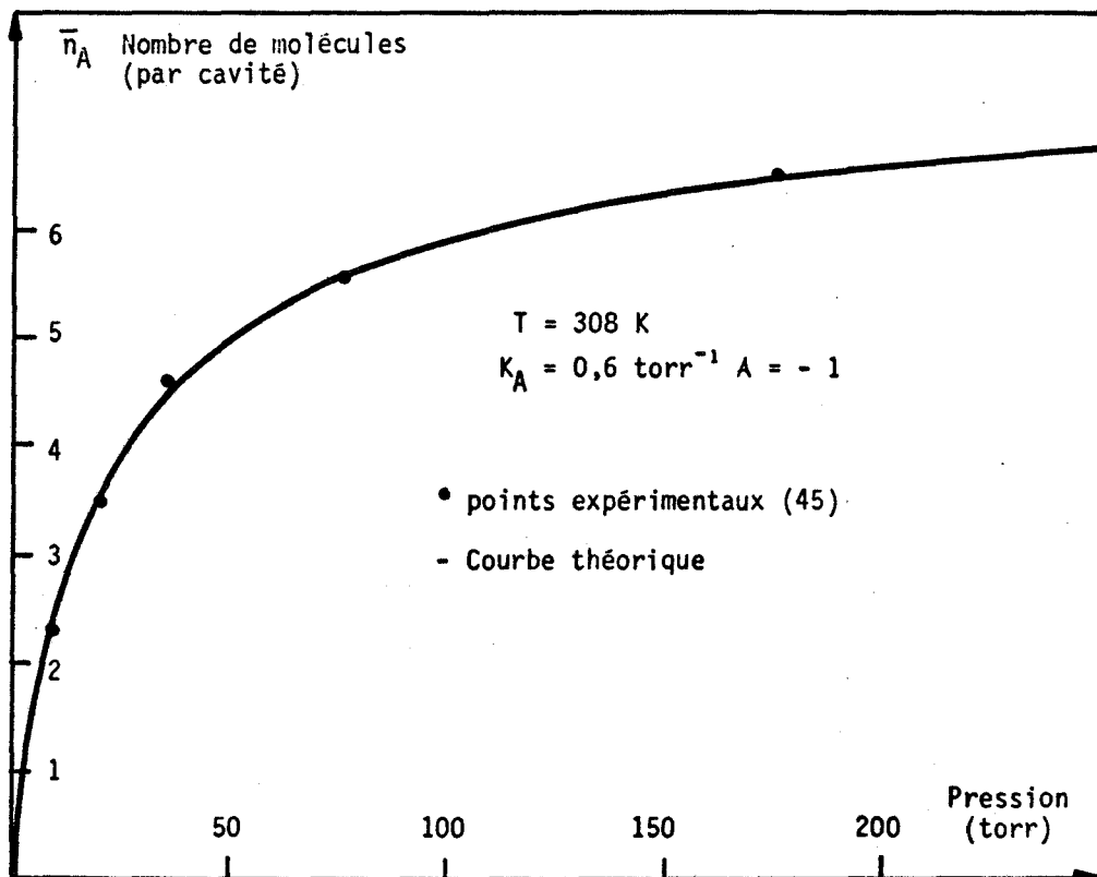
Figure II-2 : Adsorption de CO_2 sur la zéolithe 5A
