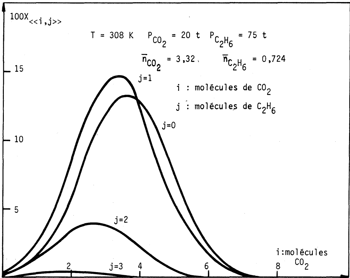
Figure III-4 : Loi de répartition du mélange \text{CO}_2 - \text{C}_2\text{H}_6 dans la zéolithe 5A
