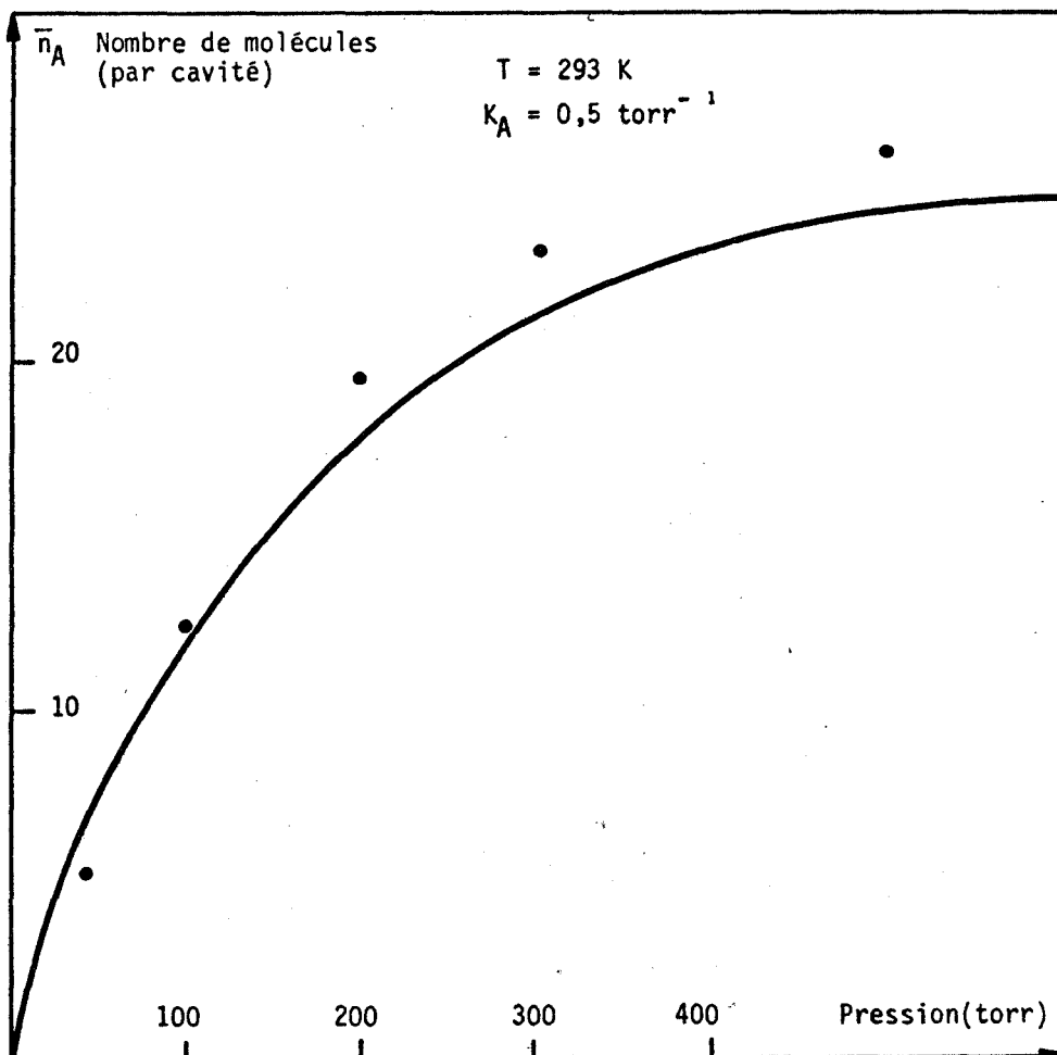
Figure II 19 : Adsorption de C_2H_6 sur 13 X
