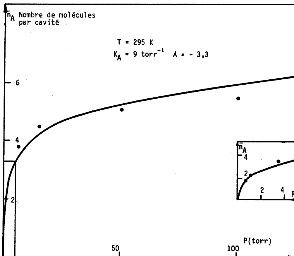
Figure II-6 : Adsorption de \text{CO}_2 sur la zéolithe 4A
