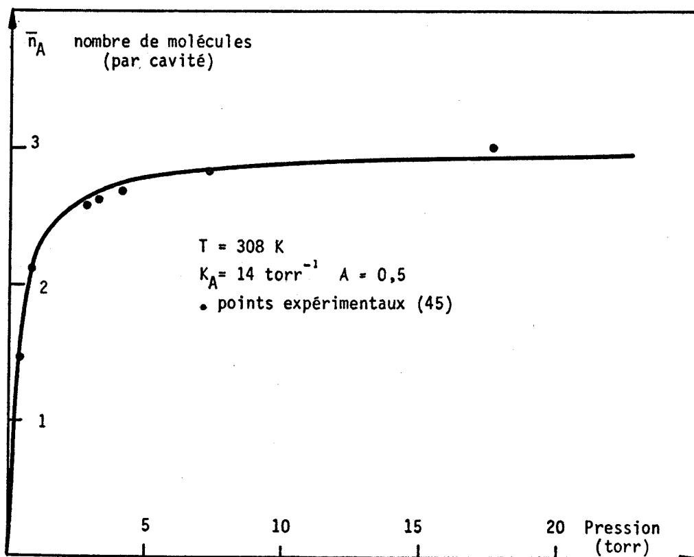
Figure II-4 : Adsorption de \text{C}_4\text{H}_{10} sur la zéolithe 5A
