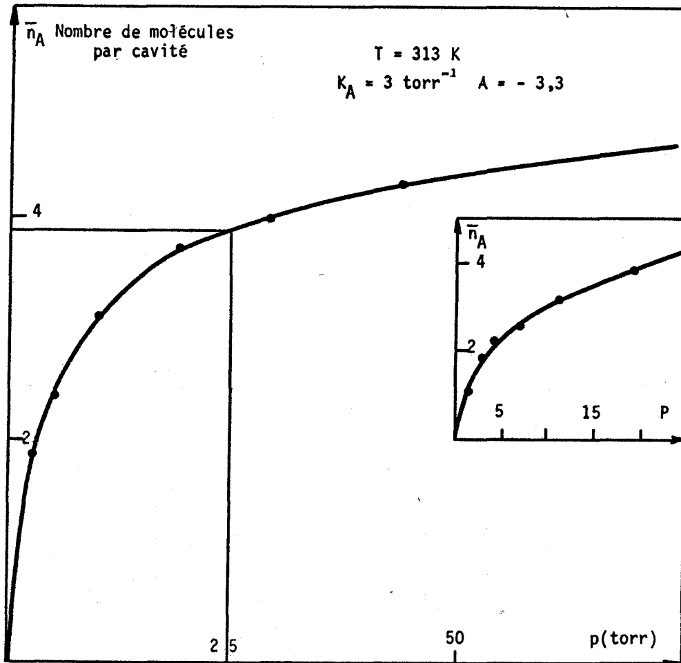
Figure II-7 : Adsorption de CO 2 sur la zéolithe 4A
