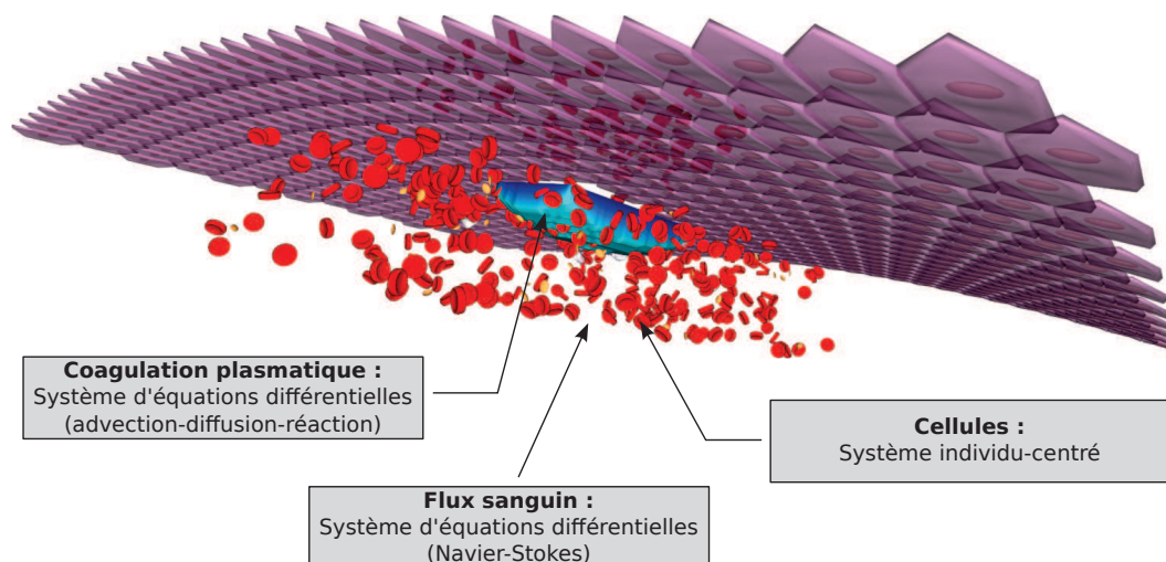
FIGURE 3.12 – Phénomènes présents au sein du vaisseau sanguin virtuel – Cette figure propose un visuel de notre vaisseau sanguin virtuel et met en évidence les phénomènes présents en son sein. En outre, le type de modélisation envisagé pour chacun d'eux est précisé.
