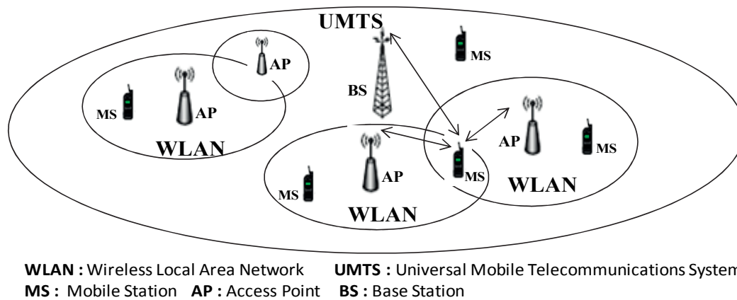
Figure 1.4 - Architecture de réseaux hétérogènes.
