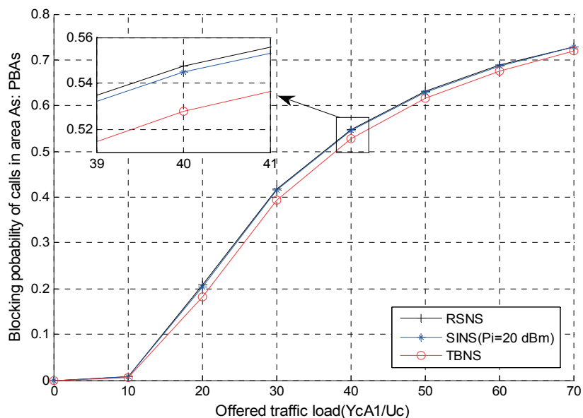
Figure 5.5 - Probabilité de blocage dans la zone A_5 .
