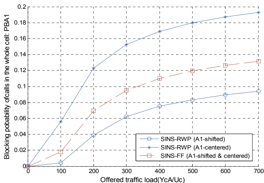
Figure 5.9 - Mobilité : Probabilité de blocage dans la cellule totale A_1 .
