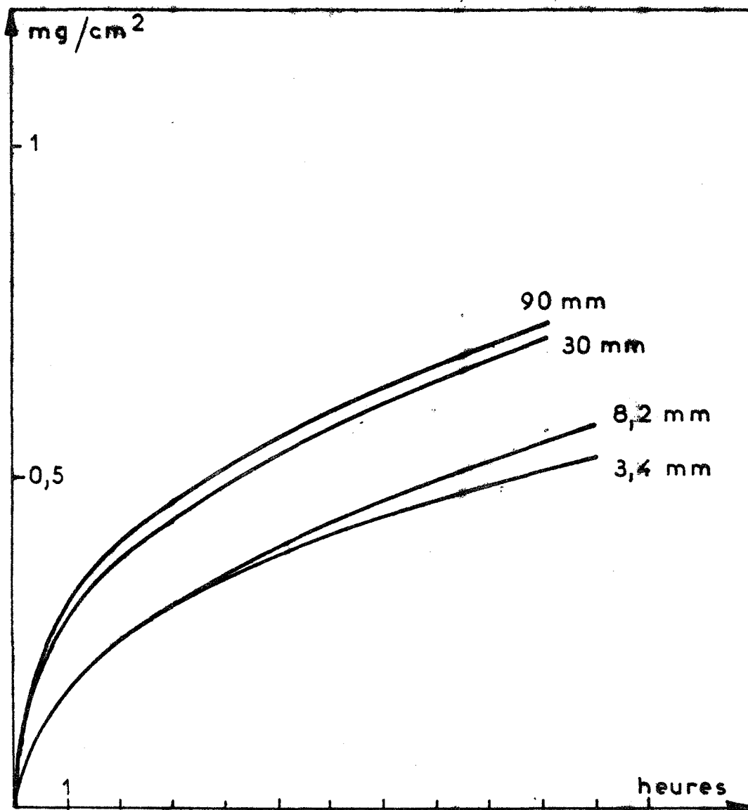
Ni-Nb: \alpha 0,94 atome % de Nb Cinétique d'oxydation T = 820^\circ \text{C}
