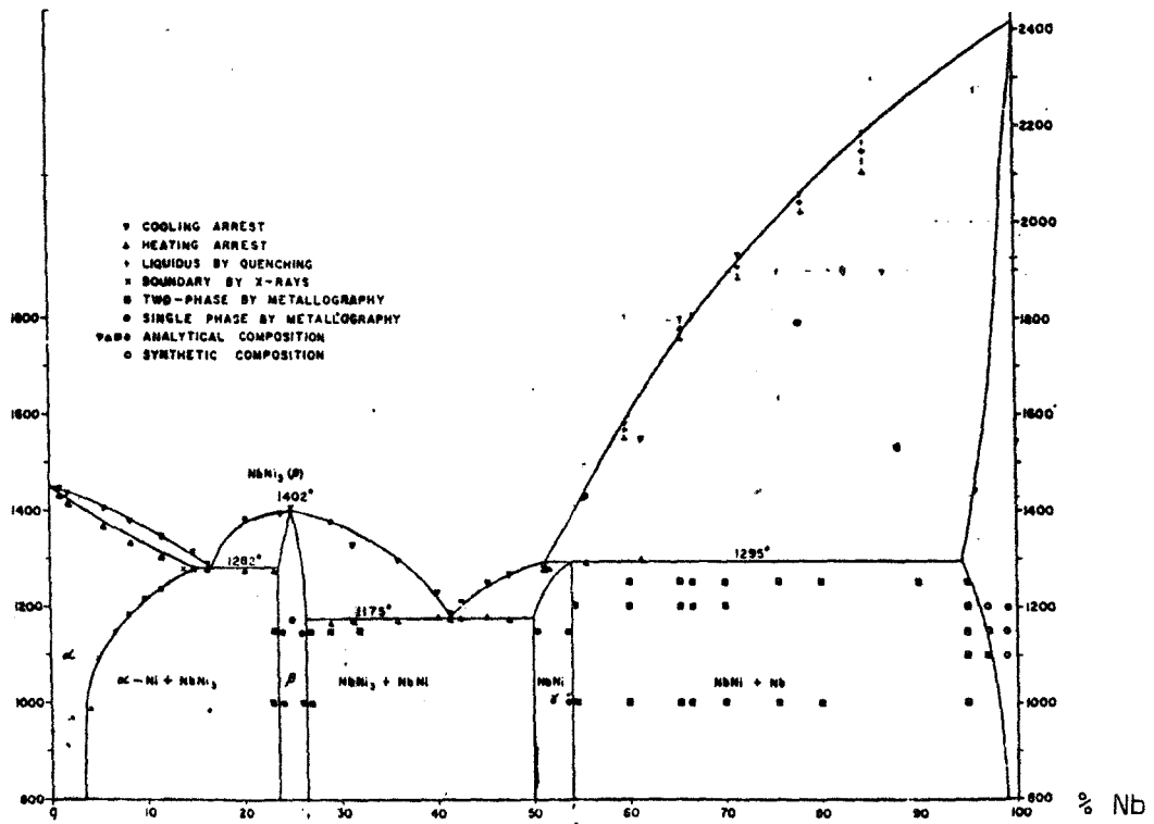
Diagramme d'équilibre du système Nobium - Nickel d'après I.J. DUERDEN et W. HUME-ROTHERY
