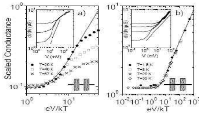
FIGURE 5.4 – Conductance différentielle en fonction de la tension pour différentes valeurs de la température. (a) Lorsque le nanotube a un point contact par le “bulk”, la valeur de l’exposant est \alpha = 0.46 . (b) Lorsque le nanotube a un point contact par les extrémités, la valeur de l’exposant est \alpha = 0.63 . Les lignes solides représentent les courbes théoriques. D’après Bockrath et coll. [21].
