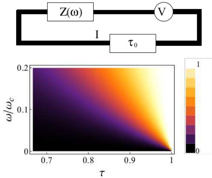
FIGURE 4.3 – En haut : Schéma représentant un conducteur à un canal de transmission \tau_0 en série avec une résistance. En bas : Profil du coefficient de transmission en fonction de la fréquence \omega/\omega_c et la transmission effective \tau .
