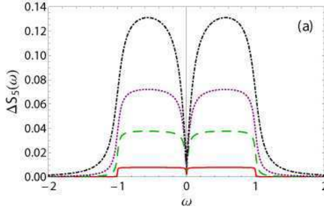
FIGURE 3.6 – Corrélateur en excès \Delta S_5(\omega) en unité de eV_{dc}G_q , en fonction de la fréquence en unité de eV_{dc}/\hbar pour différentes valeurs de l'amplitude de rétrodiffusion \Gamma_B à température k_B T = 0.001eV_{dc} . Les amplitudes de rétrodiffusion sont : \Gamma_B = 0.01eV_{dc} (ligne solide rouge), \Gamma_B = 0.05eV_{dc} (ligne verte hachurée), \Gamma_B = 0.1eV_{dc} (ligne violet en pointillé) et \Gamma_B = 0.2eV_{dc} (ligne hachurée et en pointillé noire).
