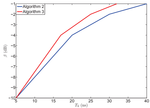
Figure 6: la relation entre le temps de bit et l'efficacité énergétique
