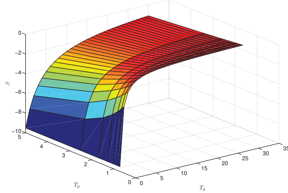
Figure 5: Relation entre l'efficacité énergétique, le temps de l'impulsion et le temps de garde
