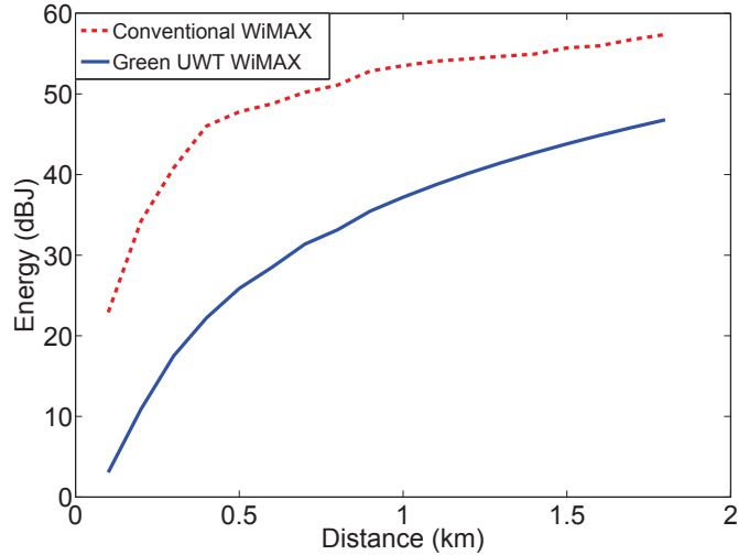
Figure 3: Energie de transmission pour WiMAX
