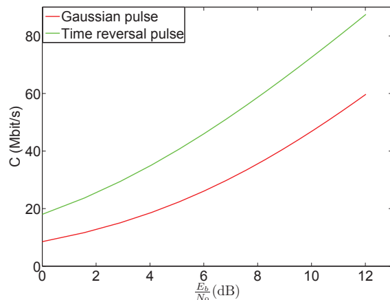
Figure 7: Performances de l'impulsion gaussienne et l'impulsion de retournement temporel pour les différents valeurs de \frac{E_b}{N_0}
