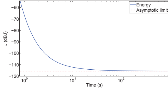
Figure 1: Relation entre l'énergie et le temps de communication
