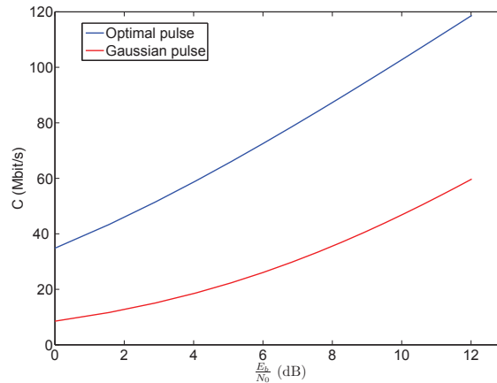
Figure 8: Performances de l’impulsion gaussienne et l’impulsion optimale pour les différents valeurs de \frac{E_b}{N_0}
