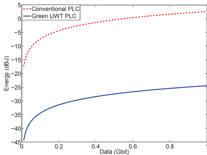
Figure 4: Energie de transmission pour CPL
