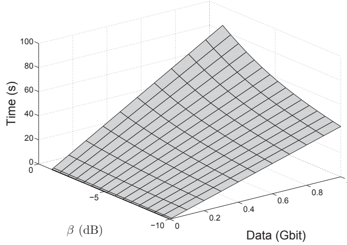
Figure 2: Relation entre l'efficacité énergétique, la quantité d'information et le temps de communication
