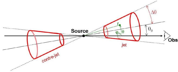
FIGURE 3.9.: Géométrie de l'éjecta relativiste.
