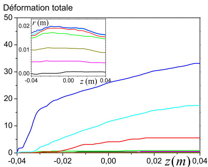
Figure 4.4 – Écoulement d'un fluide à seuil à travers un pore (à V = 0,16 \text{ mm/s} ). Déformation totale subie par les éléments de fluide le long des lignes de courant (voir figure insérée) initialement à différentes distances de l'axe central : (de bas en haut) 0, 5, 10, 15, 16, 16,5 et 17,25 mm.
