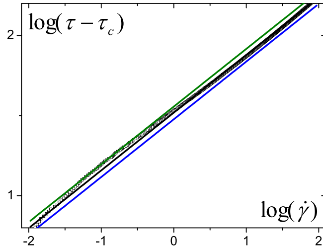
Figure 2.10 – Différents facteurs de consistance k sont envisagés pour ajuster le modèle de HB : 30Pa.s^n (ligne bleue), 33Pa.s^n (ligne noire) et 36Pa.s^n (ligne verte); les carrés représentent les données expérimentales.
