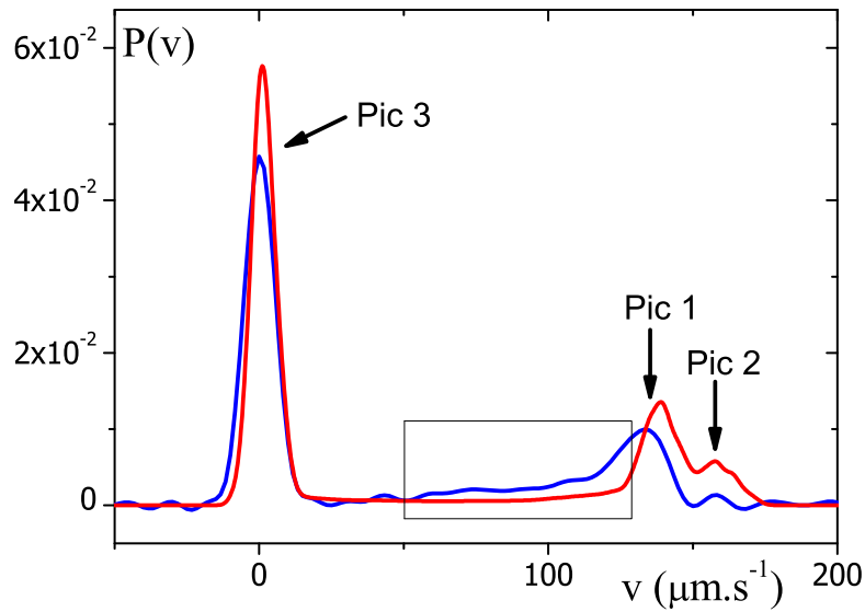
Figure 2.45 – PDF de vitesse ou densité de vitesse pour l'écoulement à travers le gros pore à V = 0,16 \text{ mm/s} obtenue à partir d'une carte de vitesse (courbe rouge) présentée sur la figure 4.1) et directement (courbe bleue).
