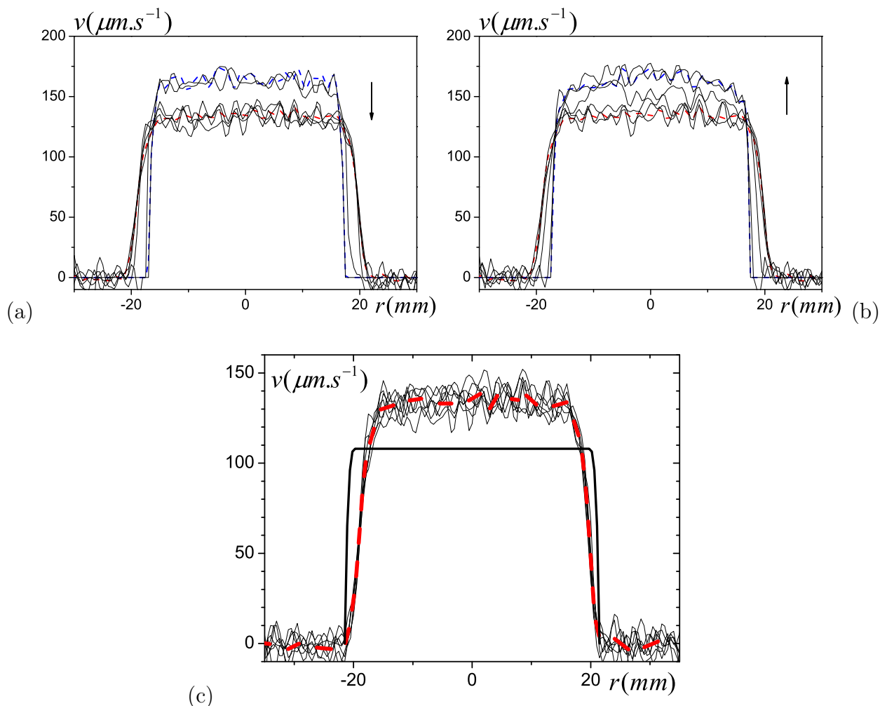
Figure 4.3 – Écoulement d'un fluide à seuil à travers une boîte cylindrique (à V = 0,16\text{mm/s} ) : profils de vitesse longitudinale obtenus à partir des images en fonction de la distance à l'axe de symétrie à différentes position z séparées par des intervalles de 0,5\text{cm} : (a) de 0,5 à 4,5\text{cm} (entrée), (b) de -4,5 à 0,5\text{cm} (sortie), (c) de -1,5 à 1,5\text{cm} (centre). La ligne pointillée bleue est la vitesse moyennée entre 3,5 et 4,5\text{cm} dans (a) et entre -4,5 et -3,5\text{cm} dans (b). La ligne pointillée rouge est la vitesse moyennée entre -1,5 et 1,5\text{cm} . La ligne noire continue (en trait épais) correspond à la théorie d'un écoulement uniforme dans une conduite d'un rayon de 21,5\text{mm} . La flèche indique le sens de l'écoulement.
