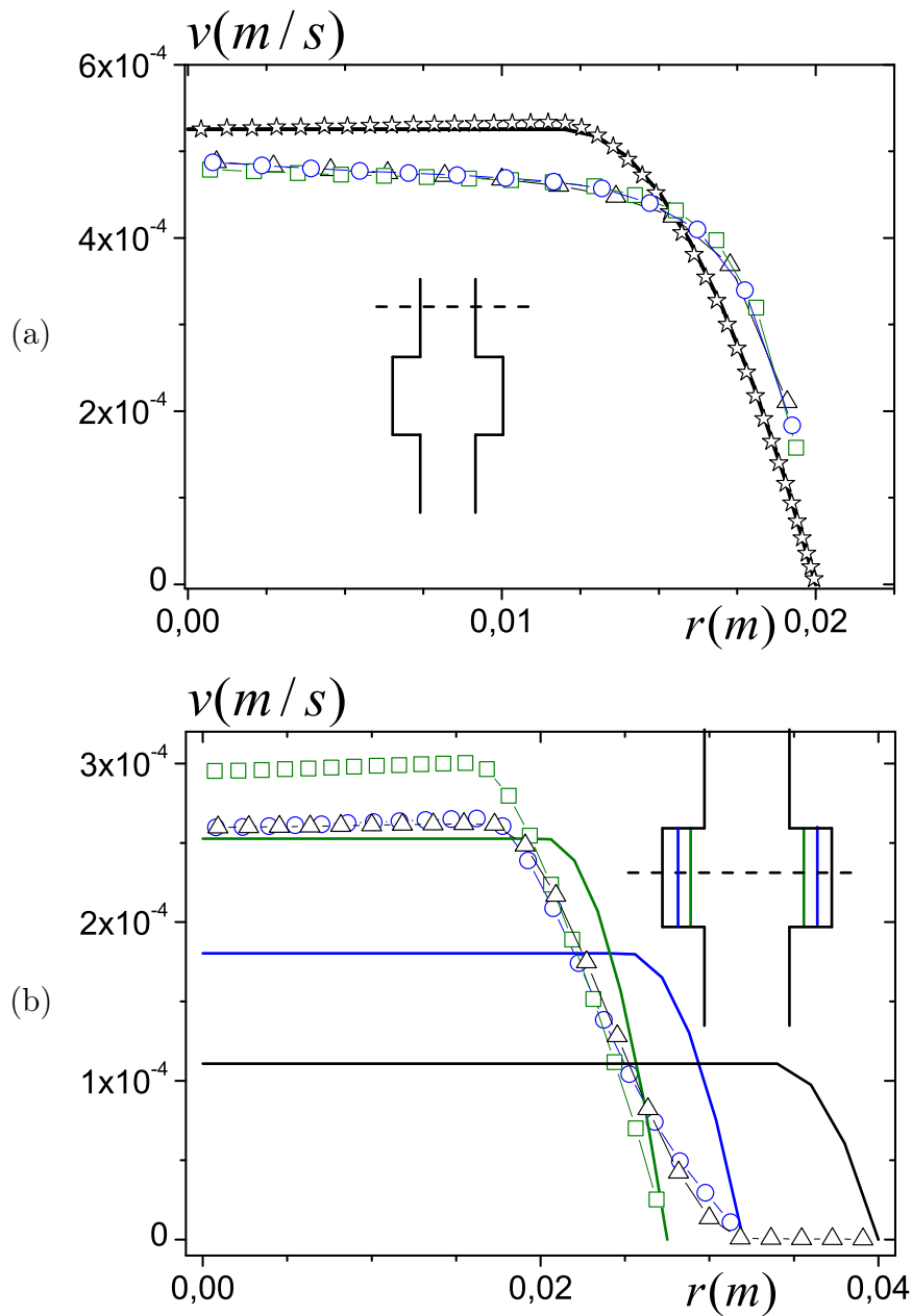
Figure 4.28 – Écoulement dans un pore modèle à Bi = 10 avec d = 4 cm et une longueur de 8 cm avec le maillage M1 . Le diamètre de la conduite la plus large D varie entre D = 8 cm (triangles noirs), D = 6,4 cm (ronds bleus) et D = 5,5 cm (carrés verts). (a) : profils de vitesse dans la conduite de diamètre d . La ligne continue représente le profil de vitesse théorique dans une conduite de diamètre d et les étoiles représentent le profil de vitesse numérique avec le maillage M4 (le plus fin). (b) : profils de vitesse au centre du pore de diamètre D . Les lignes continues représentent les profils de vitesse théoriques dans une conduite de diamètre D .
