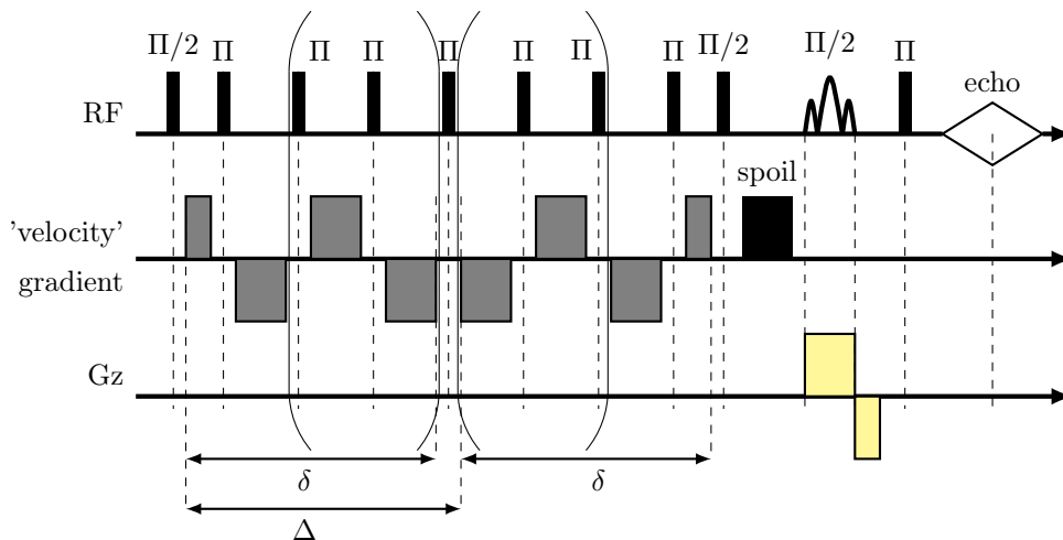
Figure 2.39 – Séquence PGSE utilisée pour obtenir les densités de vitesses. Avant l'application du spoiler, n_{pulse} impulsions \Pi sont appliquées.
