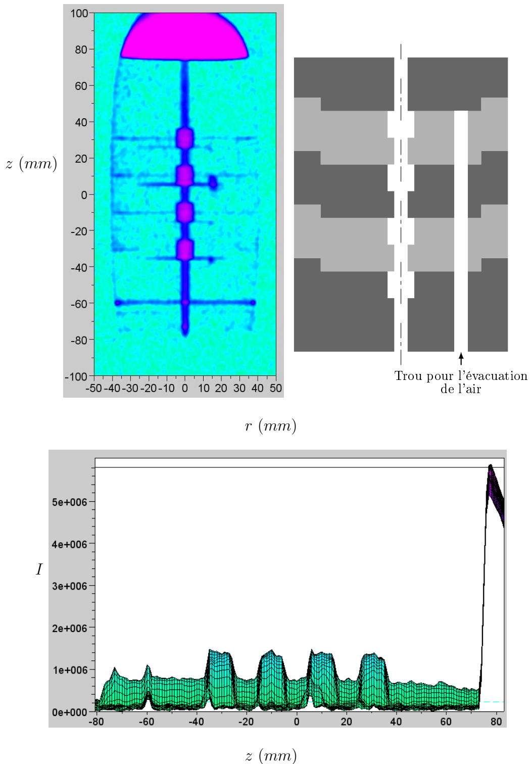
Figure 2.23 – Intensité 2D projetée du signal RMN ( I en unité arbitraire) sur une section (z, r) des pores modèles de 1\text{cm} (en haut) et sur une coupe longitudinale (en bas). En haut à droite : schéma de principe des différentes parties qui forment la série de pores.
