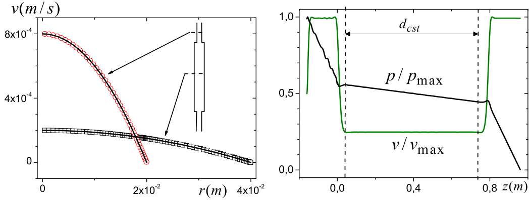
Figure 4.23 – Pore avec LR = 10 , CR = 2 , Bi = 10^{-3} et maillage M4 . A gauche : profils de vitesse longitudinale dans la petite conduite (ronds), z = -0,08 \text{ m} , et au centre du pore (carrés), z = 0,4 \text{ m} . Les lignes continues représentent le profil théorique d'écoulement dans une conduite simple. A droite : vitesse longitudinale (en vert) et pression (en noir) le long de l'axe de révolution en fonction de la hauteur, ces deux grandeurs sont adimensionnées par leur valeur maximale. Les pointillés délimitent la zone où l'écoulement est uniforme et équivalent à celui dans une conduite droite simple. La longueur de cette zone est d_{\text{cst}} .
