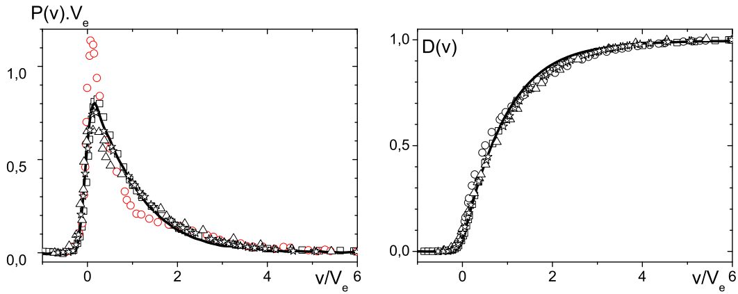
Figure 5.24 – PDF de vitesse longitudinale adimensionnées par la vitesse moyenne de l'écoulement (à gauche) et les distributions de vitesse associées : nos données dans les billes de 0,5 \text{ mm} ( Bi = 6,5 en trait noir épais, V_e = 0,12 \text{ mm/s} ), celles avec un fluide newtonien fig. 1 de Lebon [53] (carrés - V_e = 3,55 \text{ mm/s} ), fig. 5a Johns [46] (ronds - V_e = 1,5 \text{ mm/s} ), fig. 4 de Tessier [97] (triangles - V_e = 1,1 \text{ mm/s} ) et avec un fluide rhéo-fluidifiant : fig. 9 de Mertens [63] (étoiles - V_e = 16 \text{ mm/s} ).
