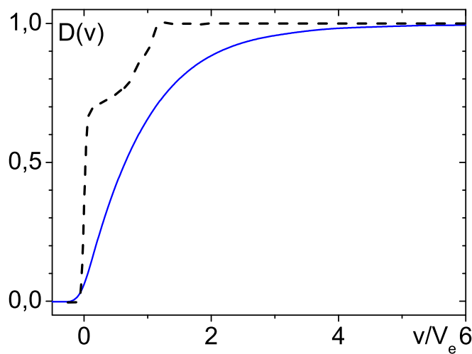
Figure 5.19 – Distributions de vitesse longitudinale d’écoulement dans des billes collées de 0,5mm (trait bleu, Bi = 6,5 ) et dans le pore modèle de 7cm adimensionnées par la vitesse moyenne d’écoulement.
