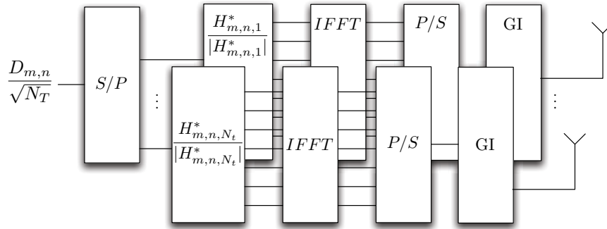
FIGURE 4.3 – Système MISO OFDM utilisant la technique EGT
