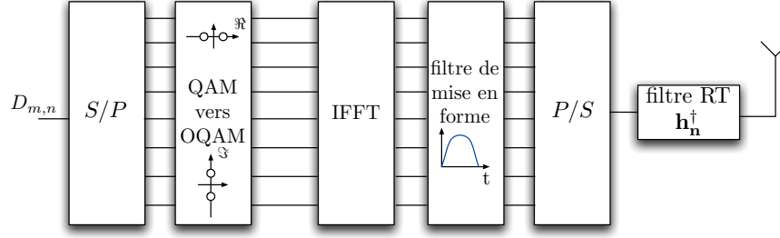
FIGURE 5.5 – Système OFDM/OQAM utilisant le Retourneement Temporel
