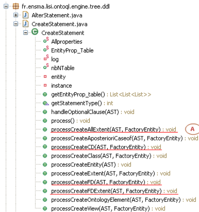
FIGURE 7.23 – Implémentation des clauses dans OntoQL
