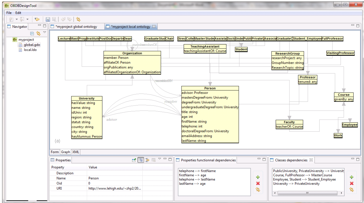
FIGURE 7.5 – Affichage de l'ontologie locale sous forme de diagramme de classes.
