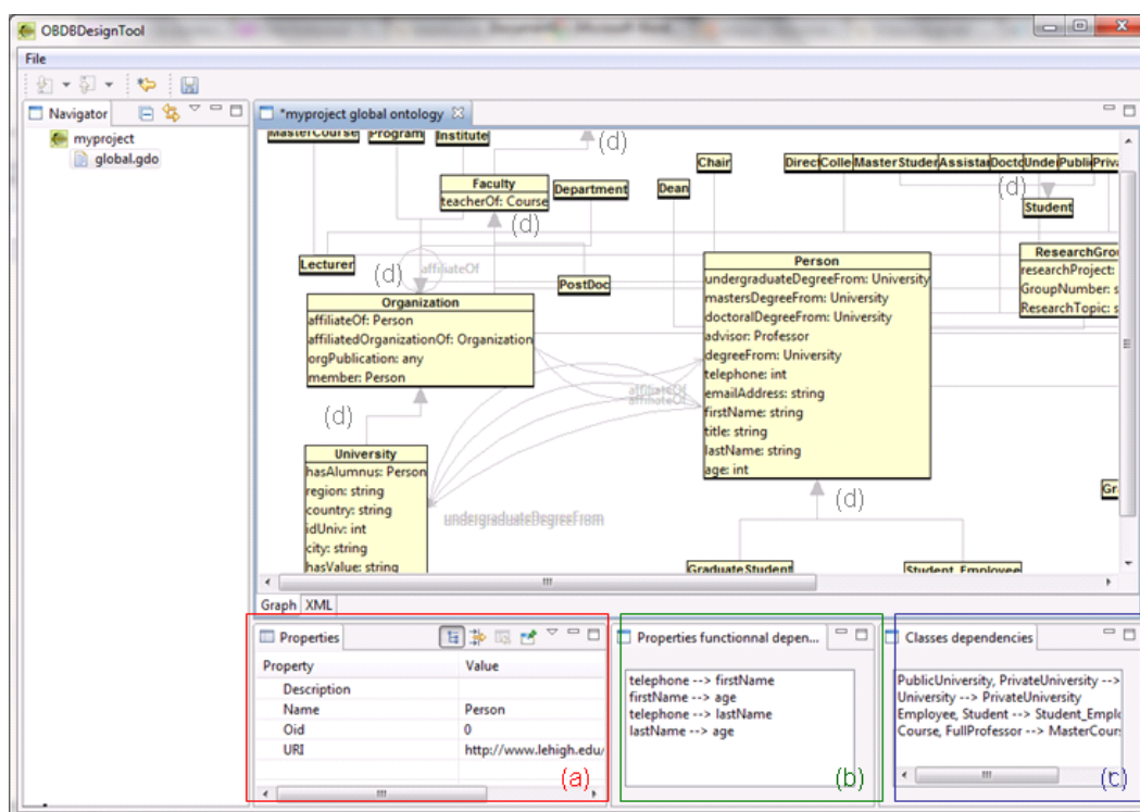
FIGURE 7.3 – Exemple de visualisation de l'ontologie globale
