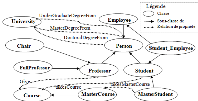
FIGURE 4.11 – Exemple d'ontologie locale canonique: un fragment de LUBM.
