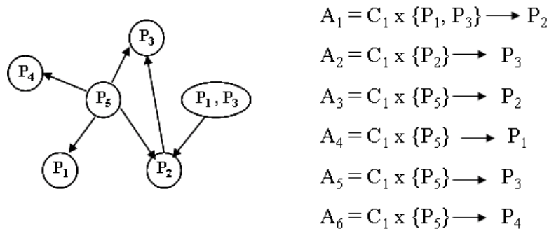
FIGURE 4.2 – Exemple de graphe de dépendances entre les propriétés des données
