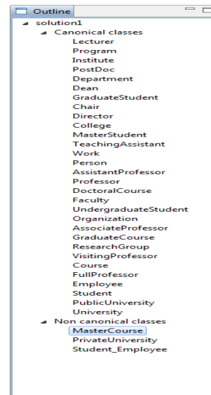
FIGURE 7.7 – Exemple de classification de classes selon la solution 1
