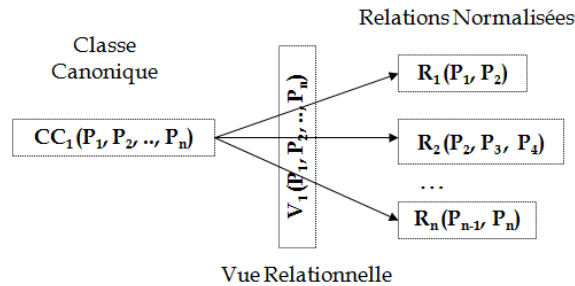
FIGURE 4.7 – Définition d'une vue relationnelle.
