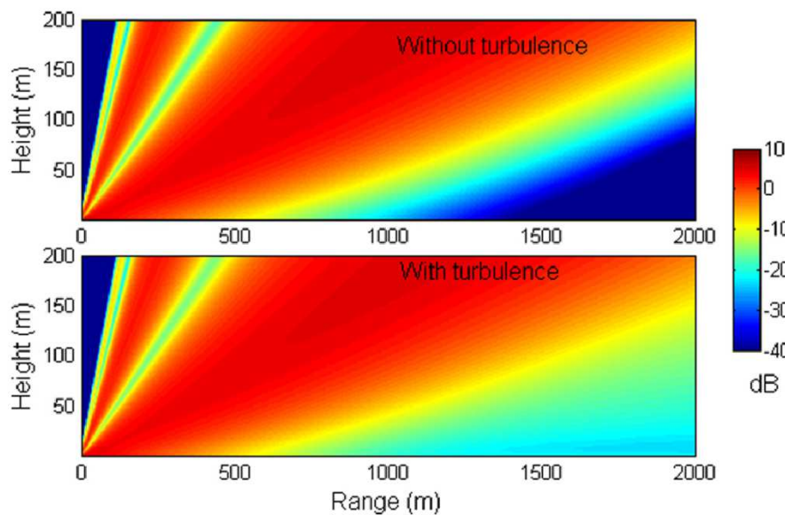
FIGURE B.1 – Niveau sonore (en dB), donné par une méthode de PE prenant en compte la turbulence atmosphérique, dans le cas d’une réfraction vers le haut. (haut) propagation sans turbulence, (bas) propagation avec turbulence. Figure extraite de Cheinet (2012).
