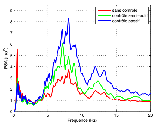
(d) Pendule de frottement ; signal sismique artificiel n° 2
