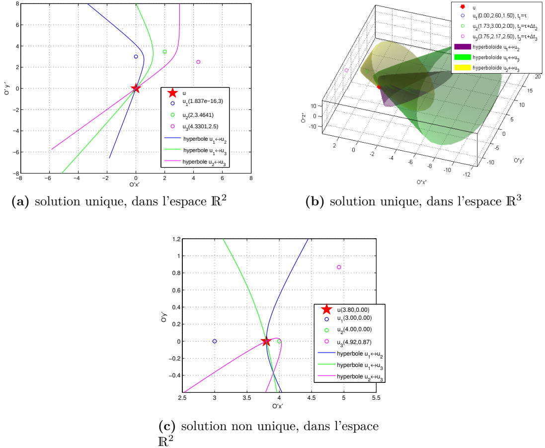
Figure 1.9 – Identification des coordonnées d'un hypocentre u , par la méthode des hyperboles. Les solutions sont situées à l'intersection des hyperboles en \mathbb{R}^2 , et hyperboloïdes en \mathbb{R}^3 , respectivement
