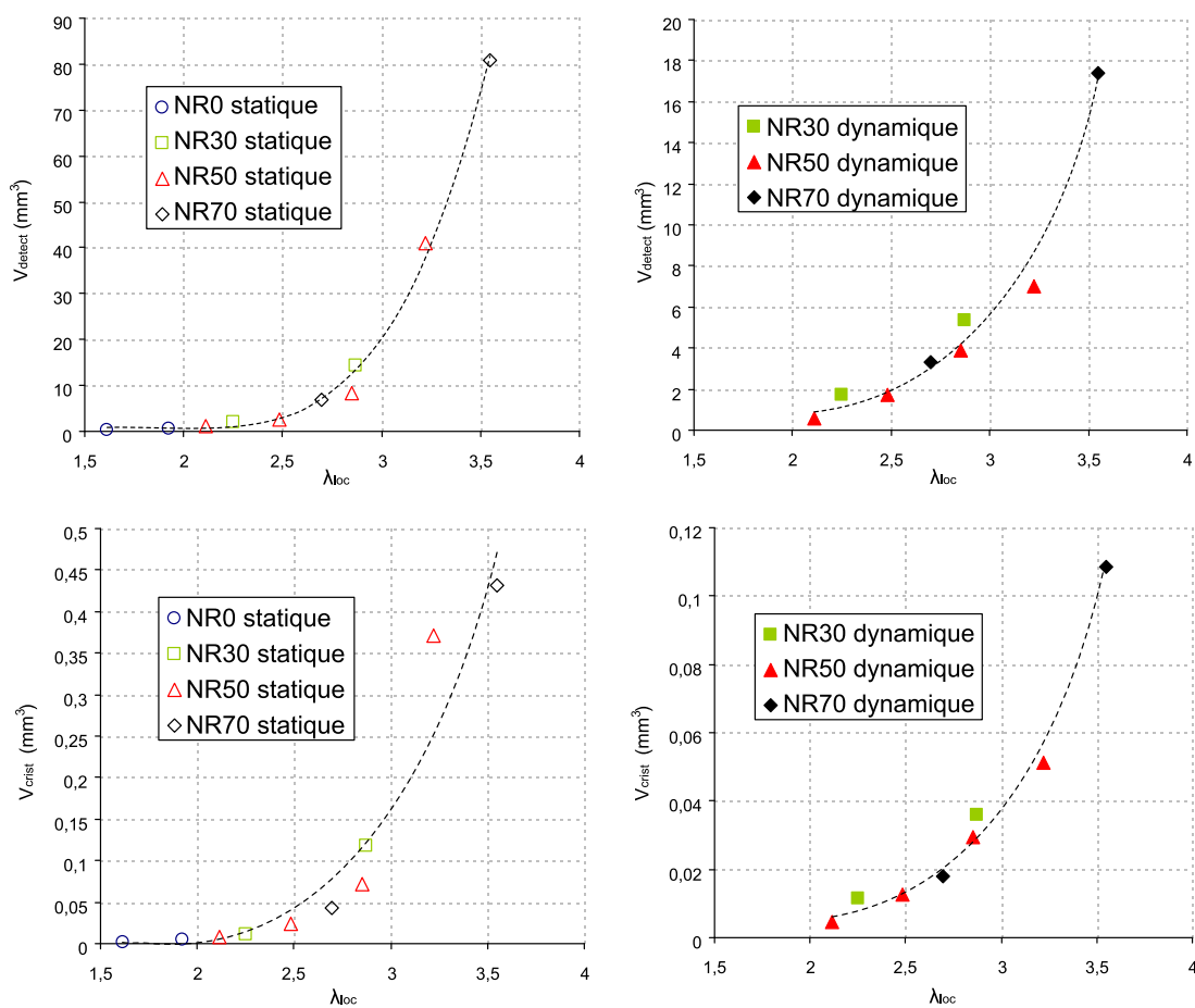
FIGURE 6.39 – Evolution des paramètres V_{detect} et V_{cris} , pour les différents mélanges NR chargés au noir de carbone, en fonction l'élongation appliquée corrigée par la formule de Nielsen \lambda_{loc} . Les courbes en traits pointillés représentent des fonctions ajustées sur les valeurs expérimentales, et servent seulement à donner une tendance d'évolution des données.
