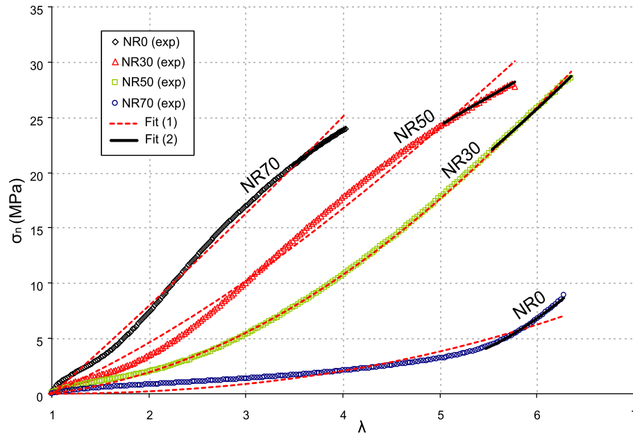
FIGURE 6.10 – Ajustements du modèle GNH sur les données expérimentales des courbes de traction à rupture, dans le cas des quatre matériaux à matrice naturelle. Les courbes pointillées et les courbes pleines représentent respectivement les ajustements effectués sur l'intégralité des points de mesure (Fit 1) et les ajustements effectués seulement sur les derniers points de mesure de la courbe de traction (Fit 2).
