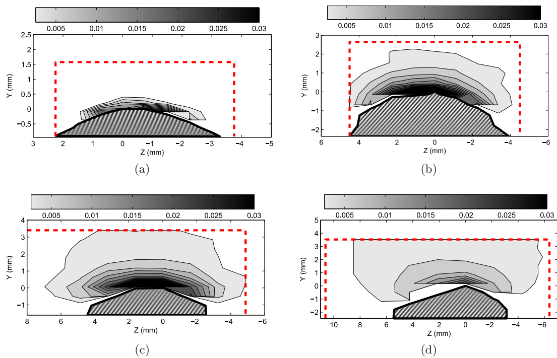
FIGURE 6.37 – Cartographies lissées des valeurs de \chi mesurées par WAXD en dynamique dans le cas des mélanges chargés, pour une même élongation maximale \lambda = 1,92 de sollicitation. a) NR0 : G = 6270 \text{ J/m}^2 . (b) : NR30, G = 10200 \text{ J/m}^2 . (b) : NR50, G = 14140 \text{ J/m}^2 . (d) : NR70, G = 20392 \text{ J/m}^2 . On notera que les échelles des axes varient pour les différentes cartographies.
