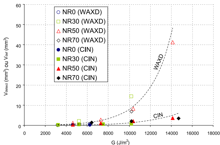
FIGURE 6.44 – Evolution des paramètres V_{detect} et V_{def}(\lambda_{1,lim} = \lambda_{c(0,25\%)}) mesurés en statique en pointe de fissure en fonction du taux de restitution d'énergie G pour les différents matériaux. Les courbes en traits pointillés représentent les ajustements sur les données expérimentales à partir d'une relation exponentielle.
