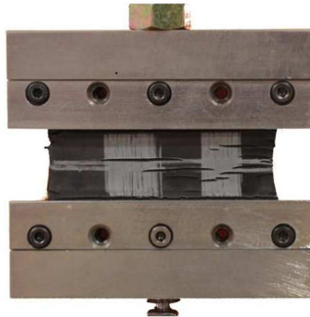
FIGURE 4.23 – Eprouvette demi-PS de mélange NR50 multifissurée en surface par oxydation étirée à \lambda = 1,65 . Les traces blanches effectuées au crayon à gomme sur la surface de l'éprouvette permettent de distinguer plus facilement les pointes de fissures lors des essais de fissuration.
