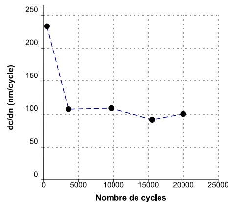
FIGURE 3.5 – Vitesse de propagation de fissure en fonction du nombre de cycles effectués lors de l’émoussement de la fissure (matériau : NR50).
