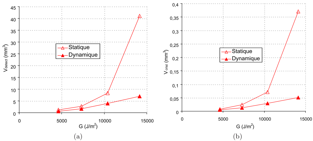
FIGURE 6.28 – Evolution des paramètres V_{detect} et V_{crist} mesurés en statique et en dynamique en fonction du taux de restitution d'énergie G dans le cas du mélange NR50.
