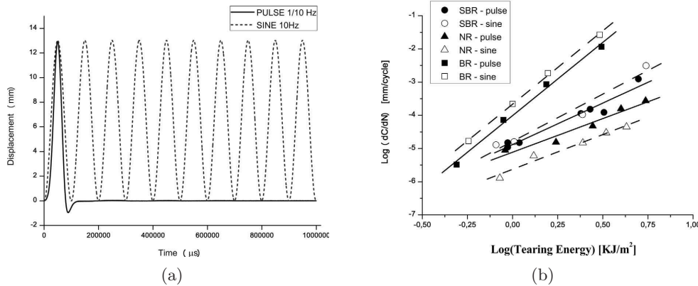
FIGURE 2.13 – Influence du type de signal sur la vitesse de propagation : (a) Signal sinusoïdal et signal impulsif, (b) Influence du type de signal sur la vitesse de propagation dans le cas de trois types d'élastomères chargés à 50 pce de noir de carbone (NR, BR et SBR), d'après Andreini et al. (2013).
