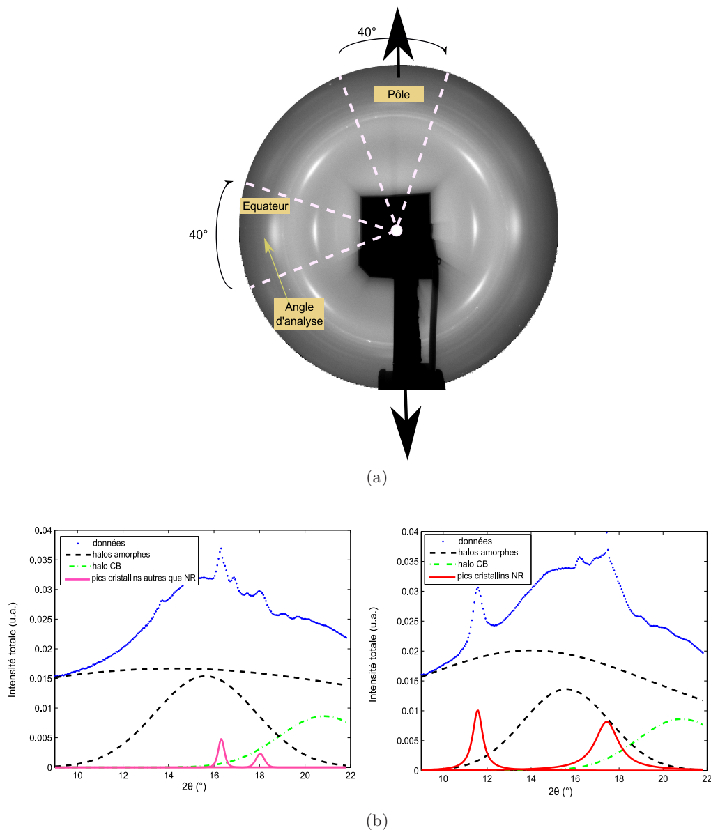
FIGURE 3.30 – Extraction du spectre d'intensité totale pour le calcul de l'index \chi . (a) Domaines d'extraction de l'intensité totale sur le cliché de diffraction, pour deux angles azimuthaux moyens différents (correspondant au pôle et à l'équateur). Les flèches indiquent la direction de traction. (b) Déconvolution du spectre d'intensité totale par des fonctions de Pearson VII au pôle (à gauche) et à l'équateur (à droite). On notera la présence de pics parasites (notés « autres » dans la légende), déconvolués seulement dans le cas du spectre de l'intensité extraite au pôle. Leur déconvolution dans le cas de la direction équatoriale entraînant une hausse importante du temps de calcul compte tenu du grand nombre de pics.
