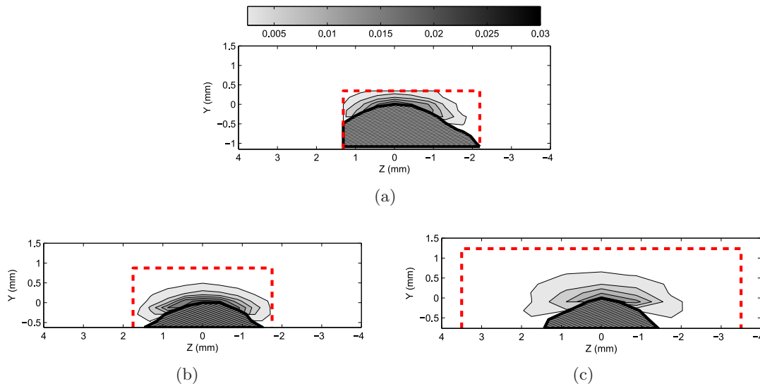
FIGURE 6.34 – Cartographies lissées des valeurs de \chi mesurées par WAXD en dynamique dans le cas des mélanges chargés, pour une même élongation maximale \lambda = 1,61 de sollicitation. (a) : NR30, G = 5230 \text{ J/m}^2 . (b) : NR50, G = 7290 \text{ J/m}^2 . (c) : NR70, G = 10230 \text{ J/m}^2 .
