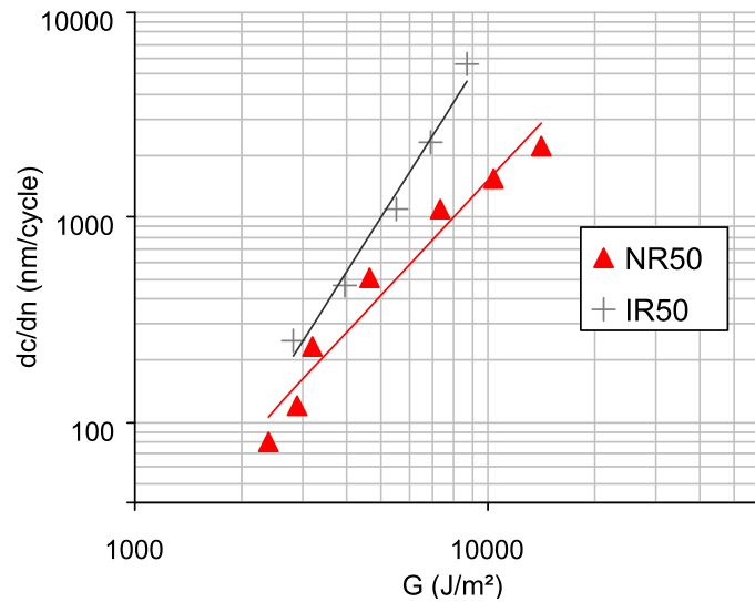
FIGURE 4.20 – Vitesses de propagation de fissure dc/dn en fonction de G à température ambiante pour les mélanges NR50 (naturel) et IR50 (synthétique). Les droites représentent les ajustements de lois puissances. Pentes des droites : NR50 ( \beta = 1,85 ), IR50 ( \beta = 2,73 ).
