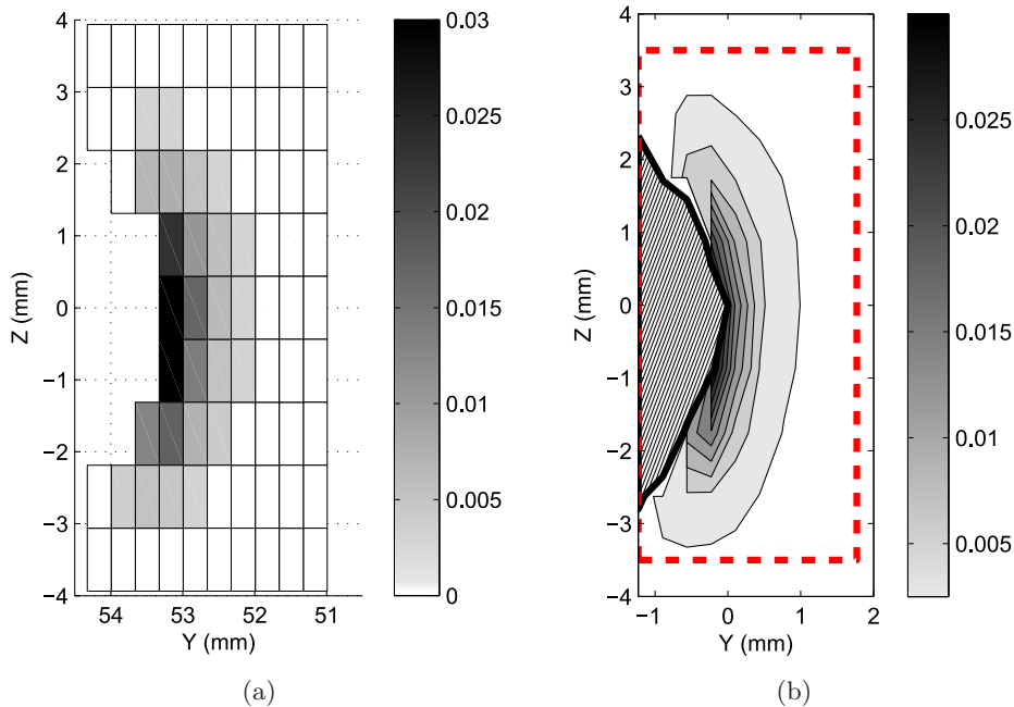
FIGURE 6.24 – Cartographie de mesures dynamiques d'index de cristallinité \chi en pointe de fissure de fatigue dans le cas d'une éprouvette de caoutchouc NR50 sollicitée à \lambda = 1,92 ( G = 14141 \text{ J/m}^2 ) : (a) cartographie de valeurs discrètes, (b) isovaleurs d'index de cristallinité correspondant aux valeurs discrètes de (a). La zone hachurée représente la fissure et le contour discontinu marque les dimensions de la zone de mesure. Les valeurs de \chi sont représentées par une échelle de niveaux de gris entre \chi_{min} = 0,0025 et \chi_{max} = 0,03 .
