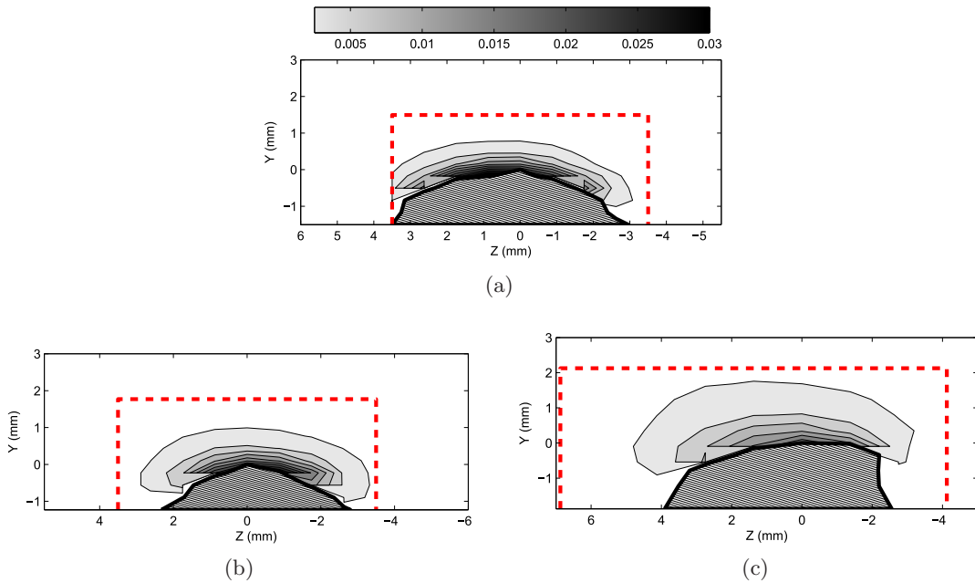
FIGURE 6.35 – Cartographies lissées des valeurs de \chi mesurées par WAXD en dynamique dans le cas des mélanges chargés, pour une même élancement maximale \lambda = 1,92 de sollicitation. (a) : NR30, G = 10200 \text{ J/m}^2 . (b) : NR50, G = 14140 \text{ J/m}^2 . (c) : NR70, G = 20392 \text{ J/m}^2 .
