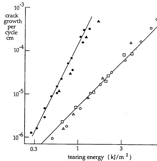
FIGURE 2.6 – Mesures des vitesses de propagation en fonction du taux de restitution d'énergie, d'après Lake (1995). Points noirs : SBR chargé au noir de carbone (50 pce), points blancs : NR chargé au noir de carbone (50 pce). Les différents symboles représentent les différentes géométries d'éprouvettes utilisées pour les mesures, confirmant l'indépendance de la relation dc/dn = f(G) à la géométrie de l'éprouvette.
