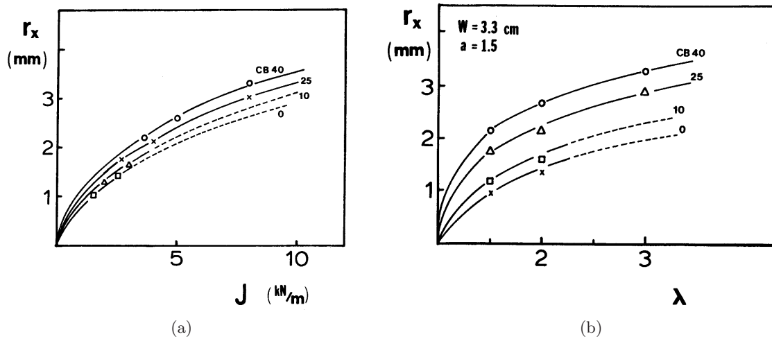
FIGURE 6.41 – Evolution du paramètre r_x , dimension de la zone cristallisée dans l'axe de la fissure, pour différents mélanges NR chargés au noir de carbone, en fonction (a) du taux de restitution d'énergie maximal J , et (b) de l'élongation globale maximale \lambda , d'après les résultats de Lee et Donovan (1987) .
