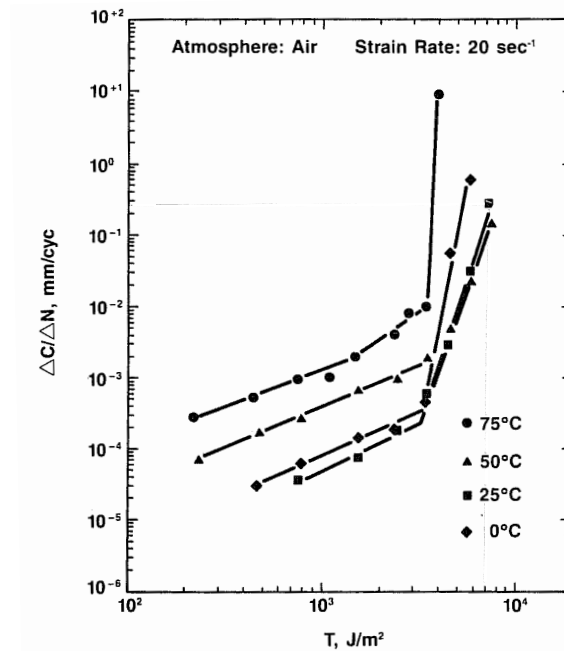
FIGURE 2.9 – Influence de la température sur la vitesse de propagation de fissure de fatigue d'un mélange NR chargé à 50 pce de noir de carbone, d'après Young (1986) .
