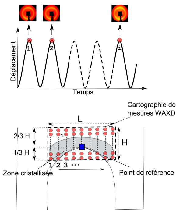
FIGURE 3.24 – Procédure d'acquisition des clichés de diffraction pendant l'essai de fatigue. En haut : les clichés de diffraction sont enregistrés au maximum de déplacement de chaque cycle. En bas : cartographie du voisinage de la pointe de fissure
