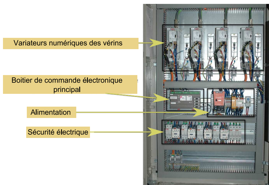
FIGURE 3.18 – Détails de l'organisation du tableau électrique de contrôle.
