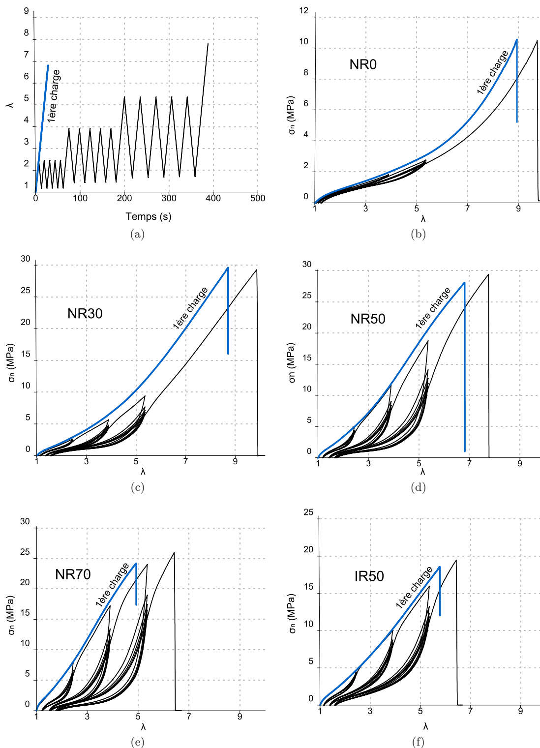
FIGURE 4.11 – Courbes de traction cyclique des différents mélanges à température ambiante. (a) Chemin de chargement, (b) NR0, (c) NR30, (d) NR50, (e) NR70, (f) IR50. Les échelles de l'axe des ordonnées peuvent varier d'un graphe à l'autre. La chute brutale de contrainte marque le point de rupture de l'éprouvette.
