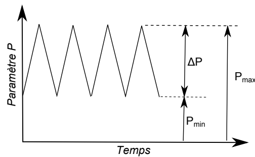
FIGURE 2.14 – Représentation schématique de la définition du rapport de chargement R = P_{min}/P_{max} .
