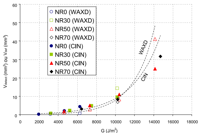
FIGURE 6.45 – Evolution des paramètres V_{detect} et V_{def}(\lambda_{1,lim} = \lambda_{d(0,25\%)}) mesurés en statique en pointe de fissure en fonction du taux de restitution d'énergie G pour les différents matériaux. Les courbes en traits pointillés représentent les ajustements sur les données expérimentales à partir d'une relation exponentielle.
