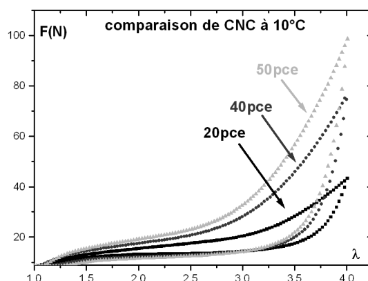
FIGURE 1.14 – Influence du taux de noir de carbone sur l’hystérèse mécanique du caoutchouc naturel, d’après Marchal (2006). Les matériaux ont subi préalablement un certain nombre de cycles à même élongation de manière à obtenir un cycle stabilisé (suppression de l’effet Mullins).
