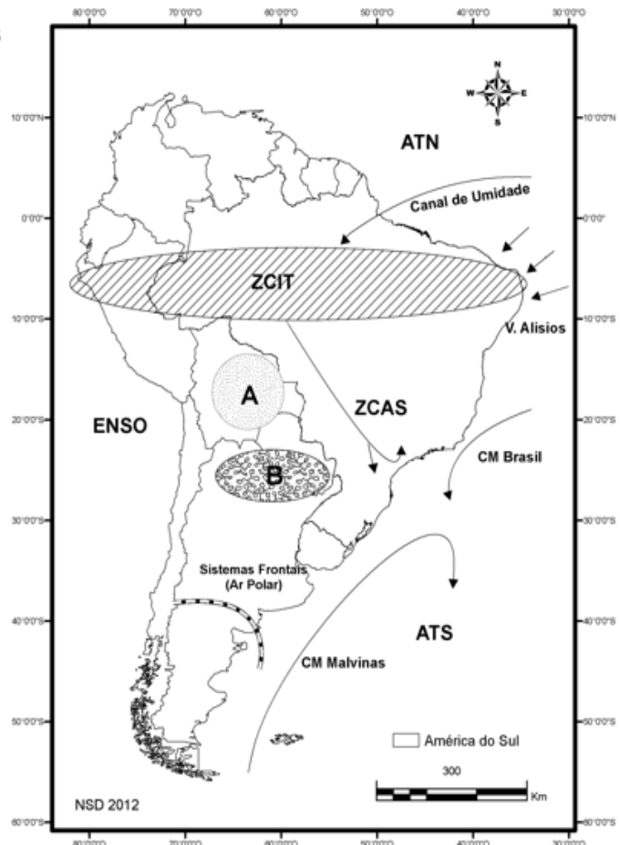
Figura 16 Representação dos principais fenômenos climáticos e de circulação atmosférica no verão austral da América do Sul. Fonte: Autor, 2012.
