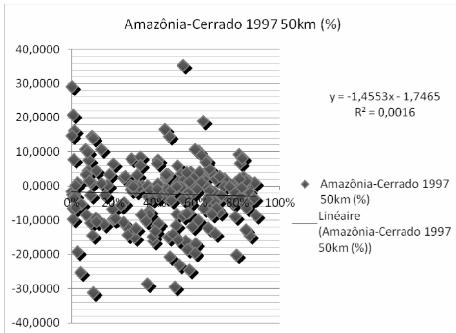
Gráfico 17 Série de gráficos representando as correlações entre pluviosidade e desmatamento para o conjunto das 207 estações no buffer de 50km. No eixo y a pluviosidade (mm) de acordo com a Análise de Regressão Linear, e no eixo x a % do total de floresta no período para o buffer.
