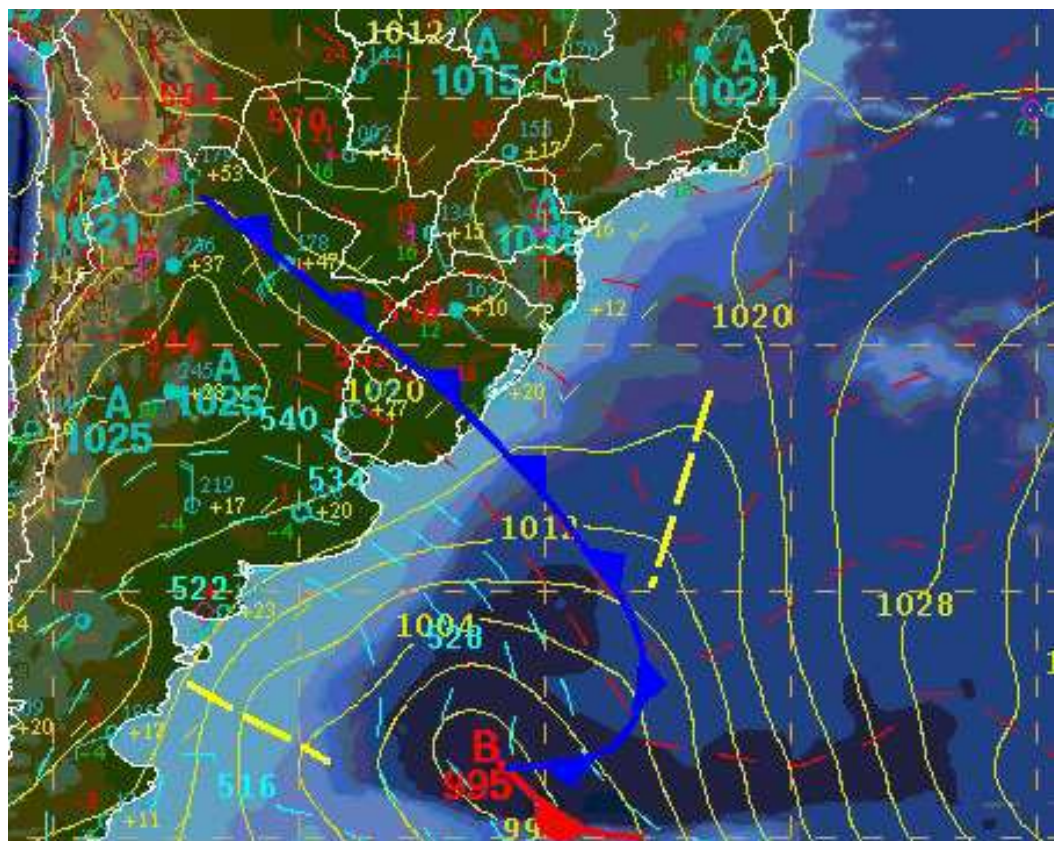
Figura 11 Na análise sinótica das 00Z do dia 01/07/2011 observa-se um sistema frontal com ramo frio que se estende do Noroeste da Argentina ao extremo sul do RS e Atlântico. Fonte: CPETEC, INPE, 2012.
