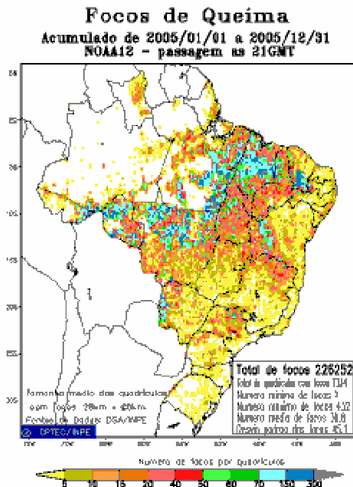
Figura 18 Focos de Queima no Brasil no ano de 2005. O ano de 2005 juntamente com os anos de 2004 e 2010 estão entre os mais importantes em relação as queimadas. Fonte: CPETEC, INPE, 2012.
