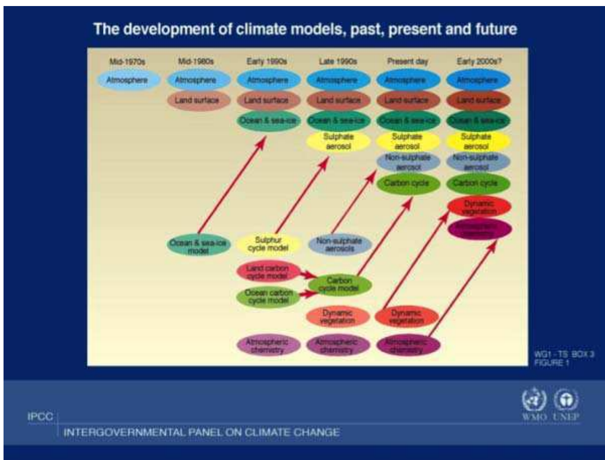
Figura 5 A figura mostra o desenvolvimento dos modelos climáticos a partir da década de 1970. Fonte: IPCC (2012) e WMO (2012).
