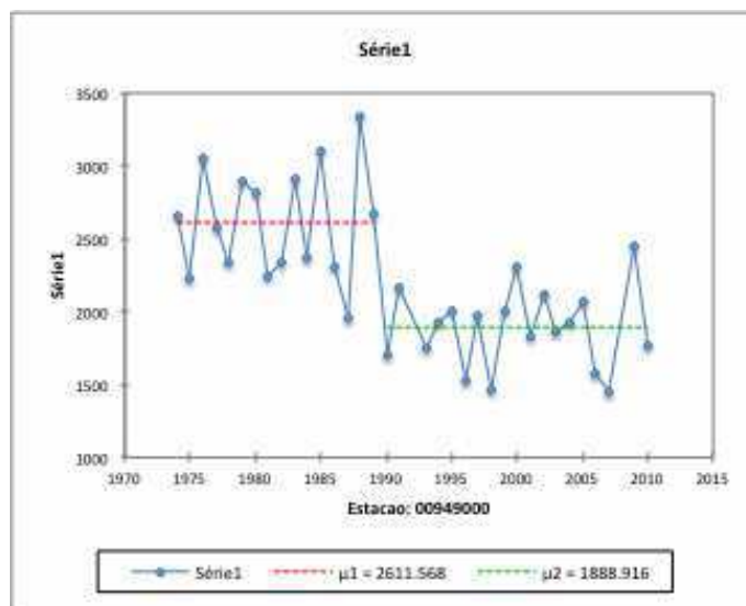
Gráfico 4 Aqui é ilustrado um exemplo de gráfico gerado por meio da utilização da análise estatística do Teste de Pettitt. Neste gráfico do município de Alta Floresta (MT) vemos uma ruptura na série histórica entre os anos de 1990 e 1991. O gráfico mostra um decréscimo substancial de 2,611 mm para 1,888 mm das médias anuais das chuvas na região.
