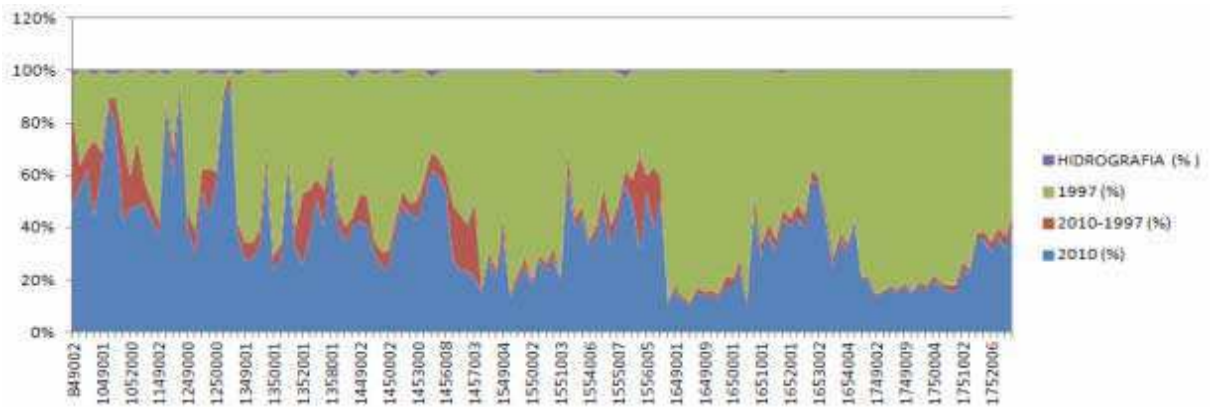
Gráfico 15 Série de Gráficos 2 - porcentagem do total das áreas e sua classificação com divisão por Biomas. A esquerda do gráfico o total da área em porcentagem. No eixo x as estações com latitude crescente da esquerda para direita. E na legenda a classificação das áreas ilustradas nos gráficos.
