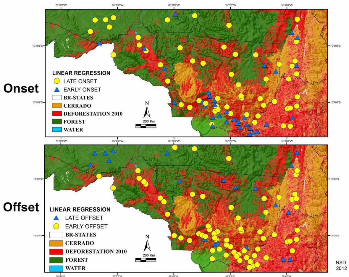
Mapa 15 Mapa ilustrando as estações pluviométricas conforme a Análise de Regressão Linear (ARL) para o IPC e FPC no período de (1971-2010). Na mapa superior o IPC e no inferior o FPC. Círculos em amarelo representam tendências negativas. Triângulos azuis representam tendências positivas.
