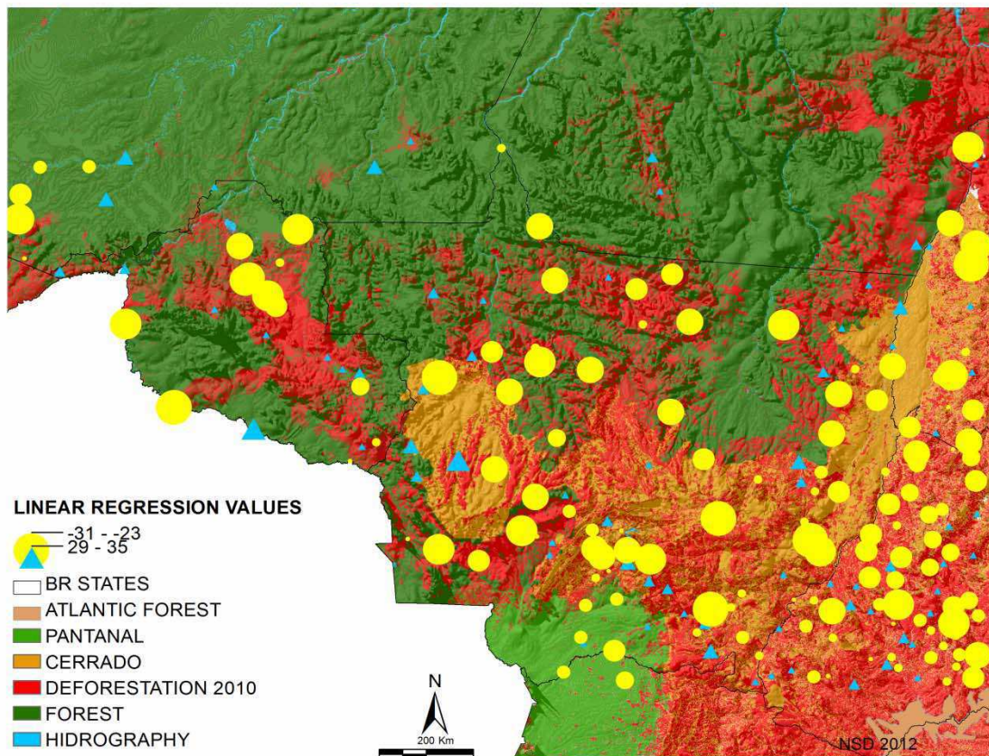
Mapa 9 Análise de regressão linear das 207 estações y = (ax+b) . A escala da legenda separa os valores entre os limites de -38 mm até 38 mm de ganho e perda. Em azul tendências positivas e em amarelo tendências negativas de precipitação. Fonte: Autor, 2012
