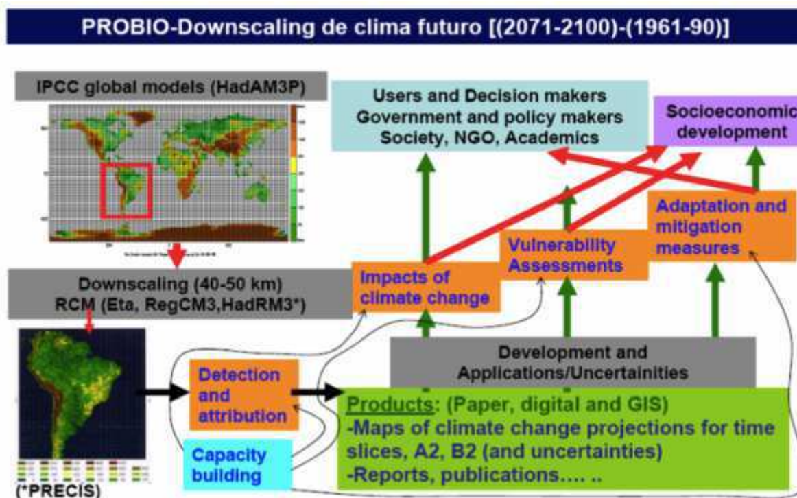
Figura 6 Programa Brasileiro PROBIO de downscaling do clima futuro com previsões até 2100. Na figura o Esquema operacional dos modelos globais e de regionalização “downscaling”, usando os modelos do IPCC e os modelos regionais Eta, RegCM3 e HadRM3 e suas implicações nas políticas públicas de vulnerabilidade, adaptação e mitigação às mudanças climáticas. Fonte: Marengo et al. (2007).
