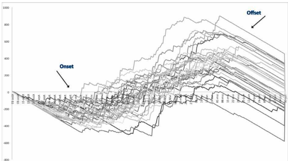
Gráfico 11 Exemplo de aplicação da metodologia para a estação de código 0074900 (ANA). No eixo x os meses do ano com as linhas respectivas para cada um dos 40 anos de dados. No eixo y os valores de pontuação acumulada mínima e máxima. Fonte: Autor, 2012.
