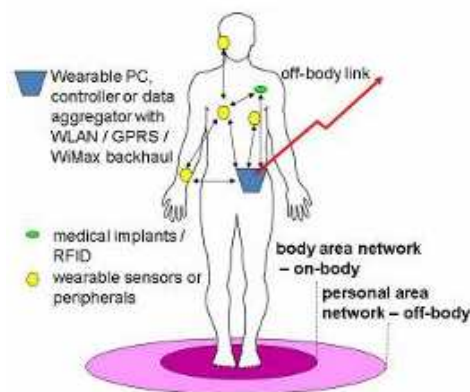
Figure II.5: Représentation d'un WBAN (IEEE-802.11.6 [32])
