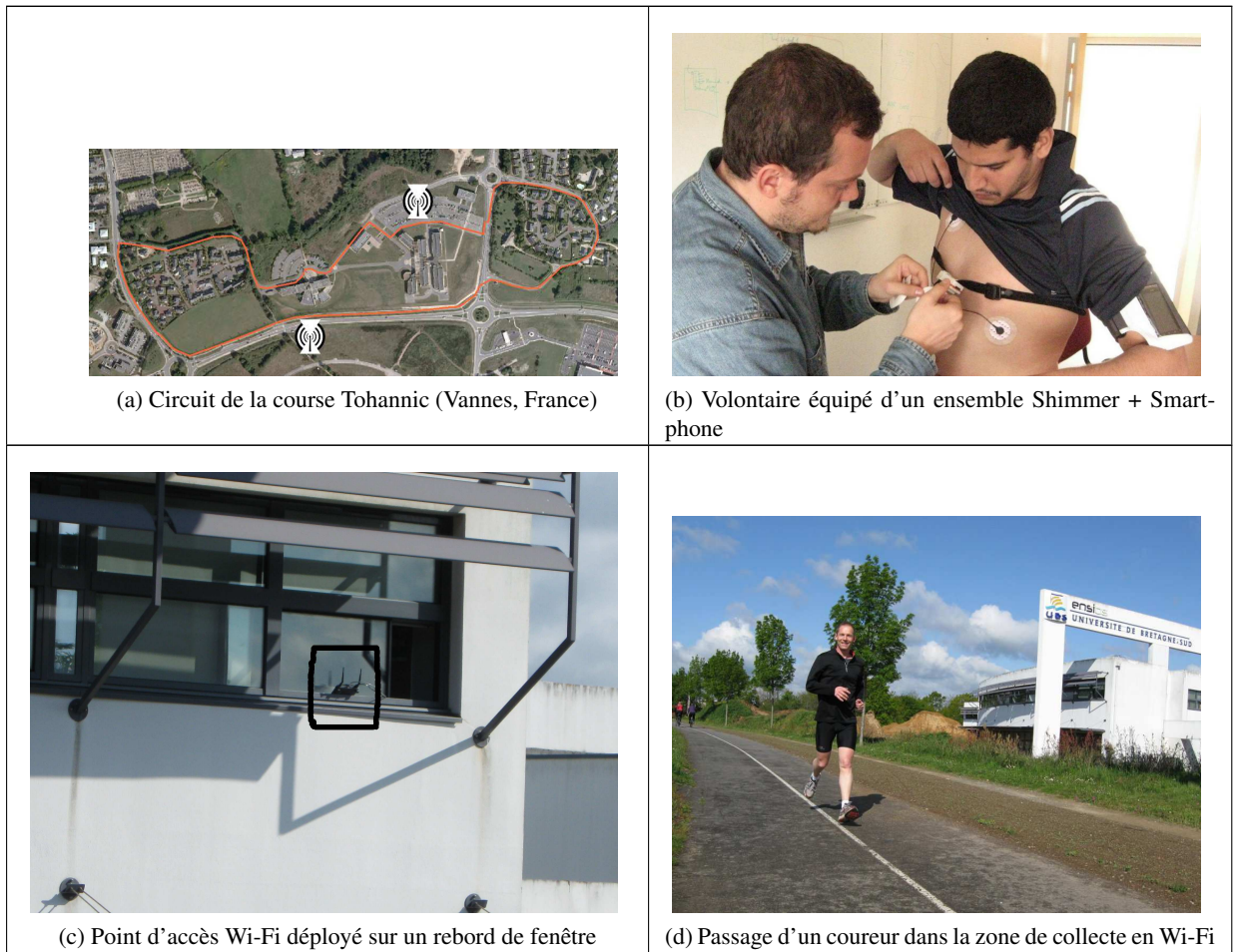
Figure V.10 : Expérimentation de la solution option Wi-Fi
