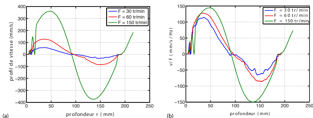
FIGURE IV.15 – Profil UDV sondant la vitesse radiale dans le plan médian pour plusieurs vitesses de rotation des disques. (b) Profil UDV normalisés par la fréquence de rotation des disques.
