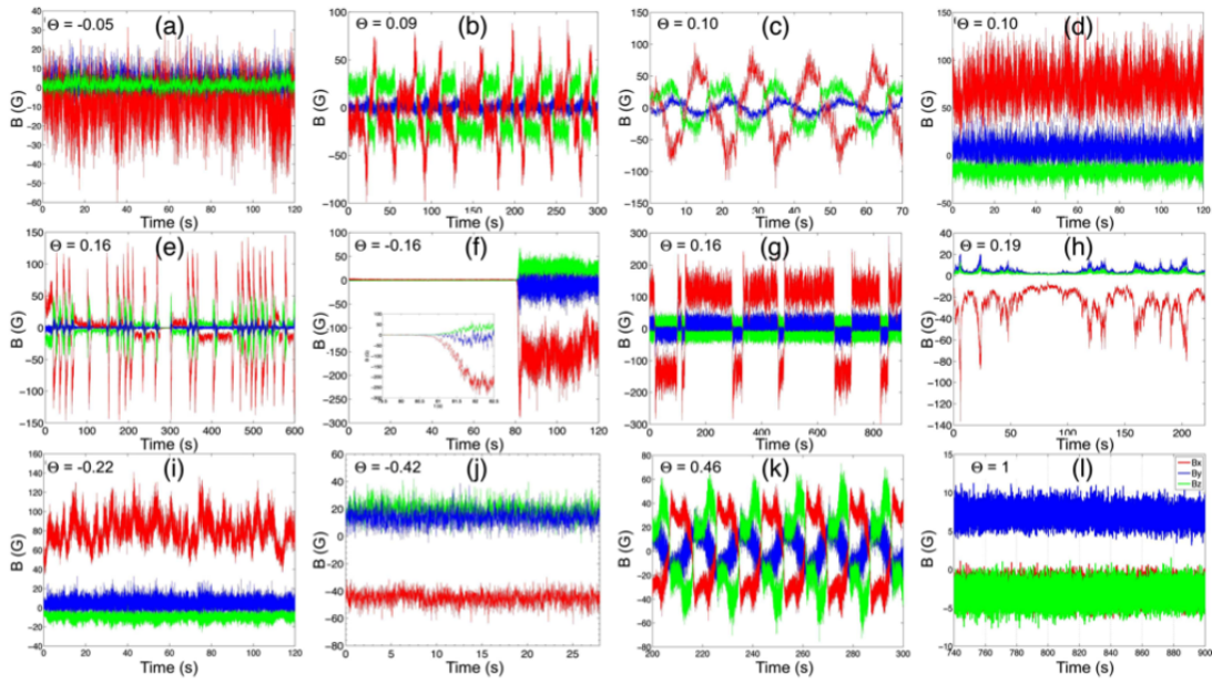
FIGURE I.23 – (a) Exemple de régimes dynamiques observée lors de la campagne VKS 2G en forçage asymétrique. ([54])
