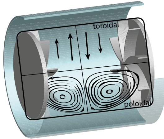
FIGURE I.20 – Écoulement s_2t_2 de Dudley James en géométrie cylindrique.
