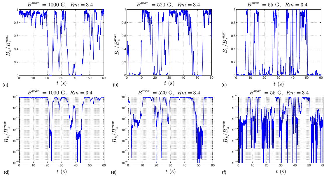
FIGURE III.9 – En haut (a, b, c) : Champ dynamo à (Rm - Rm_c) / Rm_c = 0.17 pour différentes valeurs de B_{max} . (a) B_{max} = 1000 G. (b) B_{max} = 500 G. (c) B_{max} = 60 G. En bas (c, d, e) : idem en échelle log
