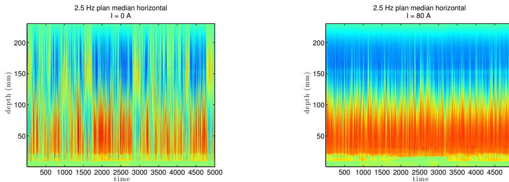
FIGURE IV.16 – (a) Diagramme spatiotemporel de vitesse radiale sans champ appliqué. (b) Diagramme spatiotemporel de vitesse radiale dans la direction du champ appliqué transverse B = 1000 G.
