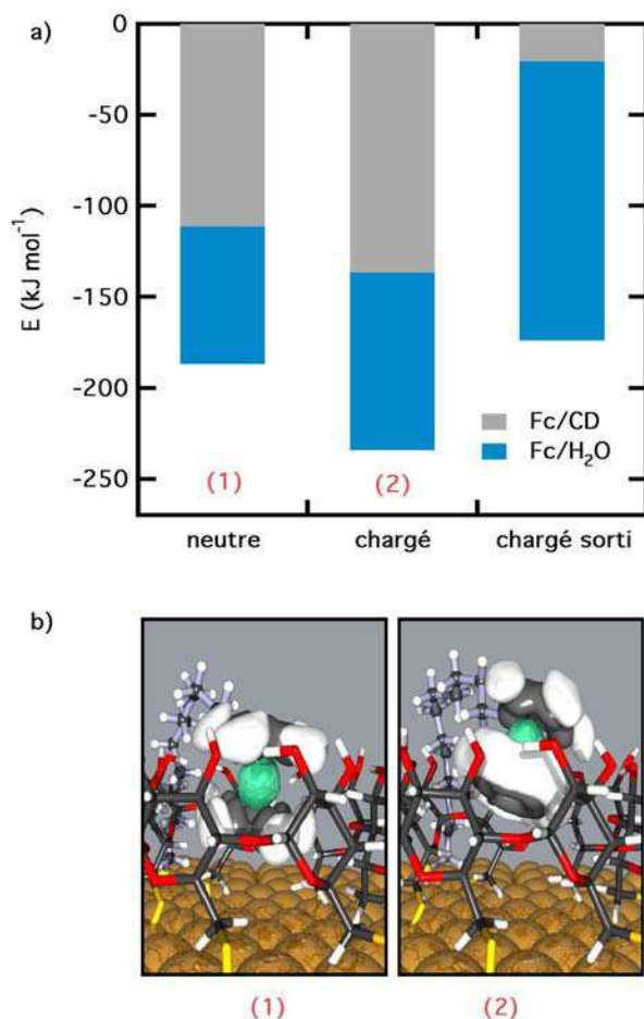
Figure 4.6 – a) Somme des interactions Lennard-Jones et électrostatiques des contributions FcC_nS/\beta -CD et FcC_nS/H_2O pour la monocouche \beta -CDS-/FcC 12 S-/C 5 S-Au (1) avant et (2) après oxydation. Pour comparaison, les mêmes contributions énergétiques ont été déterminées pour un système dans lequel la tête Fc^+ a été initialement placée en dehors de la \beta -CD. b) Fonctions de distribution spatiales de la tête ferrocène (1) à l'état neutre et (2) à l'état oxydé.
