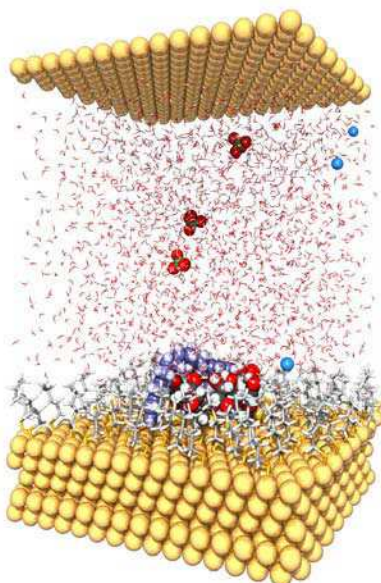
Figure A.13 – Cellule de simulation du système \beta -CDS-/ \text{FcC}_{13}\text{S} -/ \text{C}_5\text{S} -Au.
