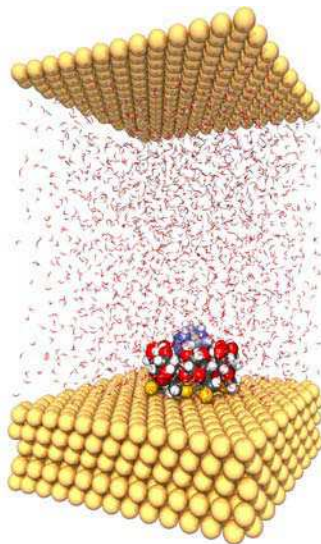
Figure A.10 – Cellule de simulation contenant le complexe d'inclusion formé entre la \beta -cyclodextrine greffée et le ferrocèneméthanol en phase aqueuse.
