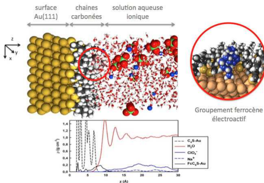
Figure A.1 – Cellule de simulation du système FcC 6 S-/C 4 S-Au et profil de masse volumique des espèces constituant le système selon l'axe z .
