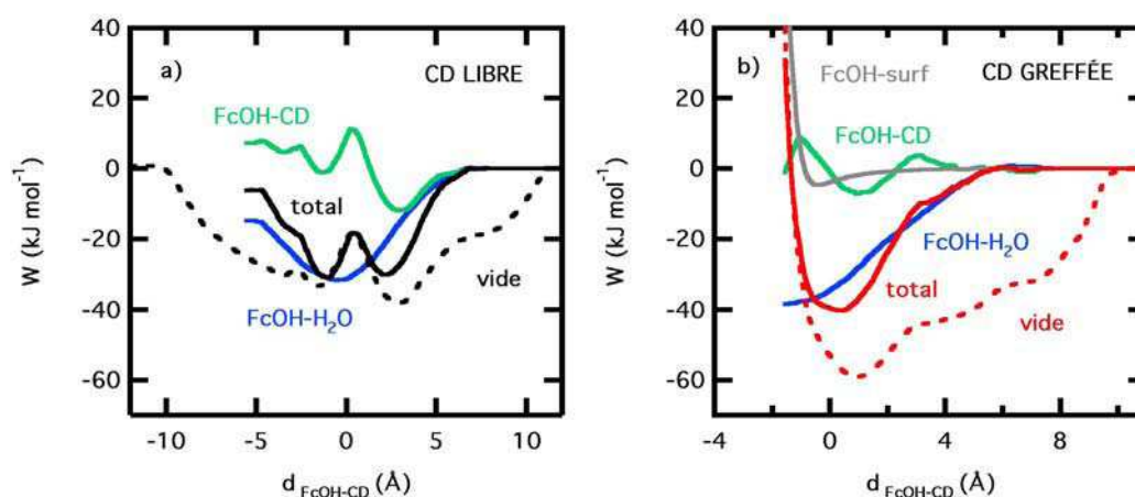
Figure 3.9 – Décomposition des profils de PMF en contributions FcOH-CD, FcOH-H 2 O et FcOH-surface a) pour l'association entre le FcOH et la \beta -CD libre dans le vide (pointillés) et en phase aqueuse (traits pleins) et b) pour l'association entre le FcOH et la \beta -CD greffée dans le vide (pointillés) et en phase aqueuse (traits pleins).
