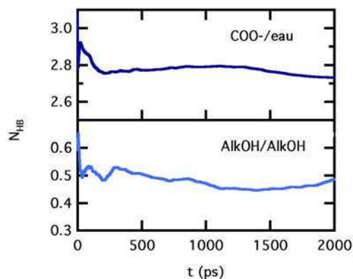
Figure A.6 – Moyenne cumulée du nombre de liaisons hydrogène par groupement en fonction du temps entre les groupements hydroxyles des chaînes et entre les groupements carboxylates et l'eau.
