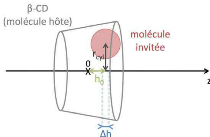
Figure 1.12 – Schéma représentant le volume accessible à la molécule invitée pour former un complexe avec la \beta -CD.
