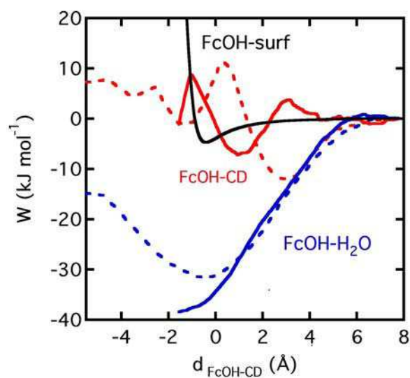
Figure 3.5 – Décomposition du profil de PMF en contributions FcOH-CD, FcOH- \text{H}_2\text{O} et FcOH-surface en milieu homogène (courbes en pointillés) et en milieu hétérogène (courbe en traits pleins).
