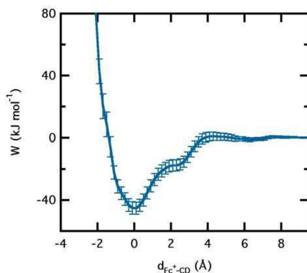
Figure 4.7 – Potentiel de force moyenne entre l'ion ferrocénium et la \beta -CD greffée dans une solution aqueuse de \text{NaClO}_4 0.1 \text{mol}\cdot\text{L}^{-1} .
