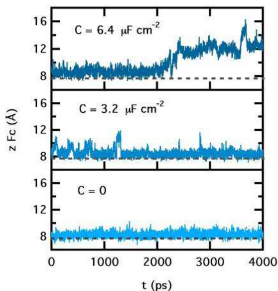
Figure 4.10 – Coordonnées du centre de masse de l'ion ferrocénium selon l'axe z en fonction du temps de simulation pour une capacité surfacique nulle, de 3.2 \mu\text{F}\cdot\text{cm}^{-2} et de 6.4 \mu\text{F}\cdot\text{cm}^{-2} .
