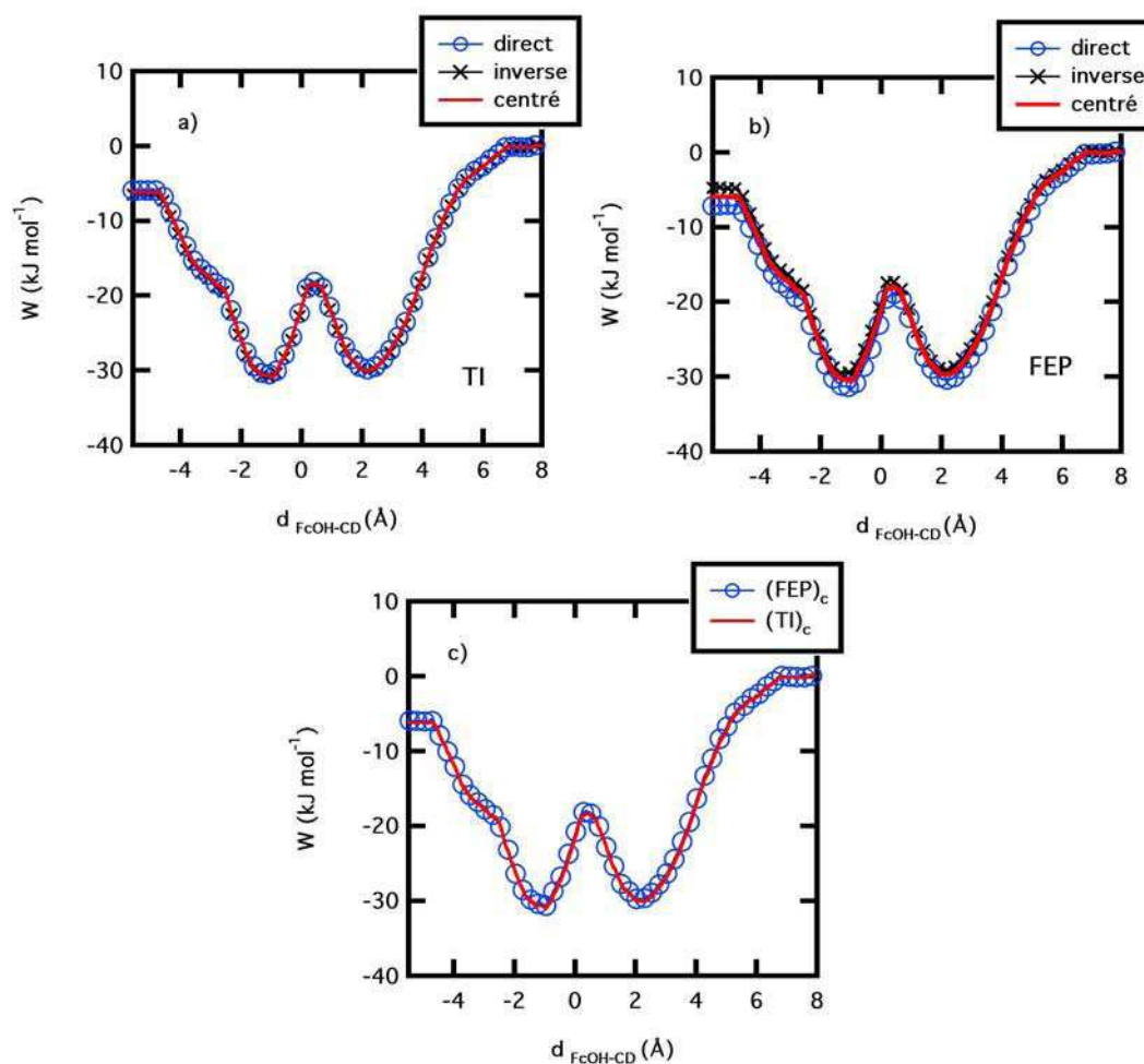
Figure 1.14 – Potentiel de force moyenne en fonction de la distance de séparation entre les centres de masse du ferrocène-méthanol et de la \beta -CD libre en phase aqueuse obtenu a) avec la méthode TI et b) avec la méthode FEP dans les sens direct et inverse. La valeur centrée est également donnée. Le graphique c) compare les valeurs centrées des deux méthodes.
