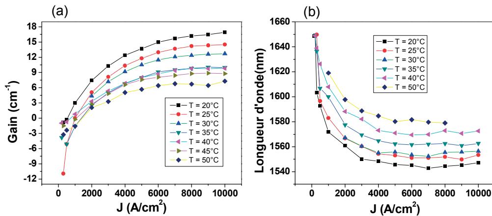
Figure 5-16 : (a) maximum du gain des SOA à BQs en fonction de la densité de courant, (b) Longueur d'onde du pic du gain
