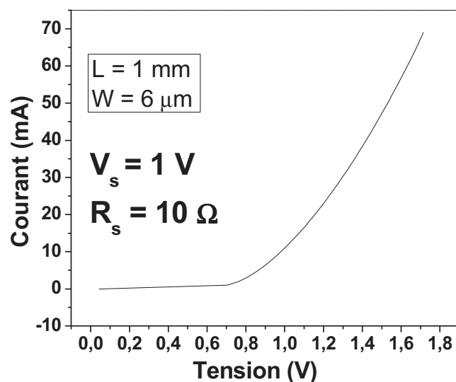
Figure 3-15 : I(V) du laser à PQs fabriqué avec le procédé P1 de longueur de cavité 1 mm et de largeur du ruban de 6 µm.
