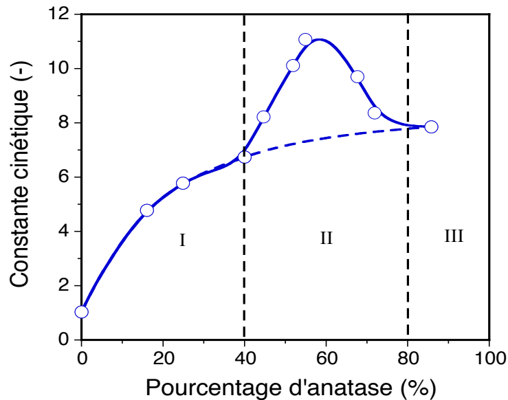
Figure 1.8. Evolution qualitative de l'activité photocatalytique de films minces de TiO 2 en fonction du pourcentage d'anatase dans la dégradation du bleu de méthylène à température ambiante. Image adaptée de la référence [91].
