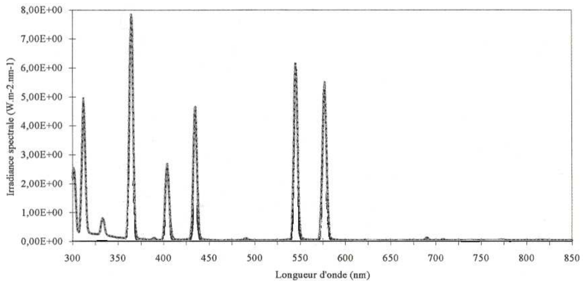
Figure II.9. Spectre d'irradiation de la lampe HPK 125W (Données fournisseur)
