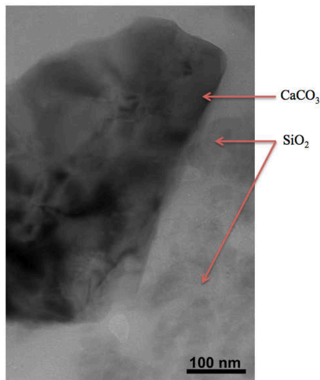
Figure III.1.a. Cliché MET d'une particule de \text{CaCO}_3 et des particule de silice générées par nucléation primaire homogène.
