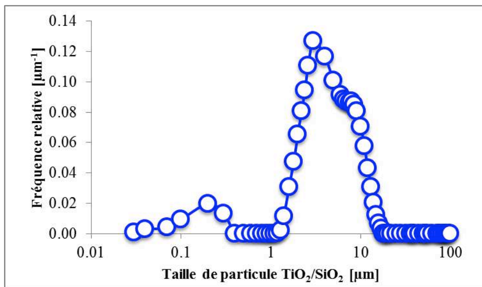
Figure III.16. Distribution de la taille des agrégats TiO 2 /SiO 2 avant incorporation dans le papier.
