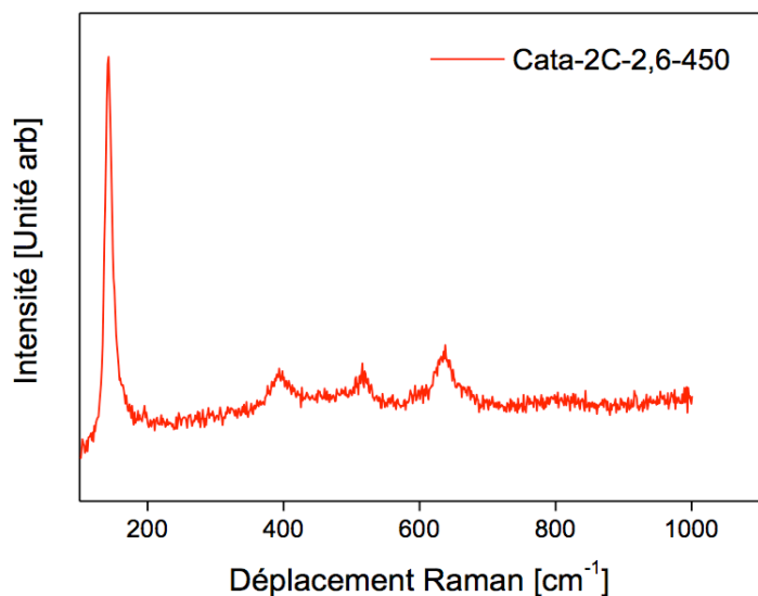
Figure III.8. Spectre Raman des échantillons Cata-2C-2,6-450 après traitement thermique à 450°C pendant 4 h.
