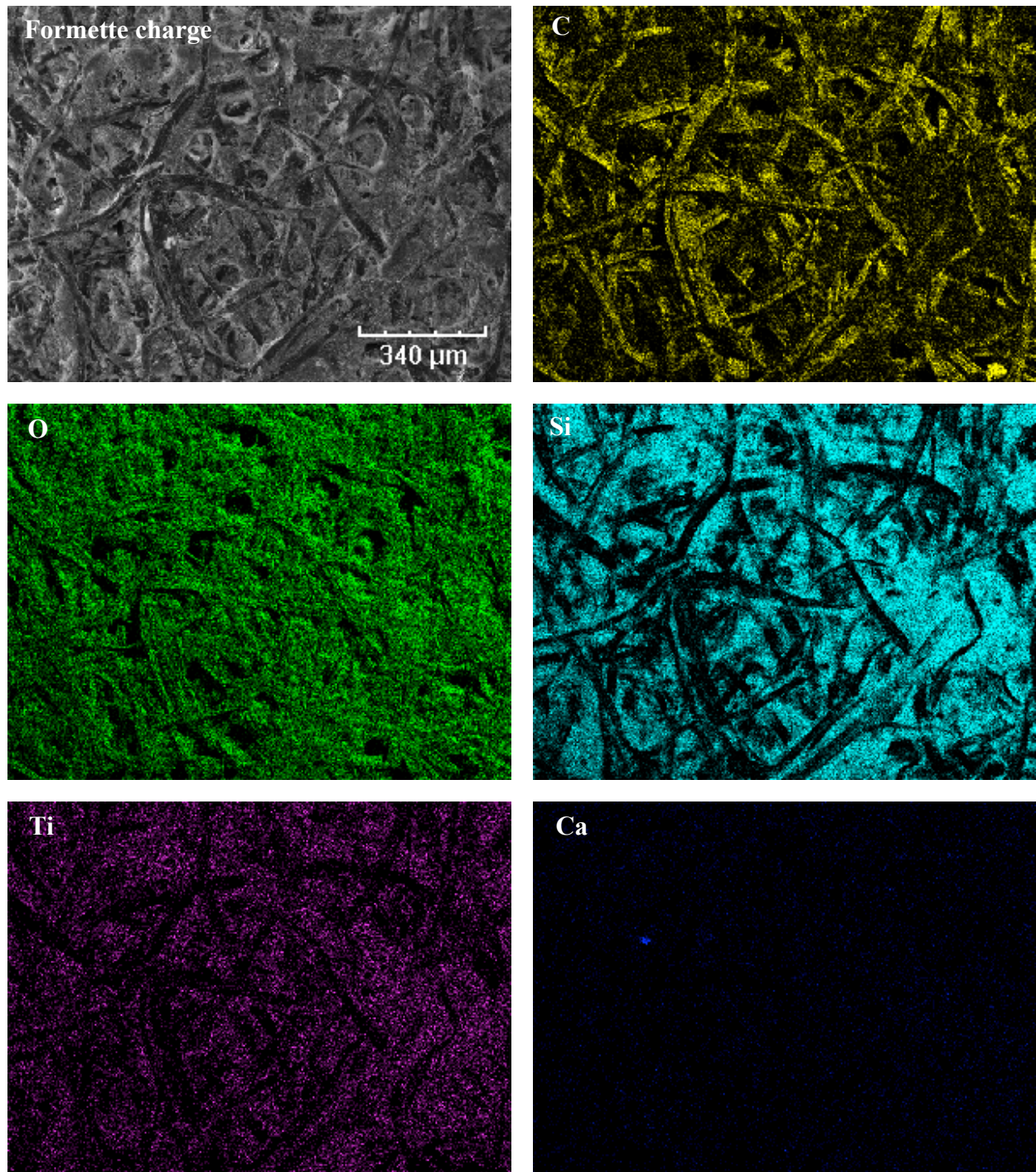
Figure III.21. Cartographie des éléments dans la formette à grammage 200 g/m 2 obtenue par microanalyse EDX.
