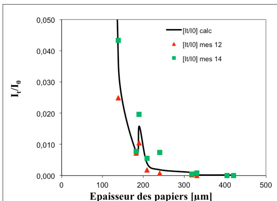
Figure V.3. Variation de I_t/I_L calculé et mesurés en fonction des épaisseurs des papiers
