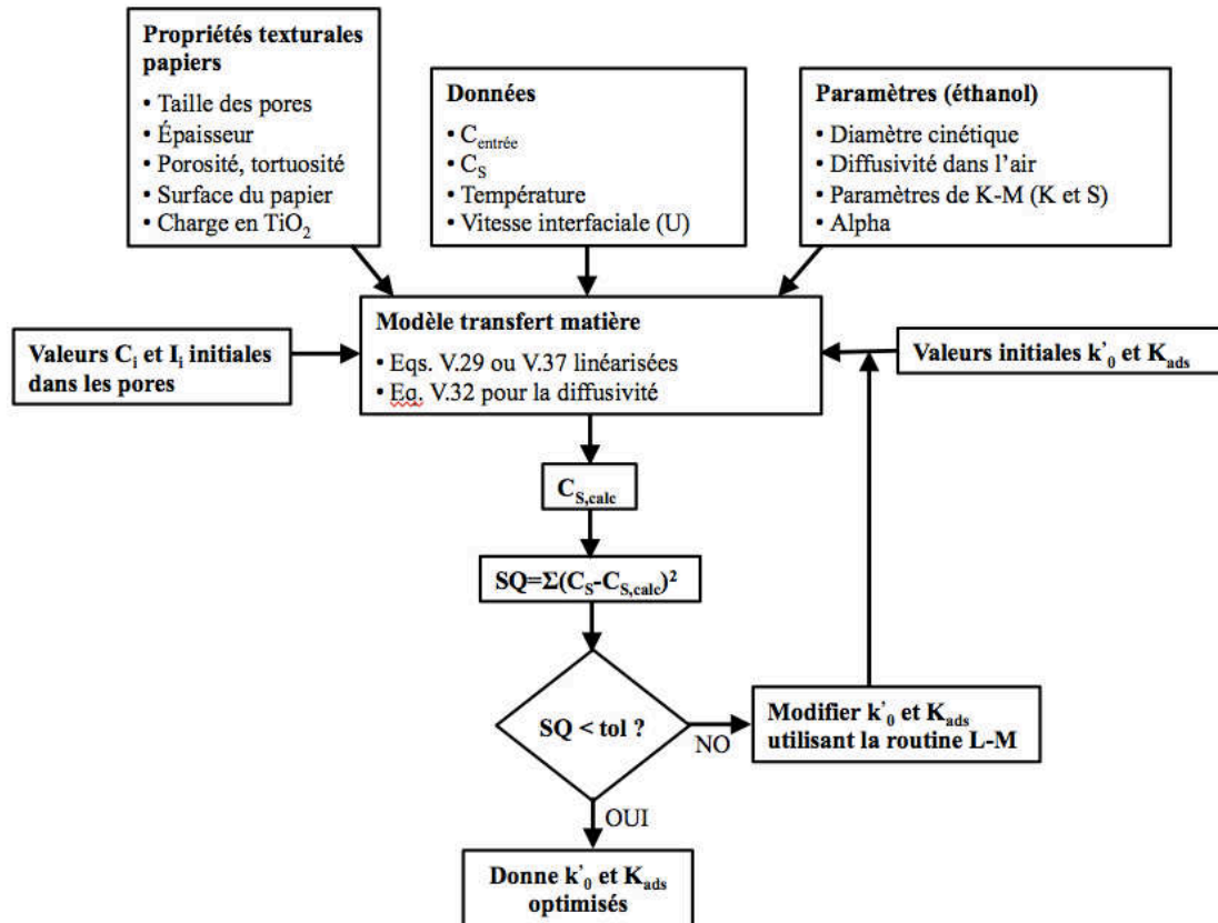
Figure V.9. Algorithme du calcul pour obtenir les valeurs de k'_0 et K_{ads} du \text{TiO}_2 dans les papiers photocatalytiques à partir des données expérimentales.
