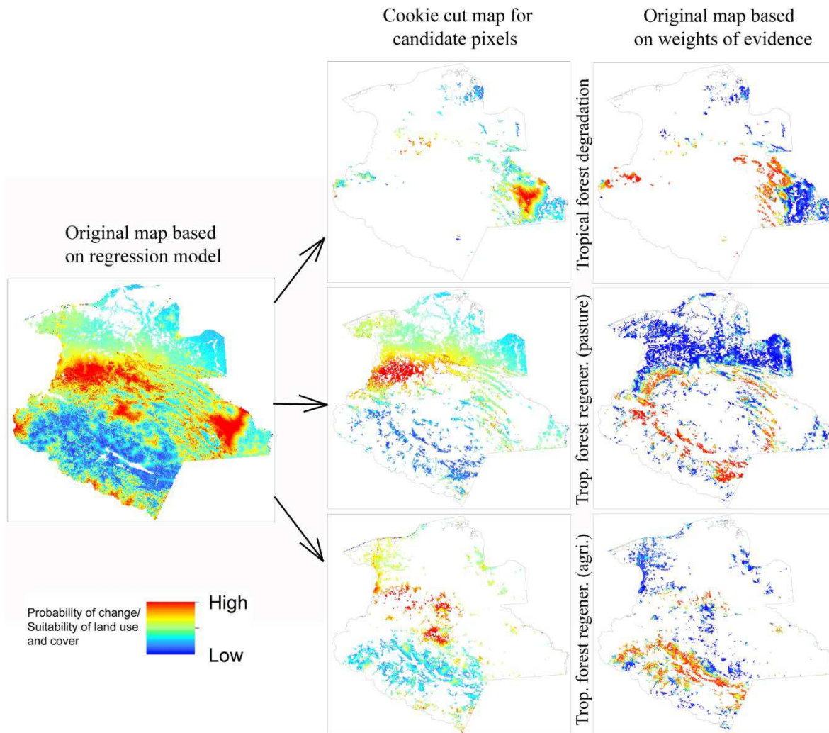
Figure 9. Les cartes de changement potentiel générées par les 12 plus importants facteurs pour l'usage des terres et le changement de couverture 1993-2002. En utilisant les modèles de régression, une seule carte décrivant la pertinence de la forêt tropicale secondaire est générée et qui peut être réduite pour les pixels susceptibles d'être choisis pour participer à une certaine transition tandis que le poids d'une approche évidente fournit des cartes spécifiques pour chaque transition.
