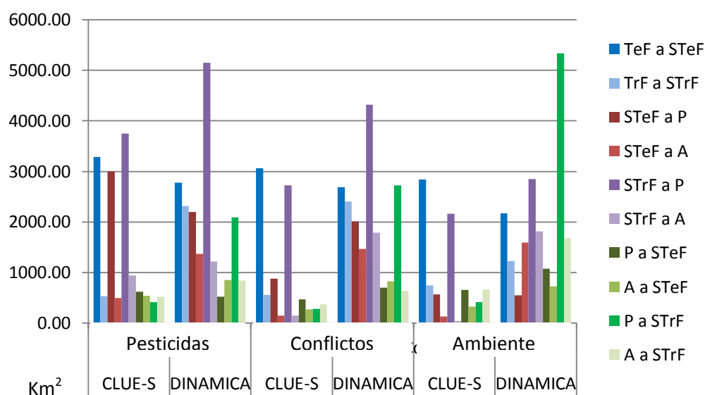
Figura 7. Áreas de cambio simuladas con CLUE y DINAMICA para cada escenario (TeF: bosque, STeF: bosque secundario, TrF: selva, STeF: selva secundaria, P: pastizal, A: agricultura).
