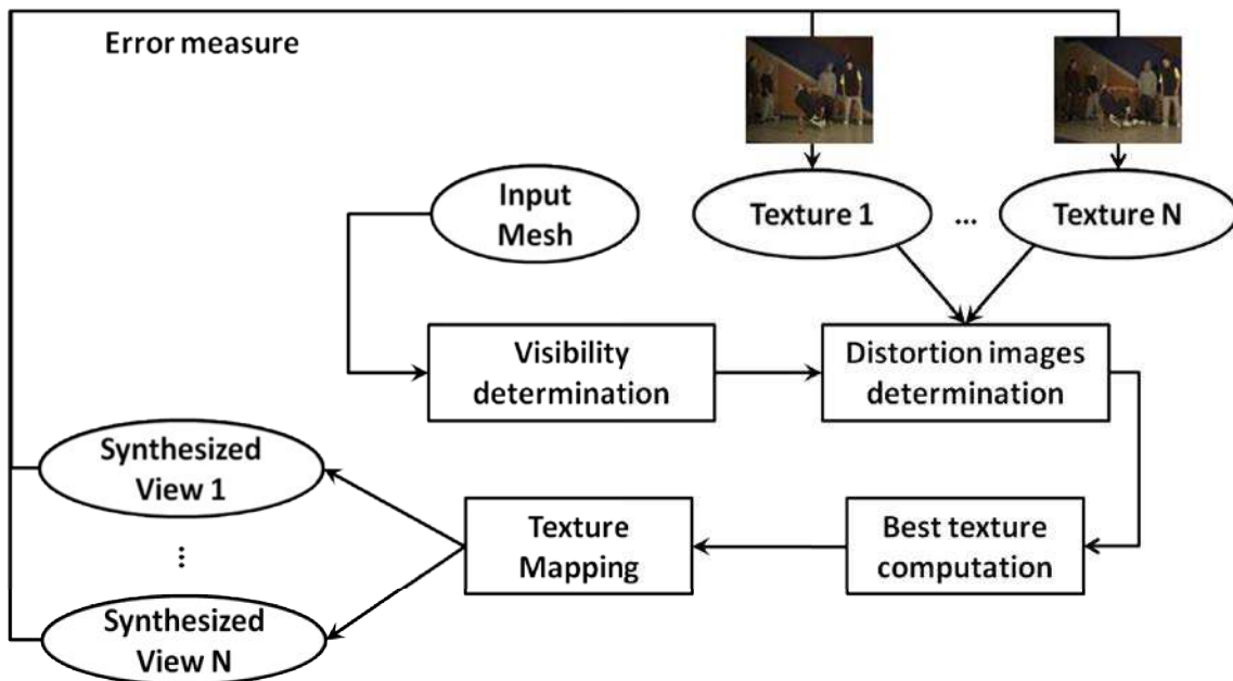
Figure 1.7: Le schéma global de la méthode de texturation proposée.
