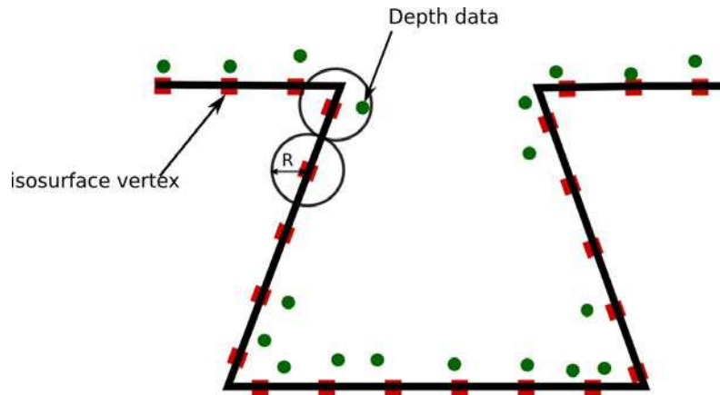
Figure 1.5: Post-traitement du maillage fusionné (rouge). Un sommet du maillage fusionné est ramené à la position du sommet le plus de l'ensemble des maillages d'entrée (vert) si la distance entre les deux points est inférieure à R .
