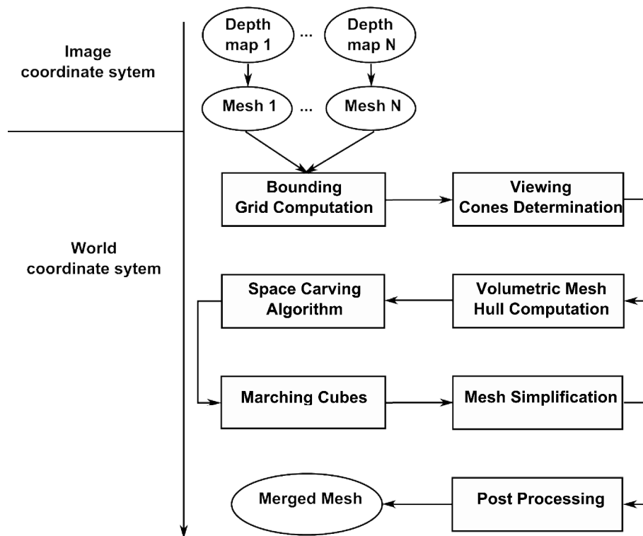
Figure 1.1: Le Schéma proposé de fusion de cartes de profondeur en un maillage triangulaire.
