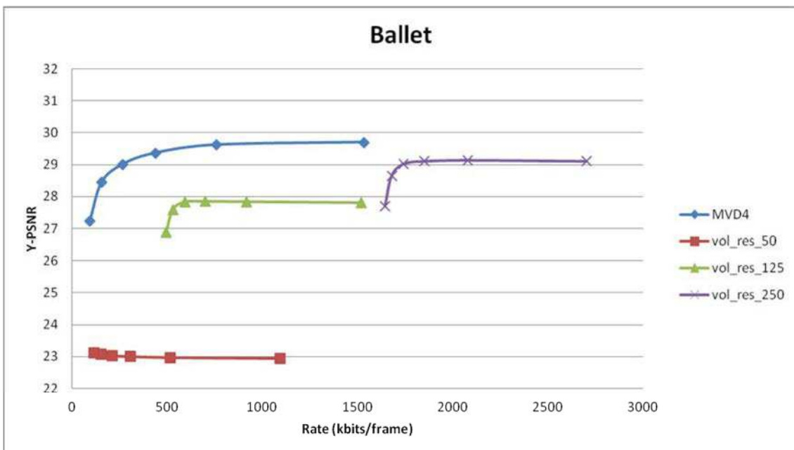
Figure 1.18: Courbes débit/distorsion pour différentes résolutions volumétriques (50, 125 et 250) vs. le modèle de référence pour la séquence ballet.
