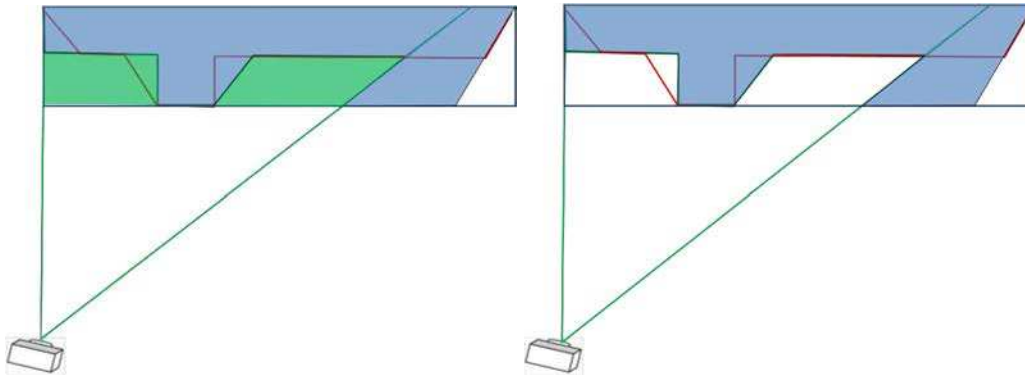
Figure 1.3: Space carving vis-à-vis de la caméra gauche. Les rayons sont tracés du centre de la caméra à l'EVM correspondante. Les zones vertes sont carvées (schéma à gauche). Le résultat du Space Carving vis-à-vis de la caméra gauche est montré dans le schéma à droite.
