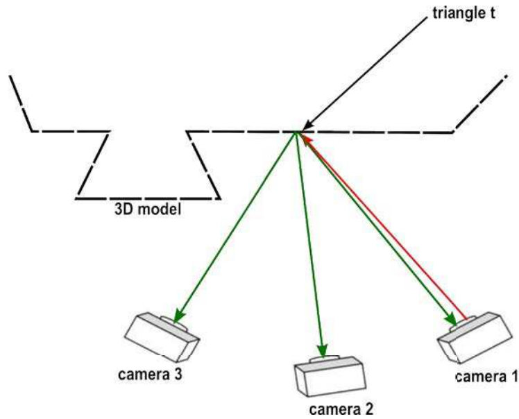
Figure 1.6: Détermination de la meilleure texture en utilisant la métrique de photo-cohérence. Flèche rouge désigne l'opération de plaquage de texture et la flèche verte désigne l'opération de projection.
