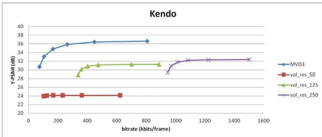
Figure 1.20: Courbes débit/distorsion pour différentes résolution volumétriques (50, 125 et 250) vs. le modèle de référence pour la séquence kendo.
