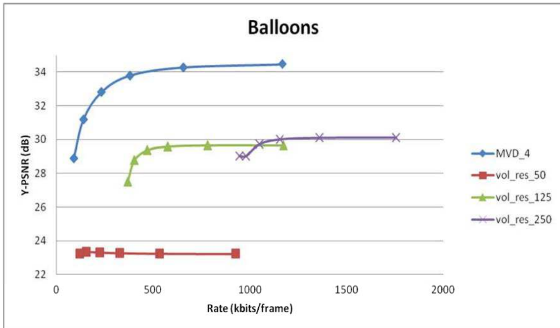
Figure 1.19: Courbes débit/distorsion pour différentes résolution volumétriques (50, 125 et 250) vs. le modèle de référence pour la séquence balloons.
