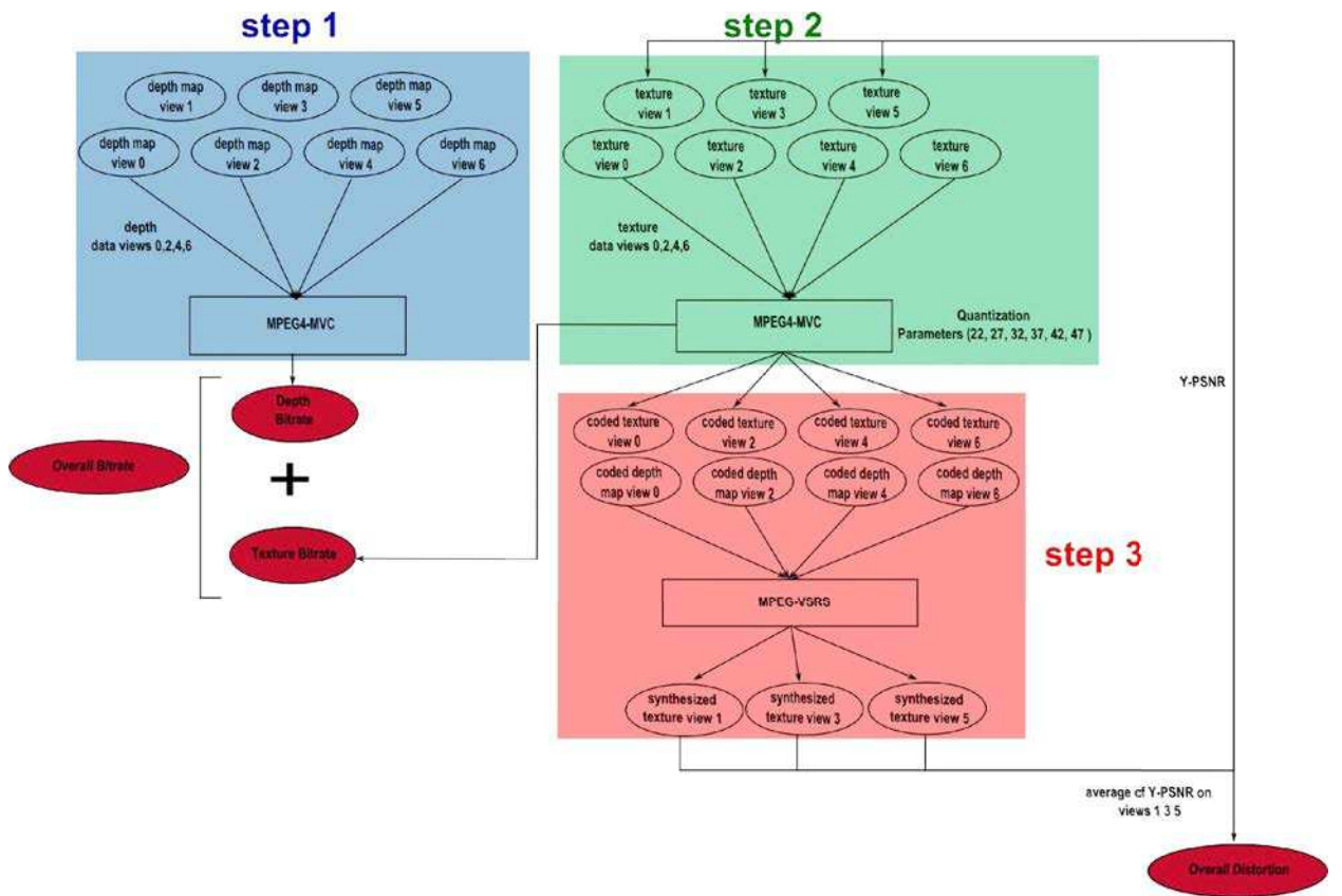
Figure 1.15: Évaluation du modèle de référence pour les séquences Microsoft ballet et breakdancers.
