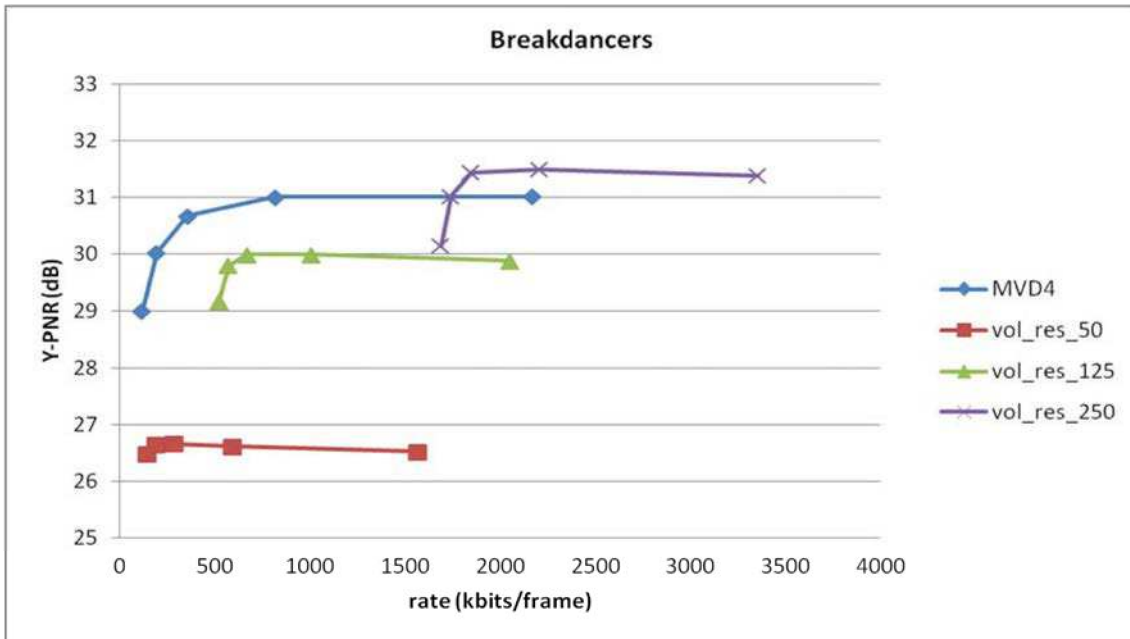
Figure 1.17: Courbes débit/distorsion pour différentes résolutions volumétriques (50, 125 et 250) vs. le modèle de référence pour la séquence breakdancers.
